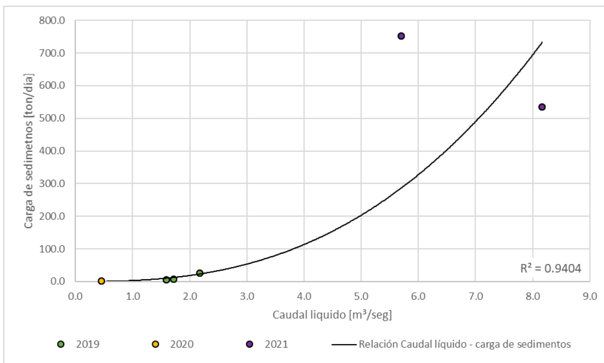
Figura 209. Relación caudal líquido - caudal sólido, Río Chinchiná - Cenicafé
