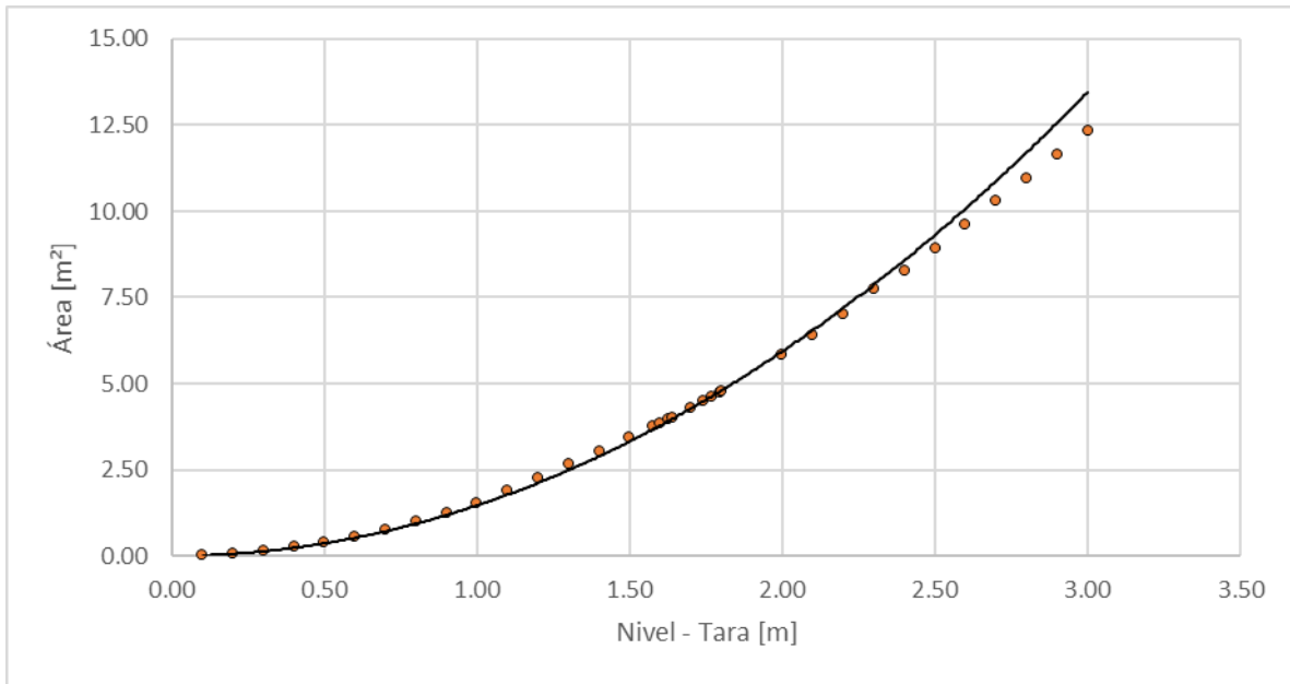
Figura 142. Nivel vs área, Río Guacaica – CHEC
