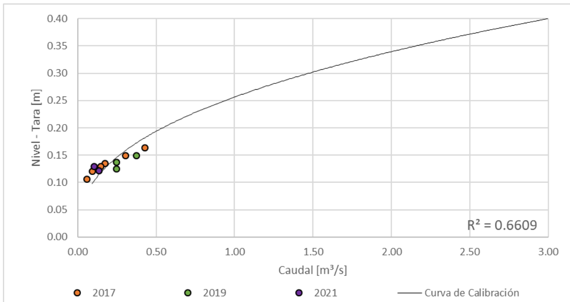
Figura 65. Curva nivel vs caudal, Quebrada Manizales – Skinco
