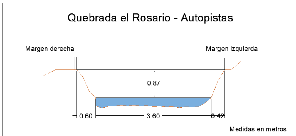
Figura 34. Sección transversal, Quebrada El Rosario - Autopistas, con medidas hechas en un cierto momento
