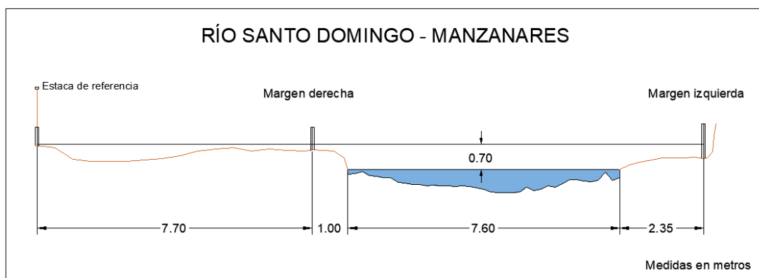
Figura 179. Sección transversal, Río Santo Domingo – Manzanares, con medidas hechas en un cierto momento
