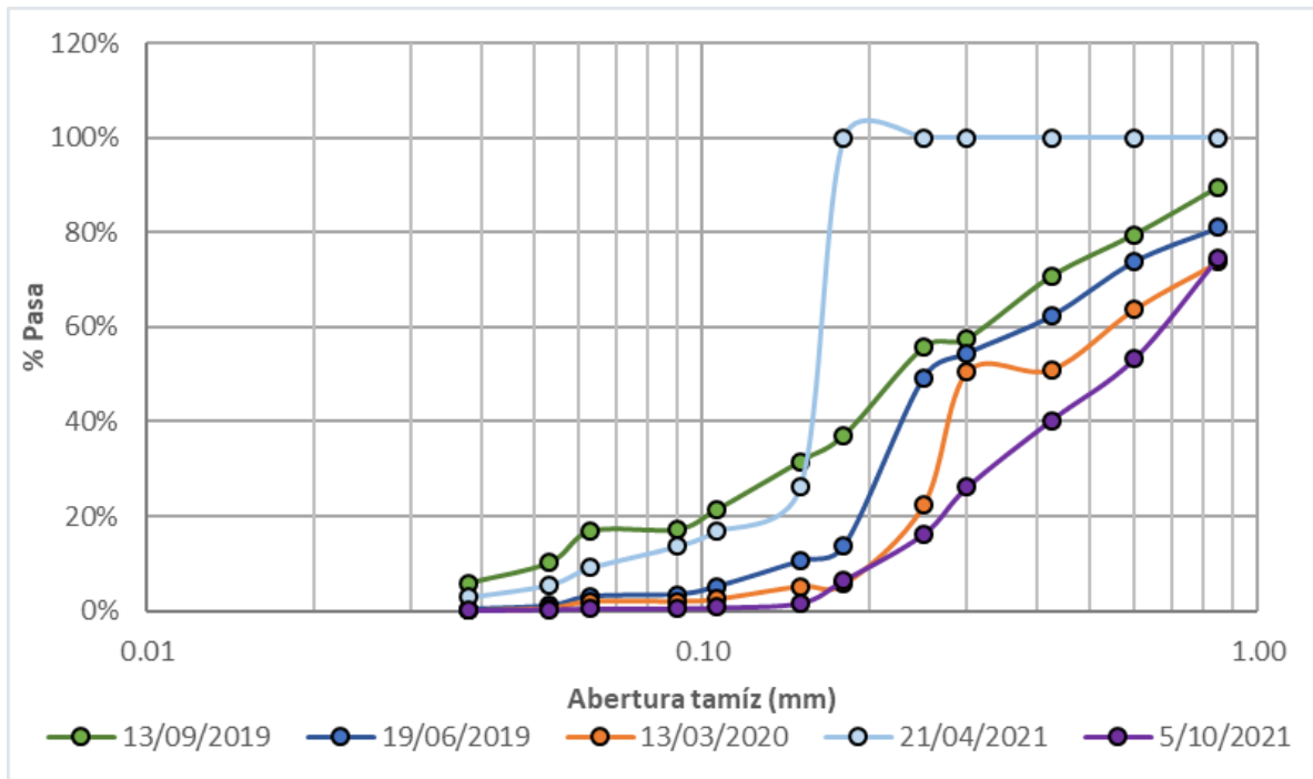
Figura 205. Granulometría sedimentos de fondo, Quebrada Olivares - El Popal
