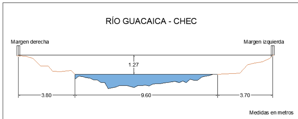
Figura 139. Sección transversal, Río Guacaica – CHEC, con medidas hechas en un cierto momento
