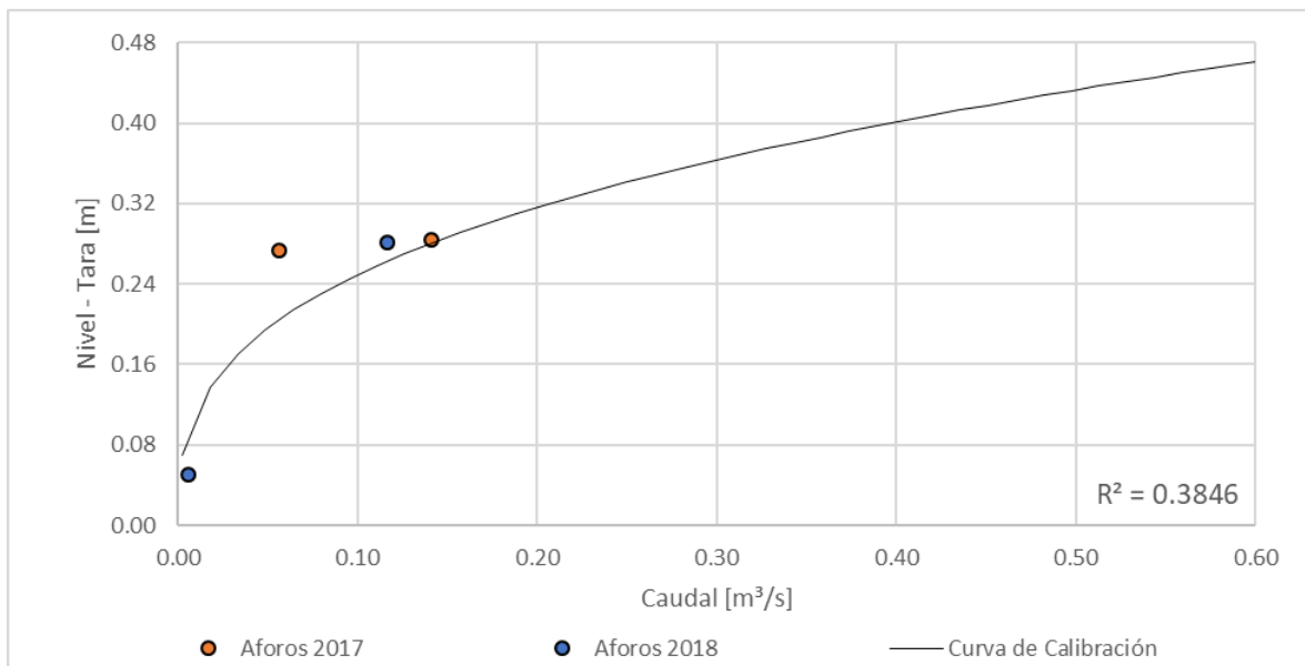
Figura 30. Curva nivel vs caudal, Quebrada El Perro – Expoferias
