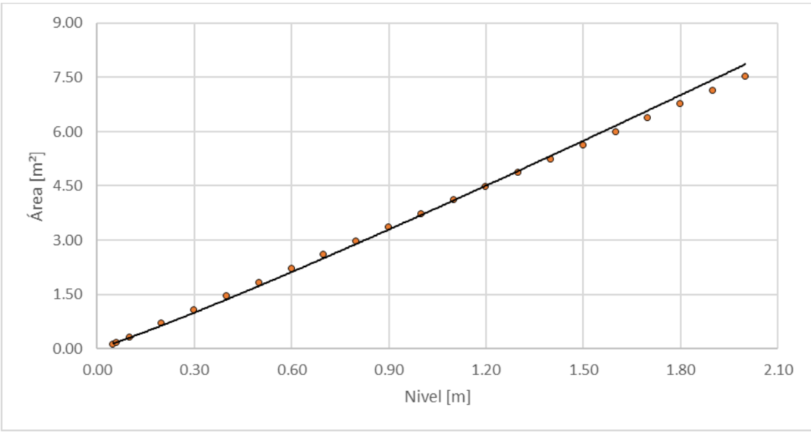
Figura 102. Nivel vs área, Quebrada Palogrande – Ruta 30
