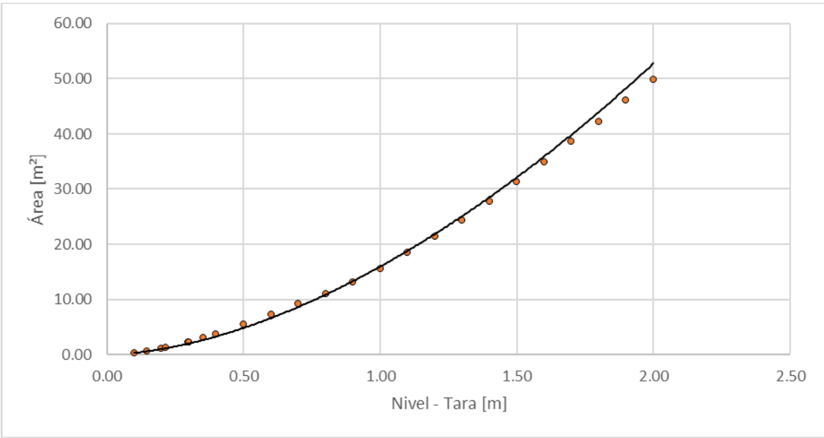
Figura 72. Nivel vs área, Quebrada Manzanares - Industrias Básicas de Caldas
