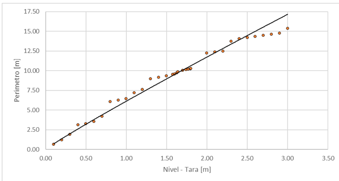
Figura 141. Nivel vs perímetro, Río Guacaica – CHEC
