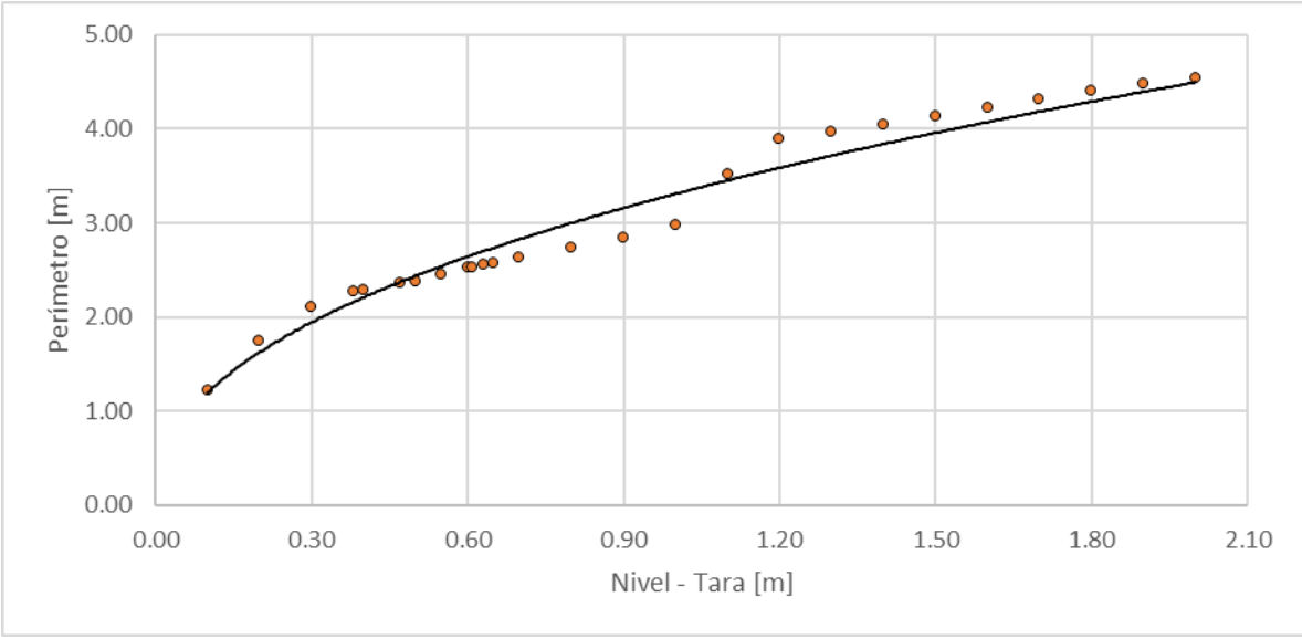
Figura 11. Nivel vs Perímetro, Quebrada Cristales - Valles de la Alhambra
