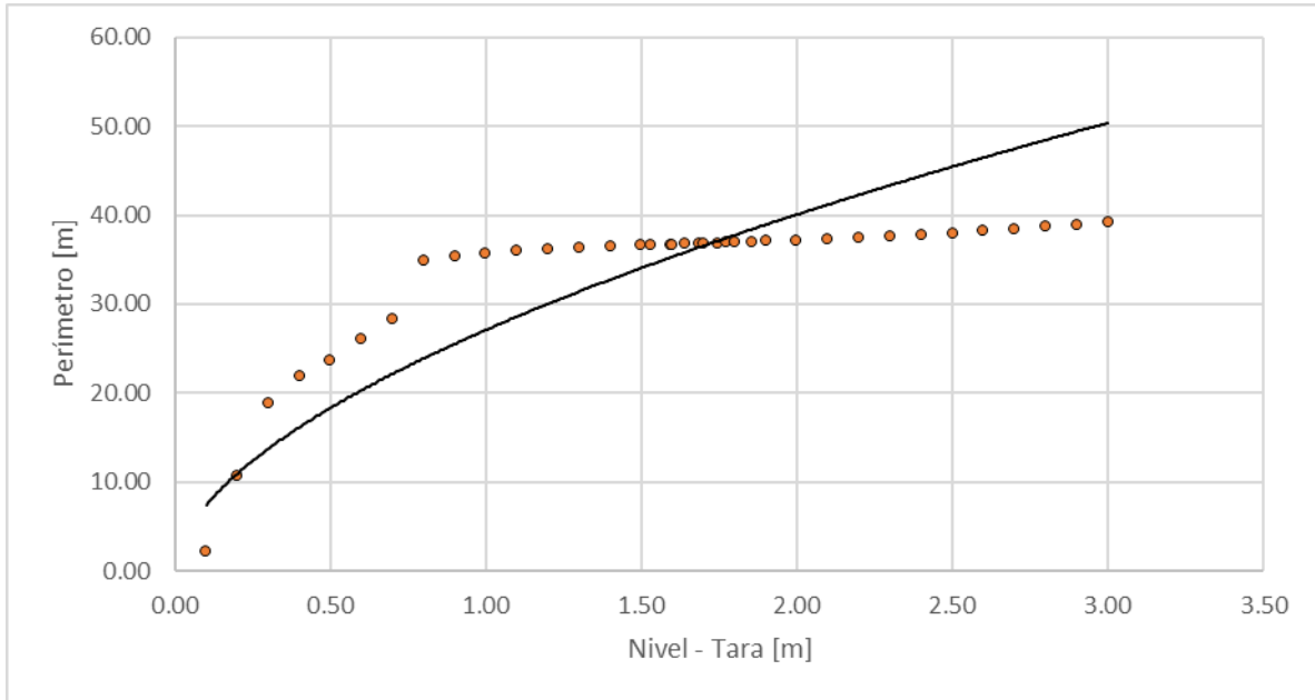
Figura 176. Nivel vs perímetro, Río Risaralda - Camping La Palmera
