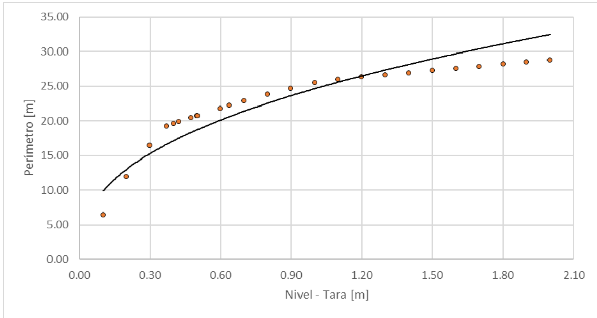
Figura 196. Nivel vs perímetro, Río Tapias
