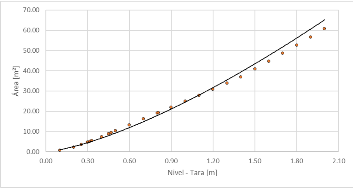
Figura 127. Nivel vs área, Río Chinchiná - Cenicafé
