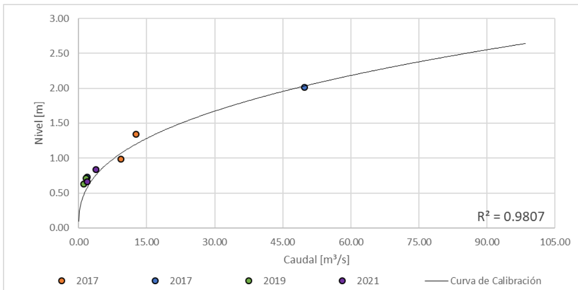
Figura 135. Curva nivel vs caudal, Río Doña Juana - Vía La Dorada Norcasia
