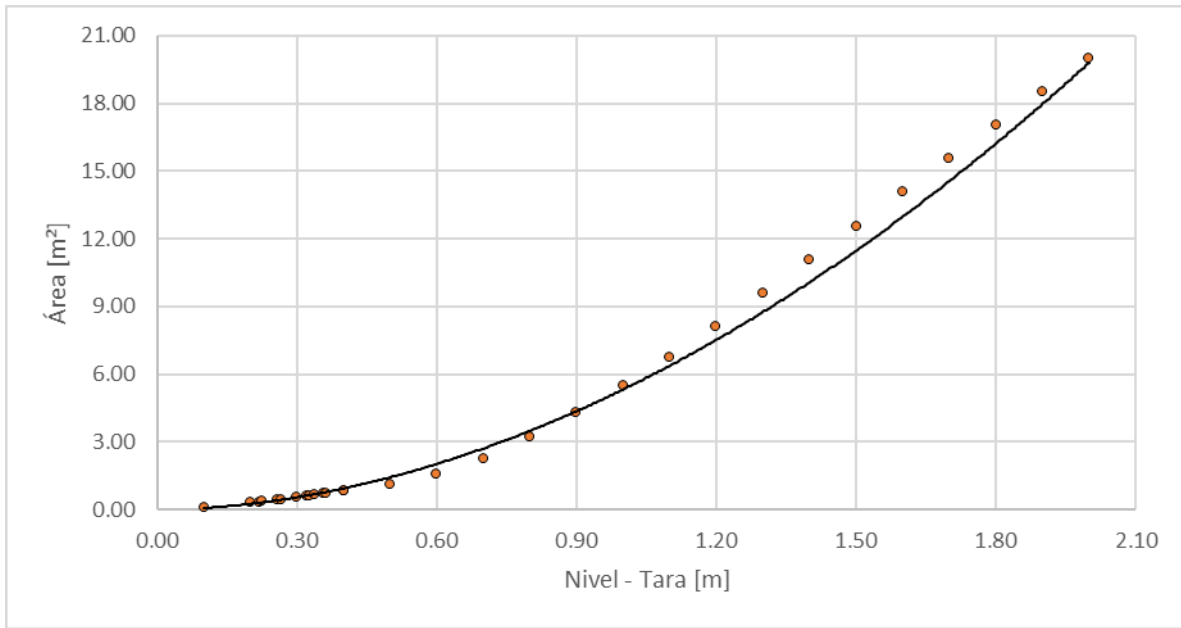
Figura 87. Nivel vs área, Quebrada Olivares - Bocatoma
