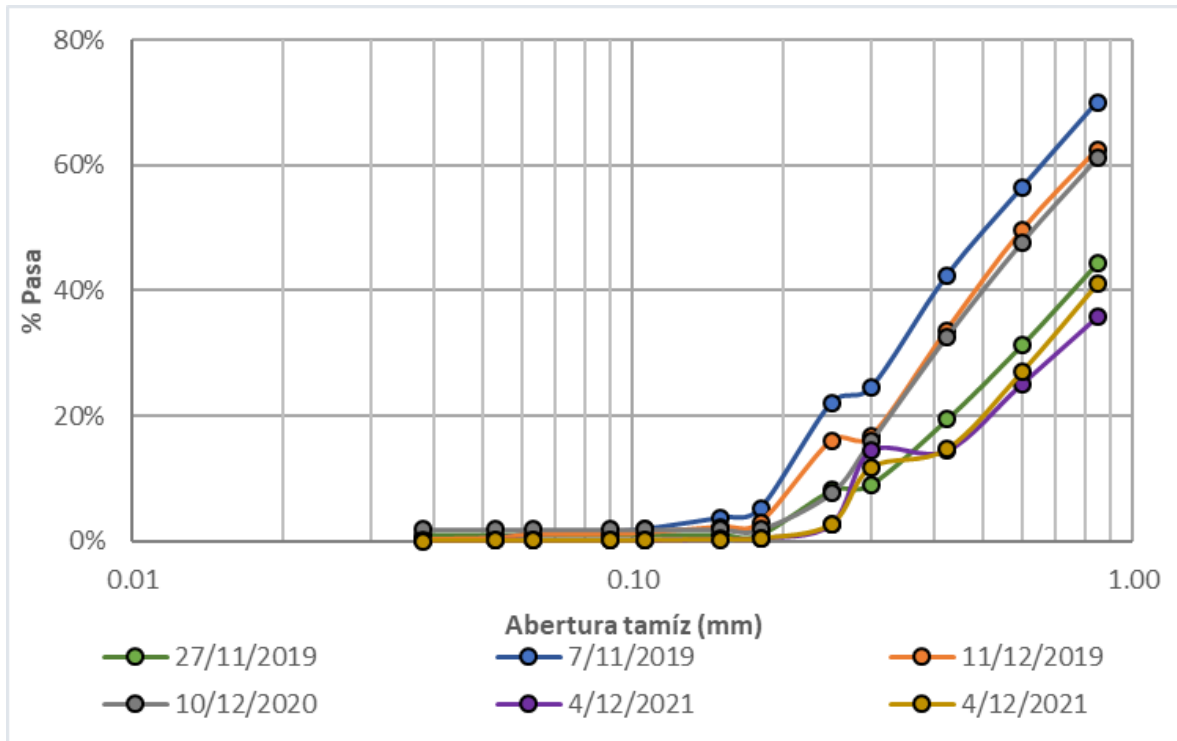
Figura 213. Granulometría sedimentos de fondo, Río Chinchiná – El Bosque
