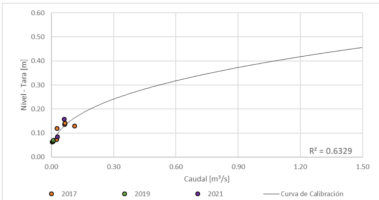
Figura 20. Curva nivel vs caudal, Quebrada el Guamo - CDI San Sebastián
