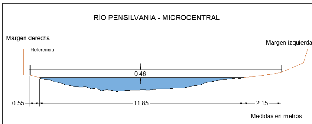
Figura 154. Sección transversal, Río Pensilvania – Microcentral, con medidas hechas en un cierto momento
