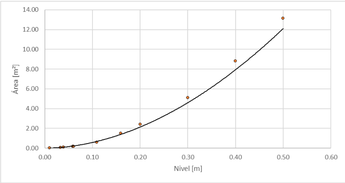
Figura 47. Nivel vs área, Quebrada El Triunfo - Mirador de Villapilar
