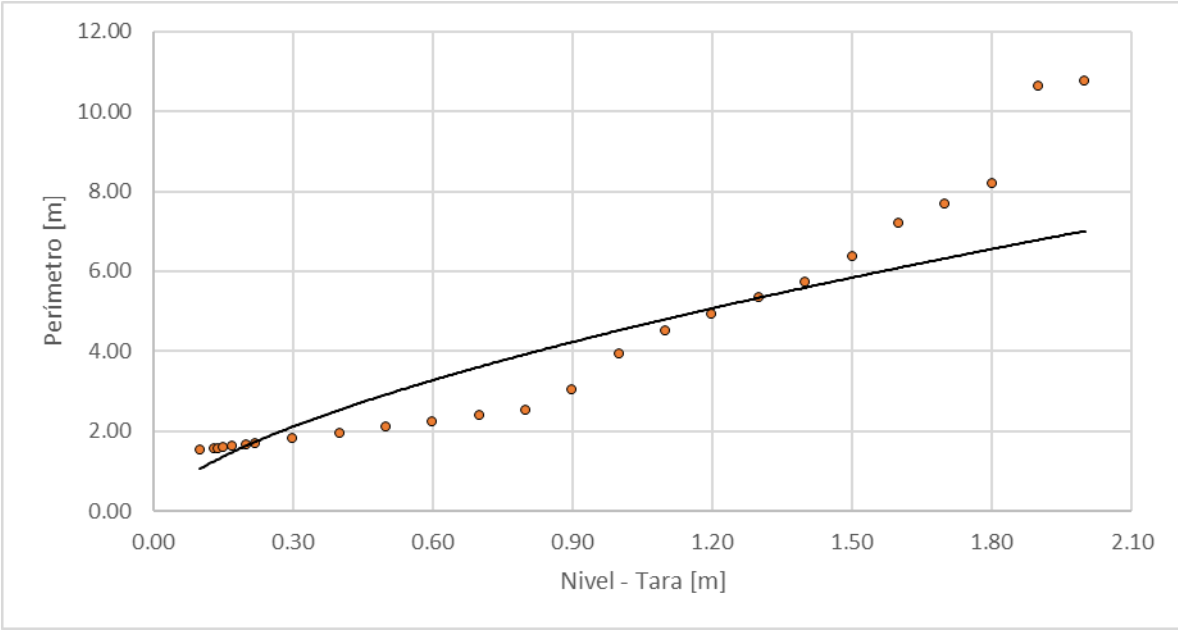
Figura 111. Nivel vs perímetro, Quebrada Salinas - Relleno sanitario EMAS
