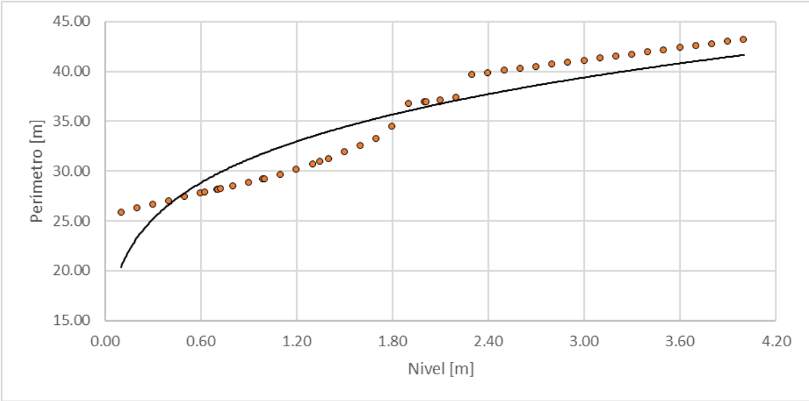
Figura 136. Nivel vs Perímetro, Río Doña Juana - Vía La Dorada Norcasia
