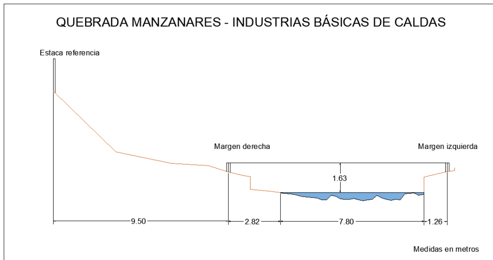
Figura 69. Sección transversal, Quebrada Manzanares - Industrias Básicas de Caldas, con medidas hechas en un cierto momento.
