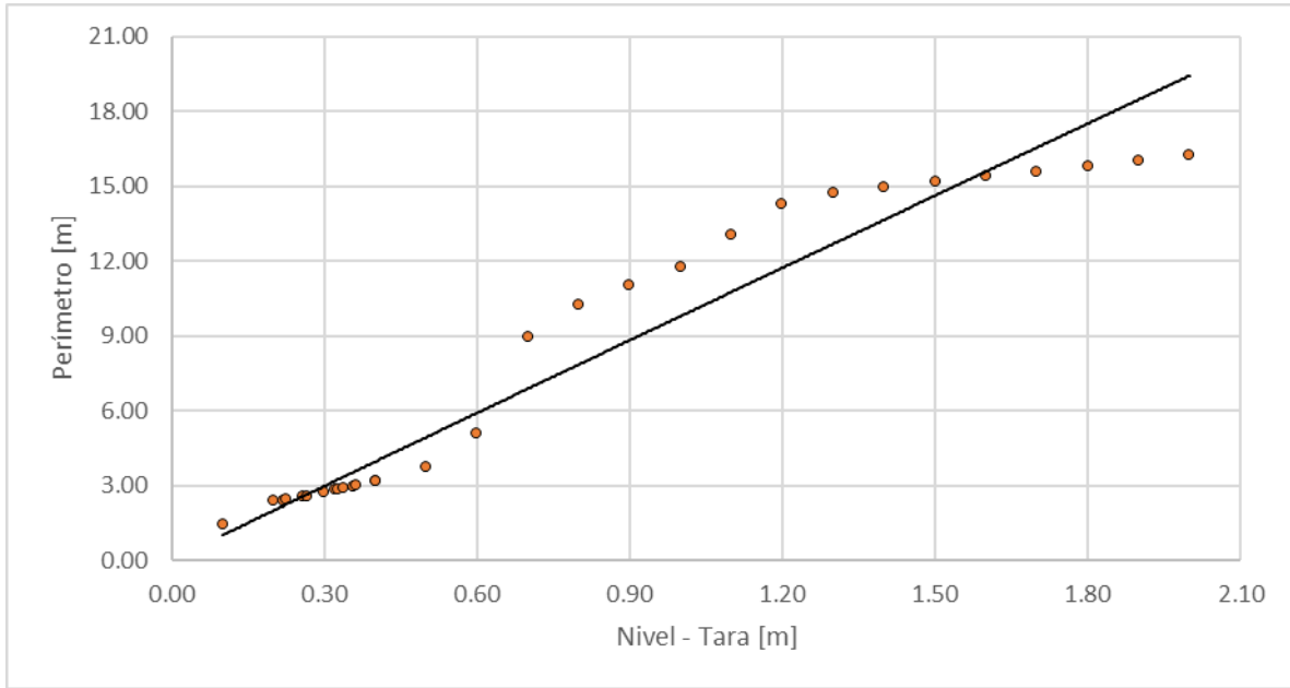
Figura 86. Nivel vs perímetro, Quebrada Olivares - Bocatoma
