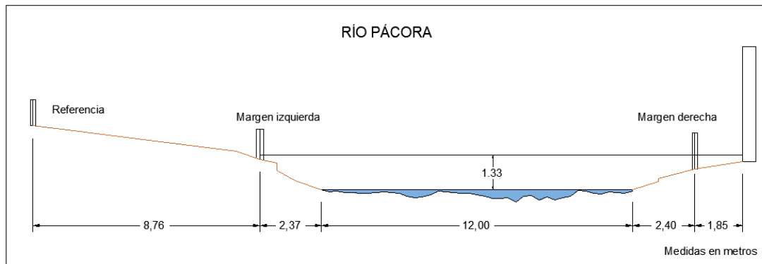
Figura 149. Sección transversal, Río Pácora, con medidas hechas en un cierto momento
