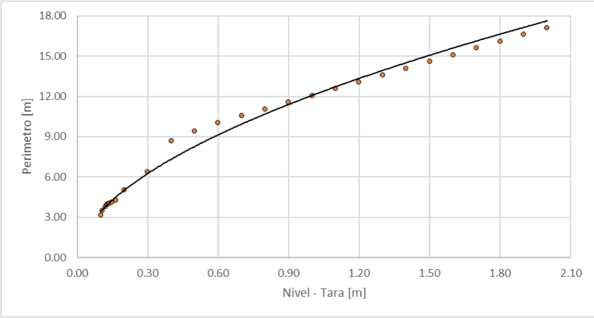
Figura 66. Nivel vs Perímetro, Quebrada Manizales – Skinco
