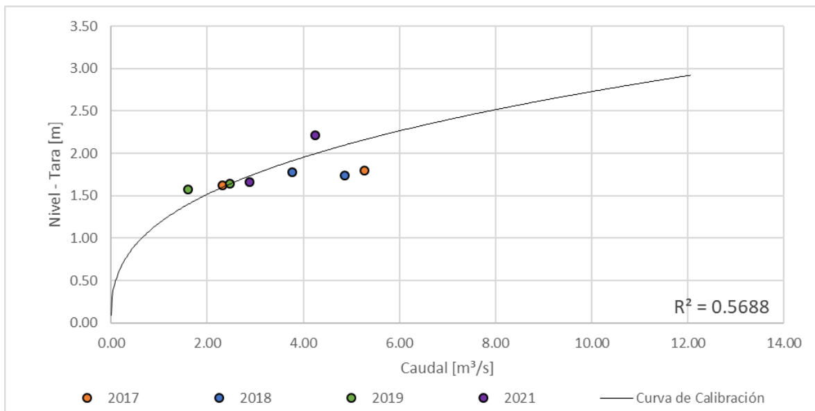
Figura 140. Curva nivel vs caudal, Río Guacaica – CHEC
