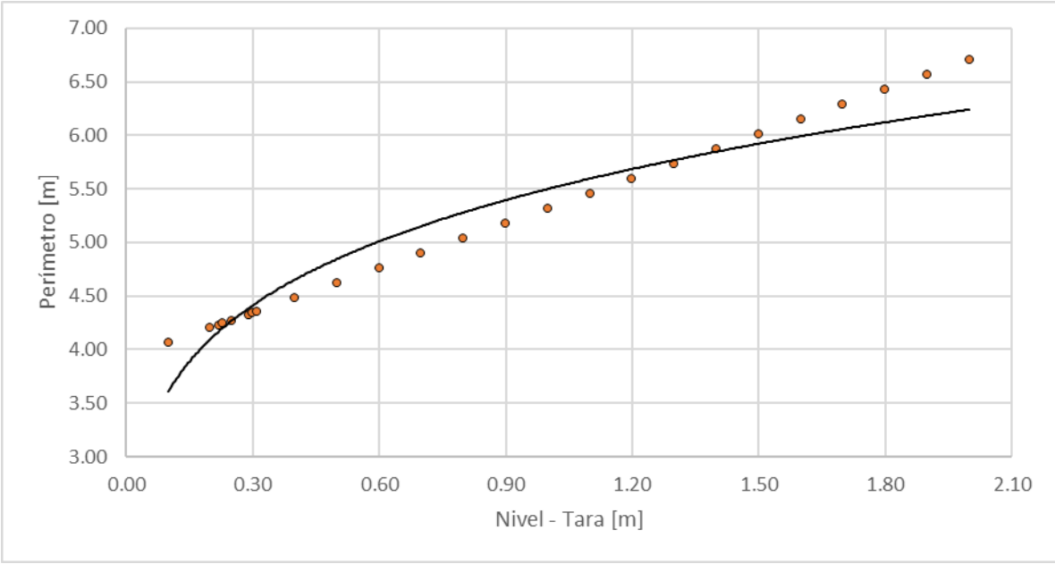
Figura 61. Nivel vs perímetro, Quebrada Las Pavas - Autopistas del Café
