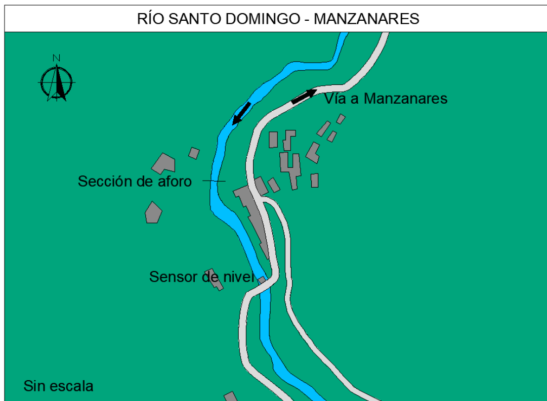
Figura 178. Vista en planta, Río Santo Domingo - Manzanares
