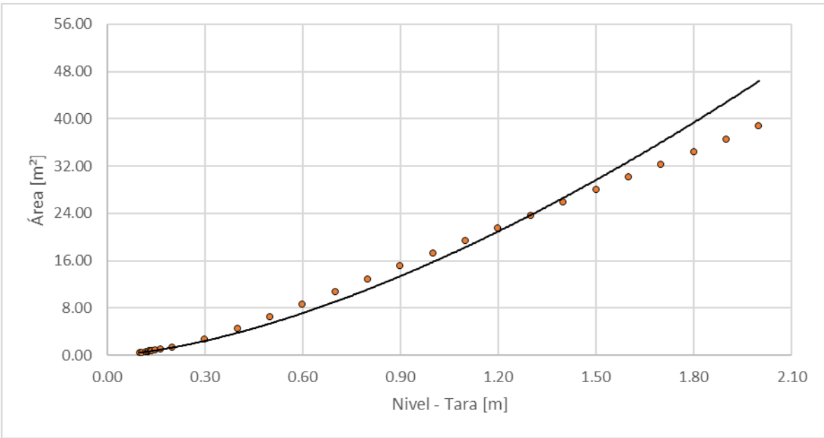
Figura 67. Nivel vs área, Quebrada Manizales – Skinco
