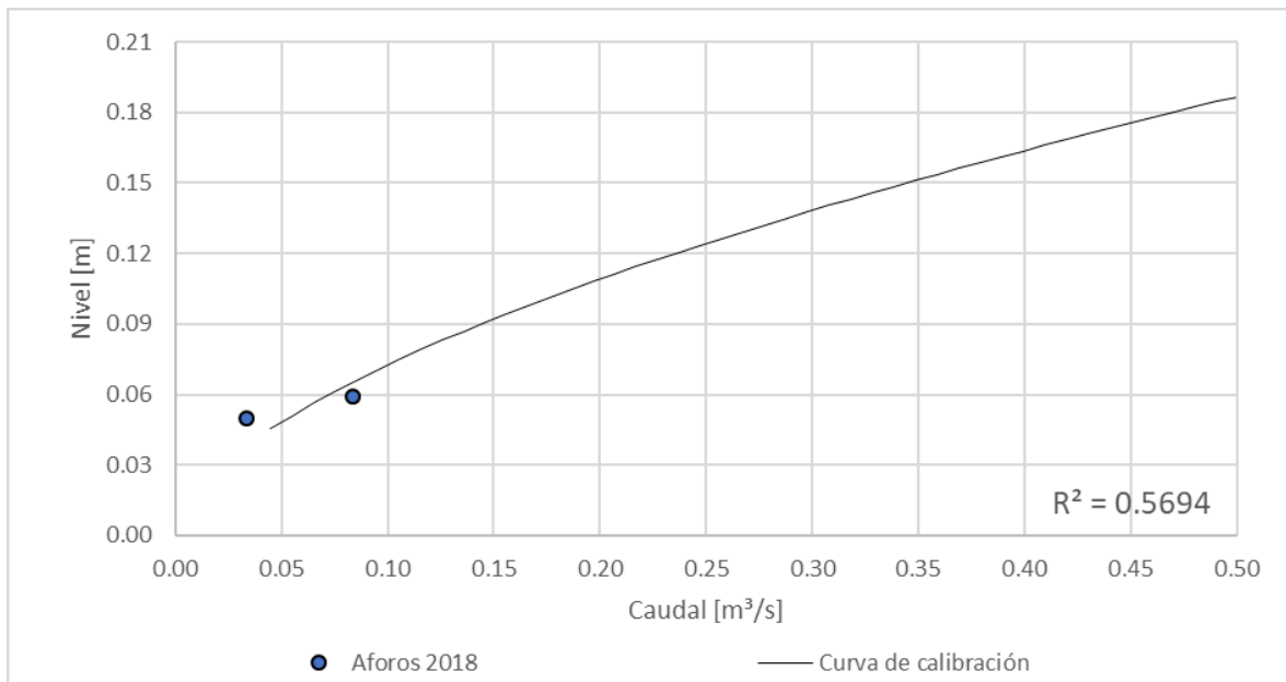
Figura 100. Curva nivel vs caudal, Quebrada Palogrande – Ruta 30
