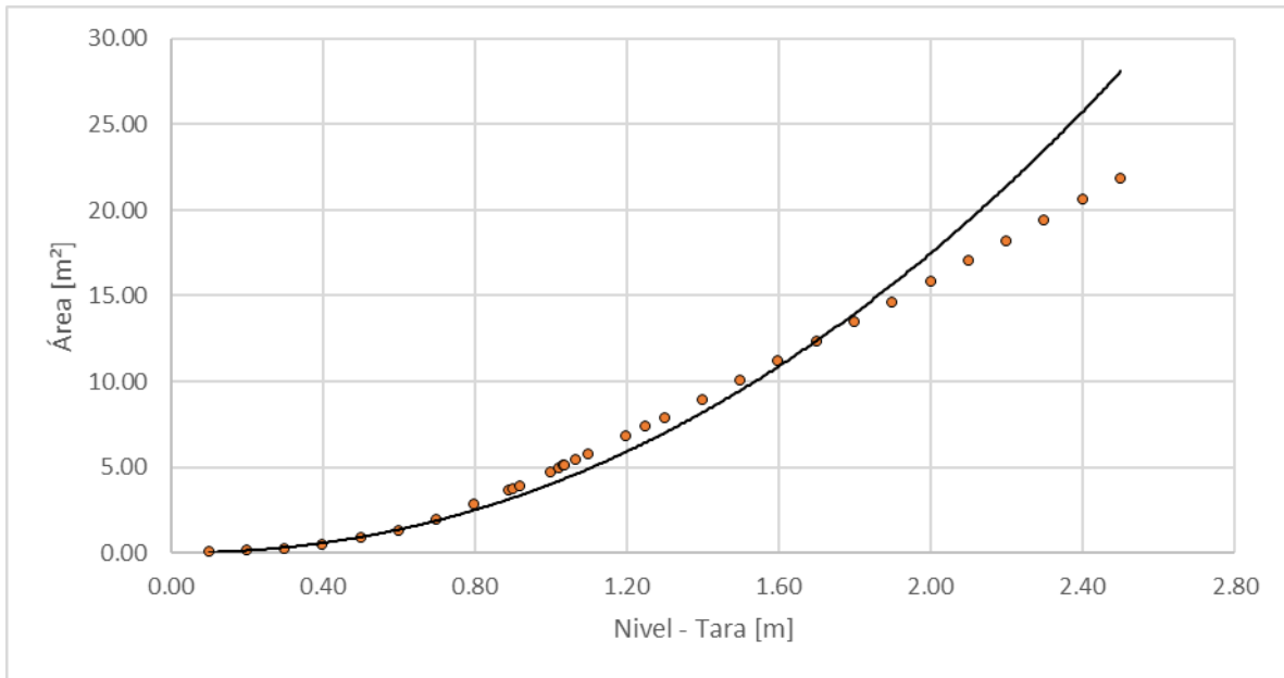
Figura 167. Nivel vs área, Río Rioclaro - La Batea
