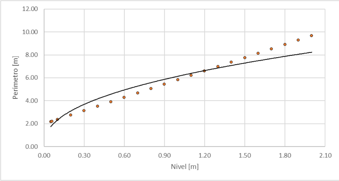
Figura 101. Nivel vs perímetro, Quebrada Palogrande – Ruta 30
