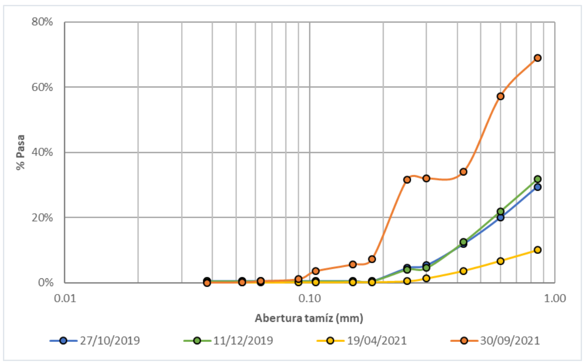
Figura 199. Granulometría sedimentos de fondo, Quebrada El Rosario - Autopistas
