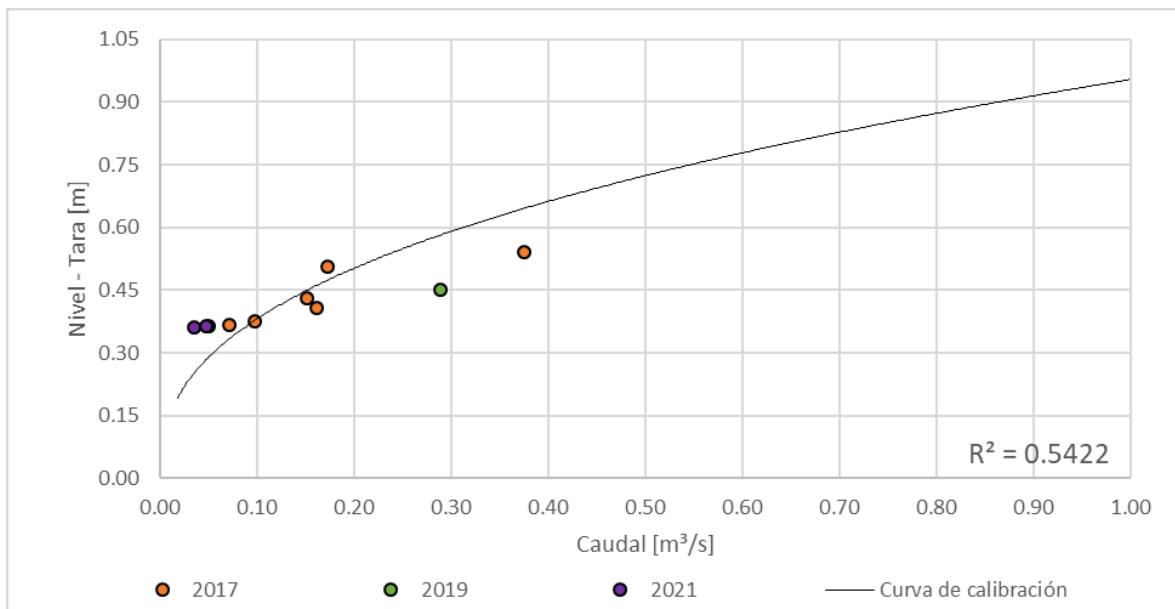
Figura 50. Curva nivel vs caudal, Quebrada Guayabal - Recinto del pensamiento
