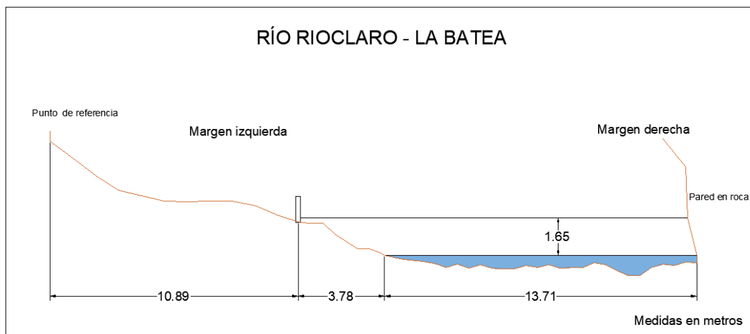
Figura 164. Sección transversal, Río Rioclaro - La Batea, con medidas hechas en un cierto momento
