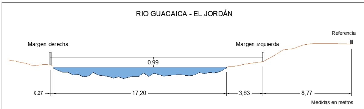
Figura 144. Sección Transversal, Río Guacaica - El Jordán, con medidas hechas en un cierto momento
