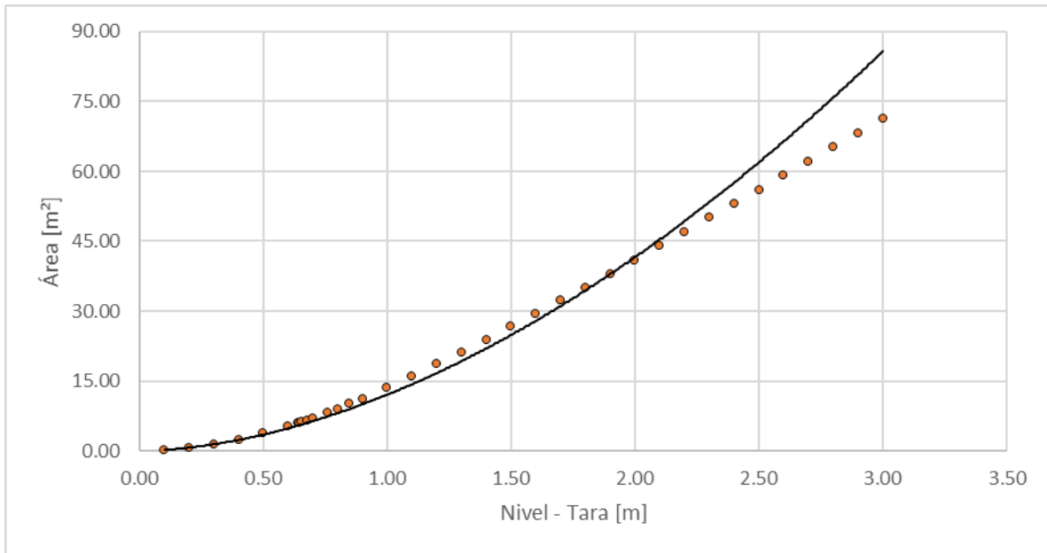
Figura 162. Nivel vs área, Río Pozo – Vía La Merced Pácora
