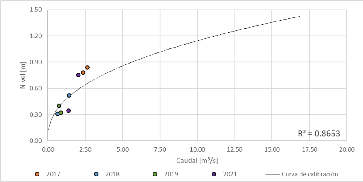
Figura 150. Curva nivel vs caudal, Río Pácora
