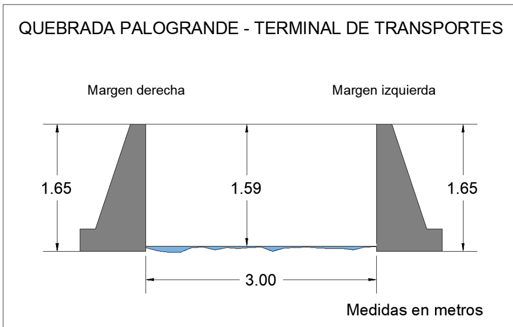
Figura 104. Sección transversal, Quebrada Palogrande - Terminal de transportes, con medidas hechas en un cierto momento.
