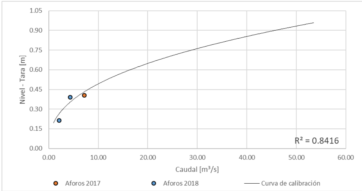
Figura 190. Curva nivel vs caudal, Río Supía – Supía
