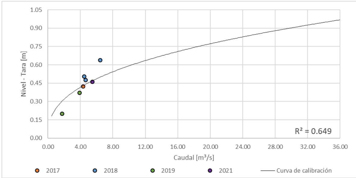
Figura 195. Curva nivel vs caudal, Río Tapias
