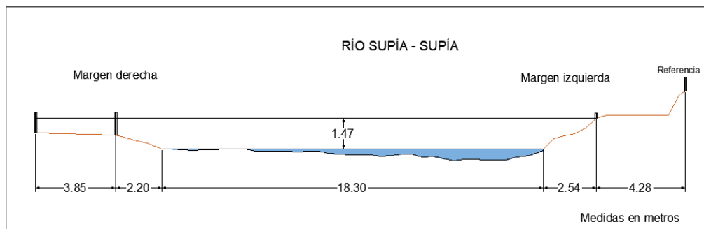
Figura 189. Sección transversal, Río Supía – Supía, con medidas hechas en un cierto momento
