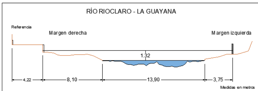
Figura 169. Sección transversal, Río Rioclaro – La Guayana, con medidas hechas en un cierto momento
