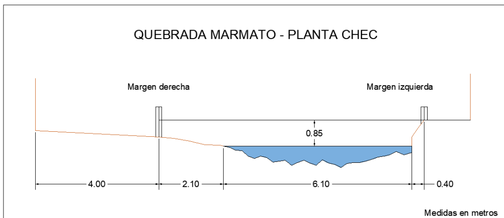
Figura 74. Sección transversal, Quebrada Marmato - Planta Intermedia CHEC, con medidas hechas en un cierto momento.
