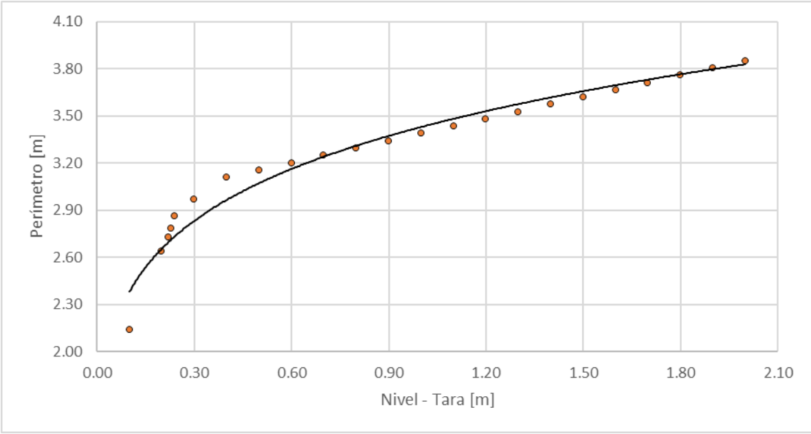
Figura 106. Nivel vs perímetro, Quebrada Palogrande - Terminal de transportes
