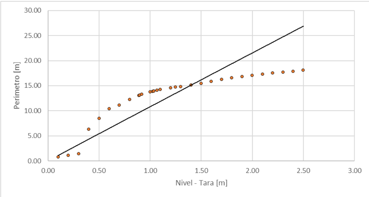
Figura 166. Nivel vs Perímetro, Río Rioclaro - La Batea
