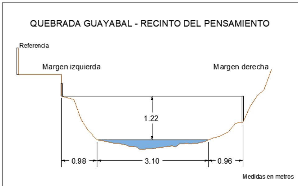
Figura 49. Sección transversal, Quebrada Guayabal - Recinto del pensamiento, con medidas hechas en un cierto momento
