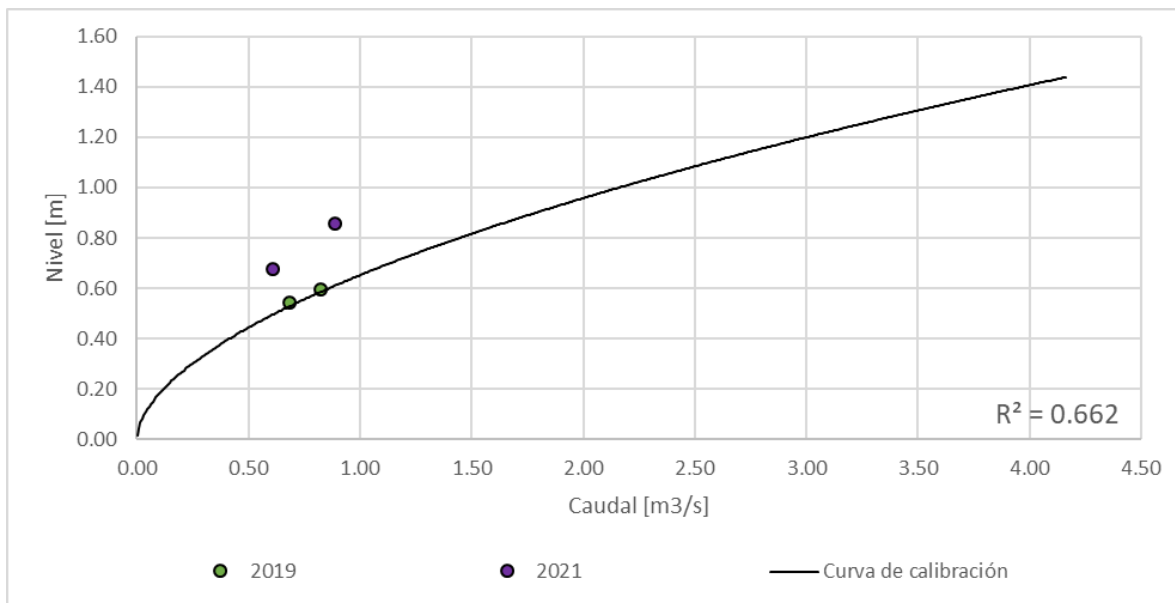
Figura 35. Curva nivel vs caudal, Quebrada el Rosario – Autopistas
