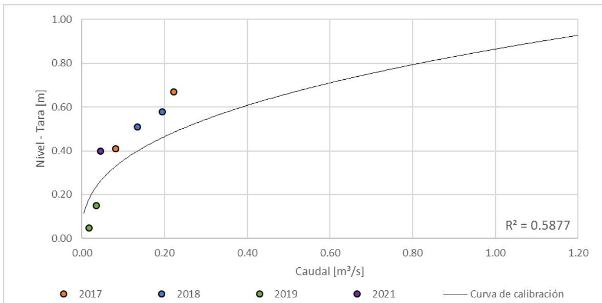
Figura 40. Curva nivel vs caudal, Quebrada El Rosario - San Marcos de León
