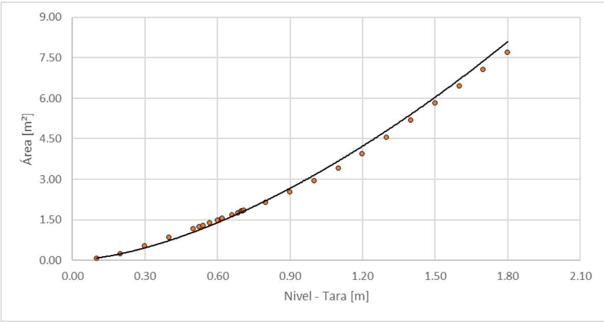
Figura 97. Nivel vs área, Quebrada Olivares - El Popal
