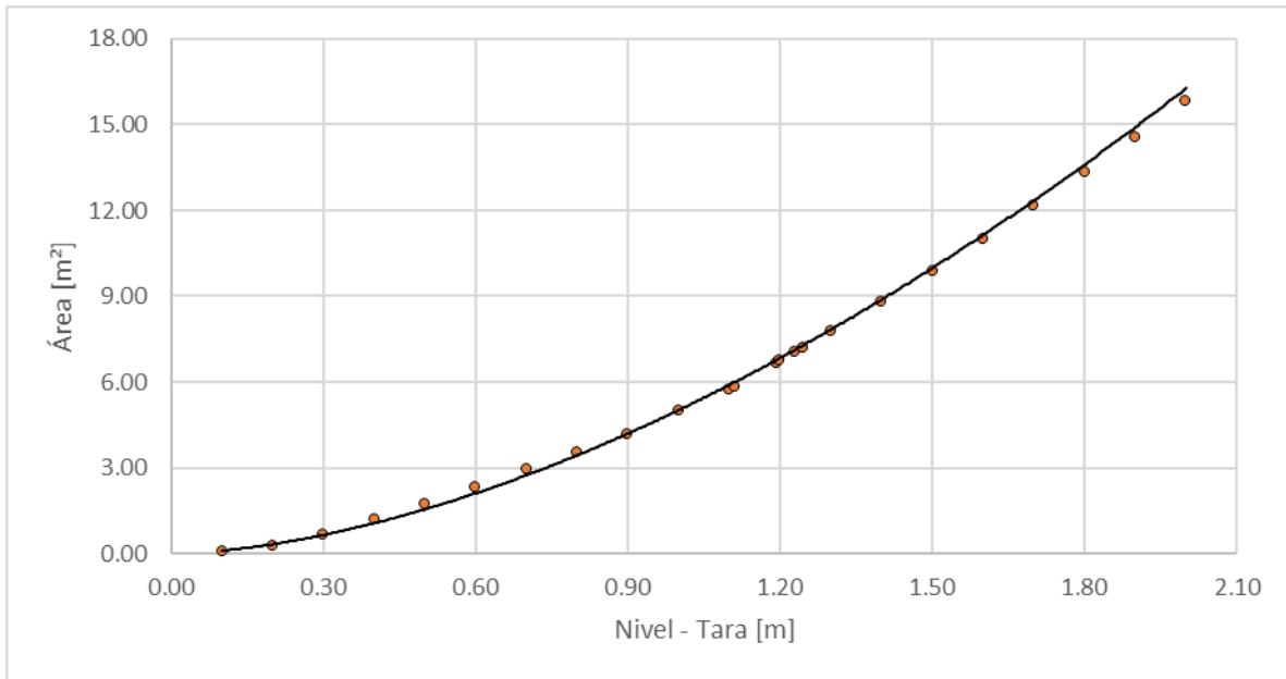
Figura 172. Nivel vs área, Río Rioclaro - La Guayana
