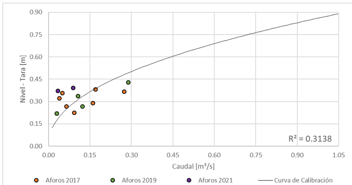
Figura 85. Curva nivel vs caudal, Quebrada Olivares - Bocatoma
