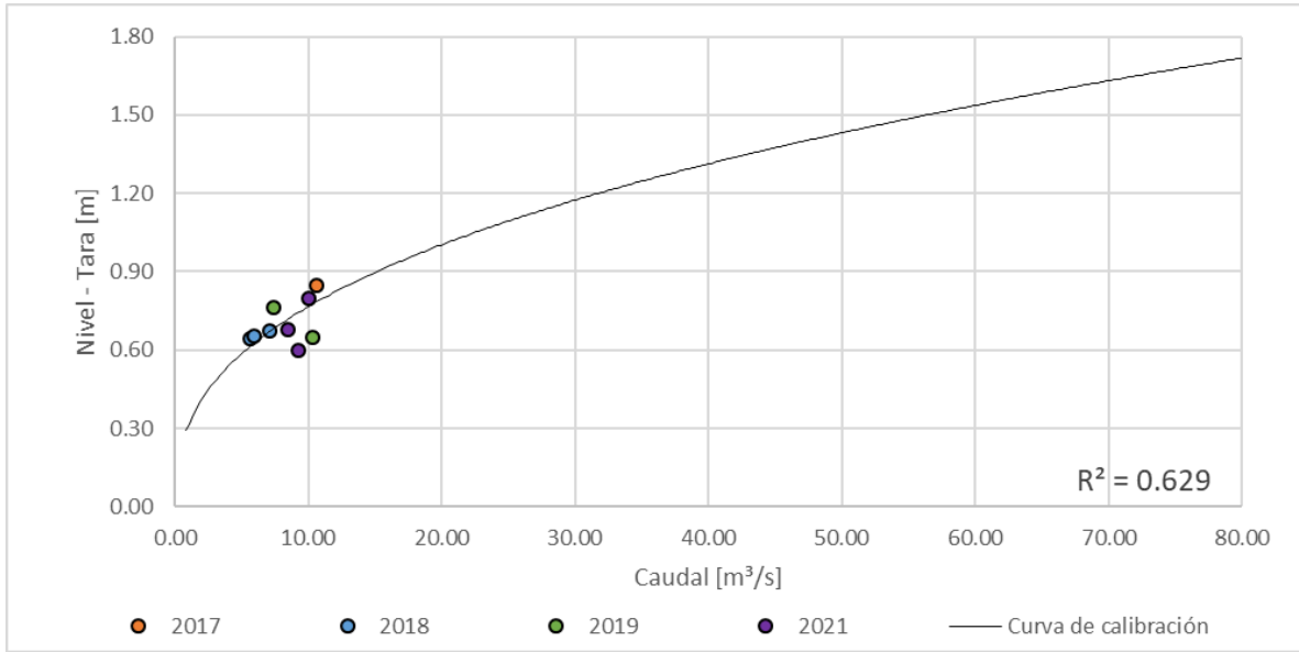
Figura 160. Curva nivel vs caudal, Río Pozo – Vía La Merced Pácora
