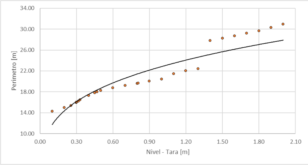
Figura 126. Nivel vs Perímetro, Río Chinchiná - Cenicafé
