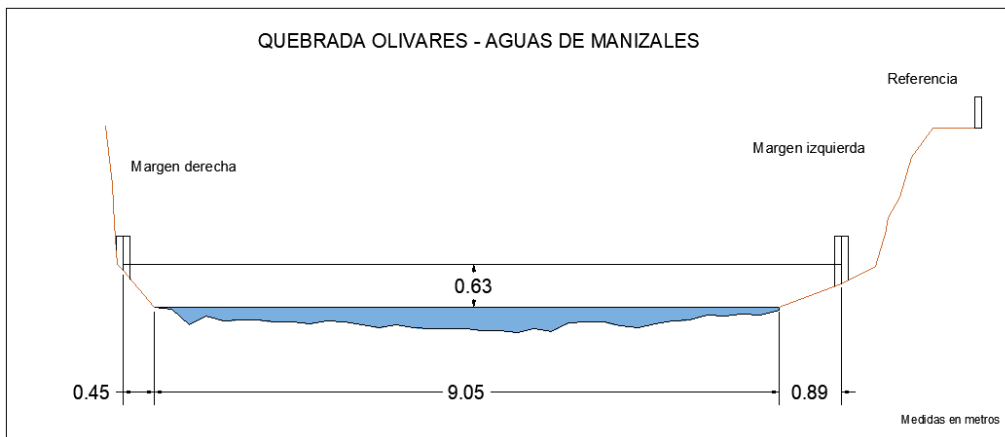
Figura 79. Sección transversal, Quebrada Olivares - Aguas de Manizales, con medidas hechas en un cierto momento
