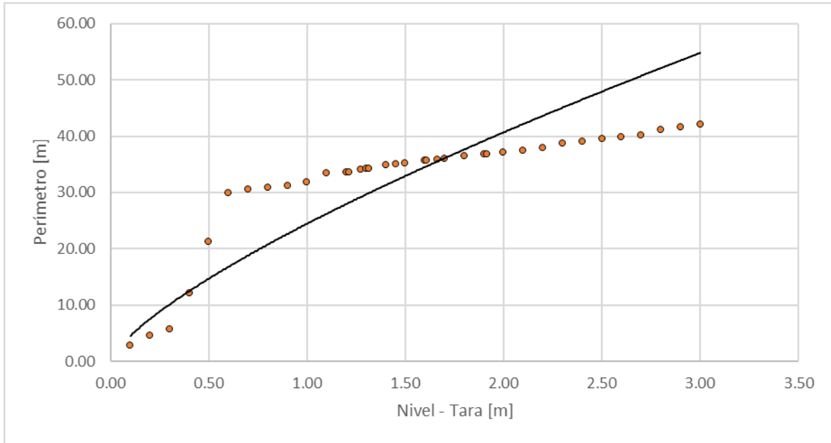
Figura 186. Nivel vs perímetro, Río Supía - Los Piononos
