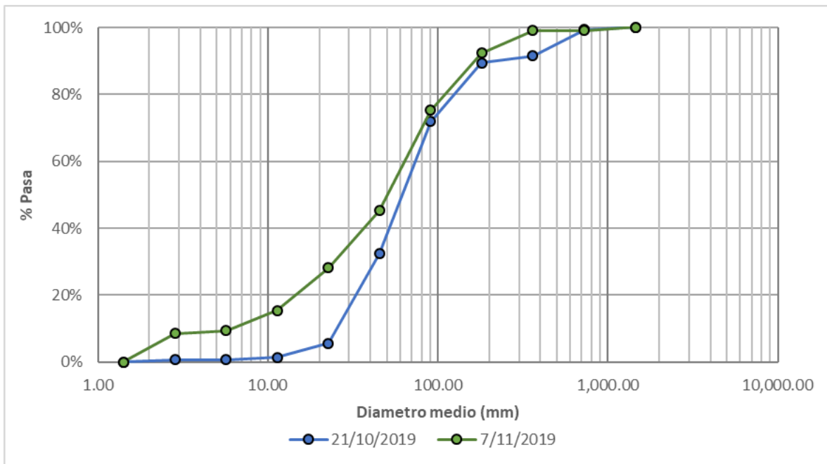
Figura 211. Granulometría material del lecho (conteo de Wolman), Río Chinchiná - Cenicafé
