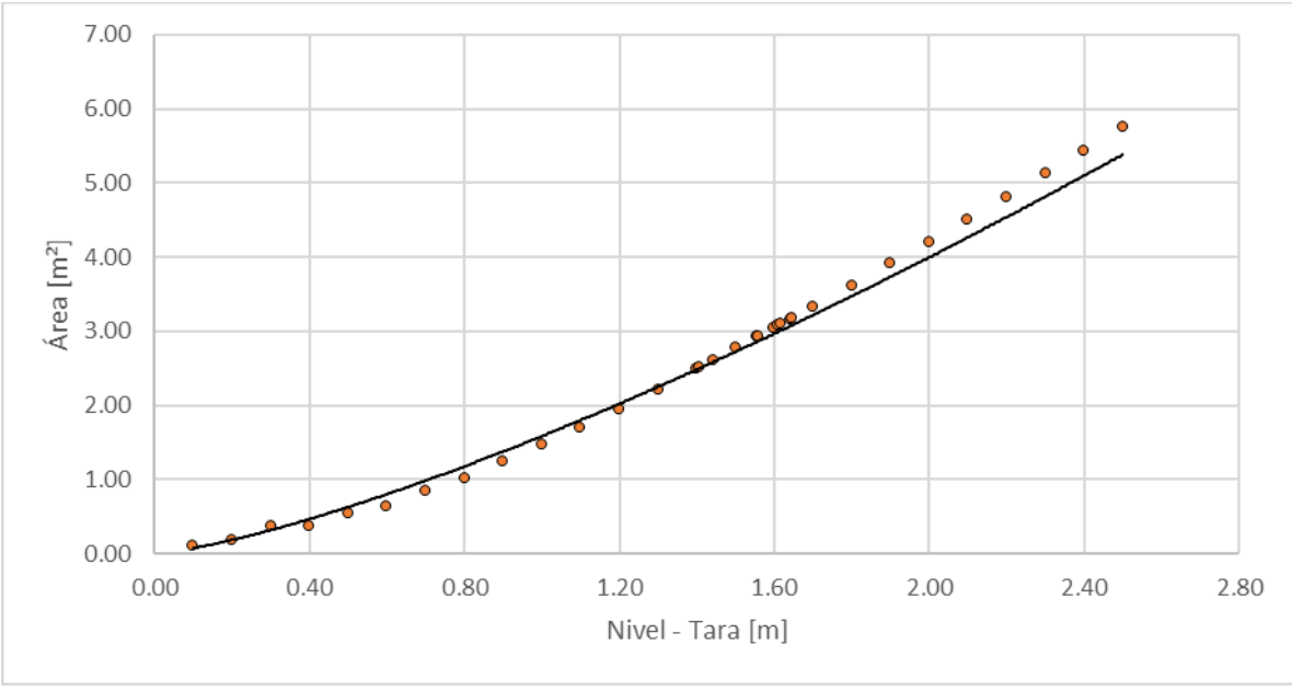
Figura 92. Nivel vs Área, Quebrada Olivares - Bomberos voluntarios
