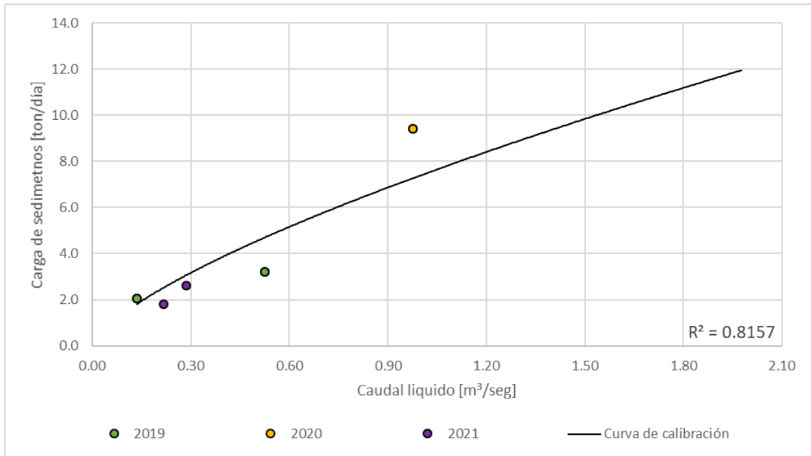
Figura 204. Relación caudal líquido - caudal sólido, Quebrada Olivares - El Popal
