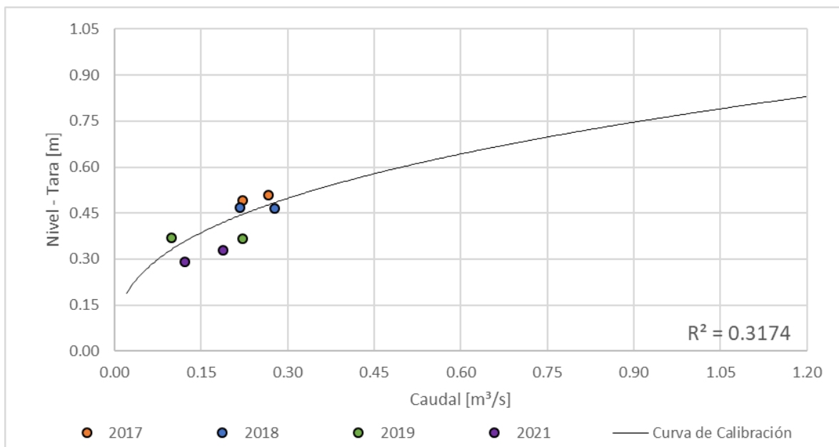
Figura 75. Curva nivel vs caudal, Quebrada Marmato - Planta Intermedia CHEC
