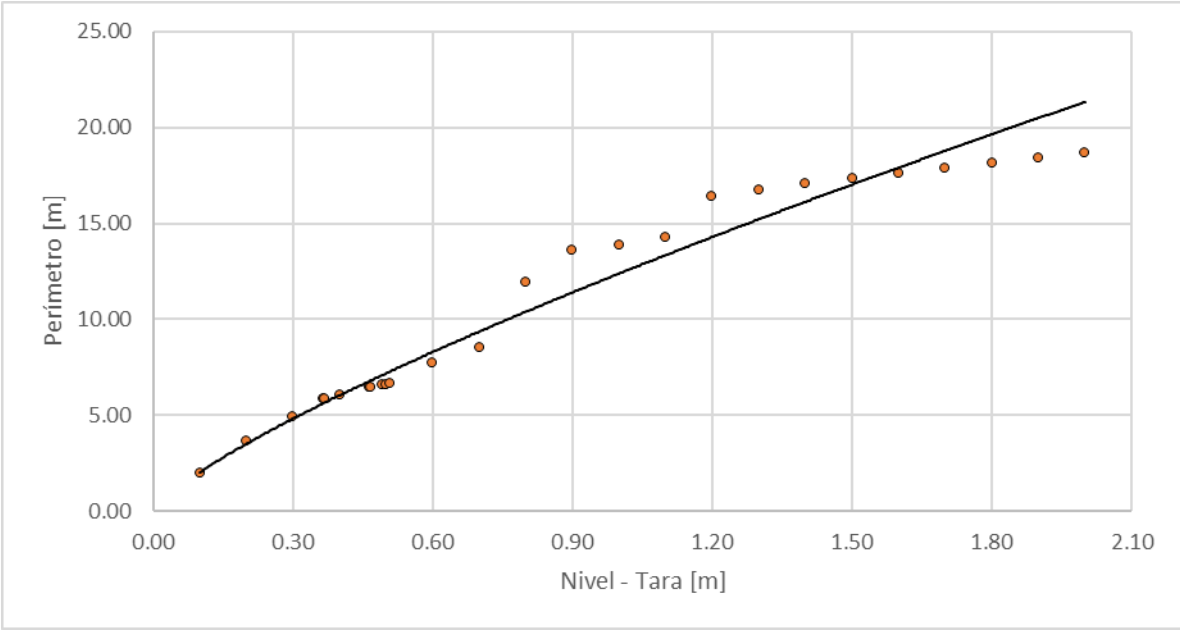
Figura 76. Nivel vs perímetro, Quebrada Marmato - Planta Intermedia CHEC
