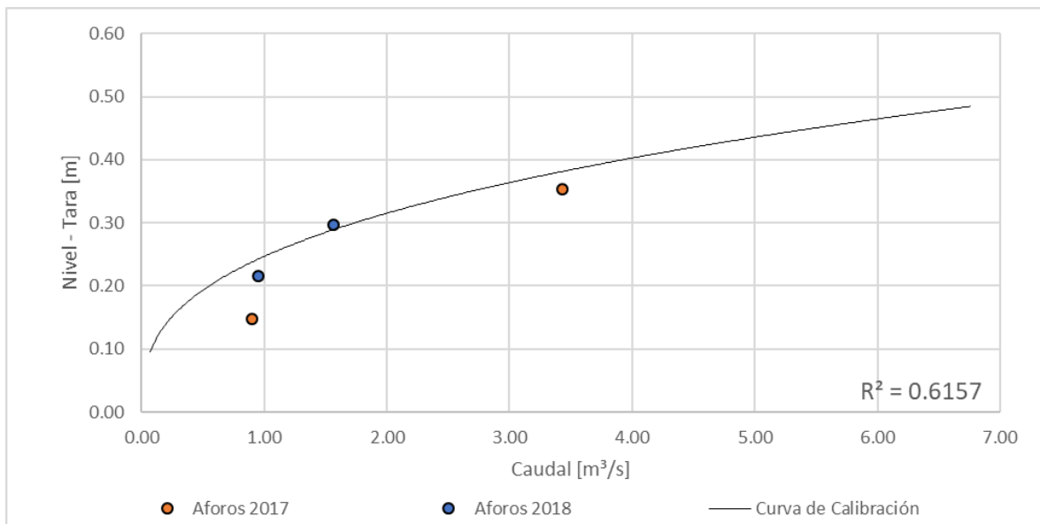
Figura 70. Curva nivel vs caudal, Quebrada Manzanares - Industrias Básicas de Caldas
