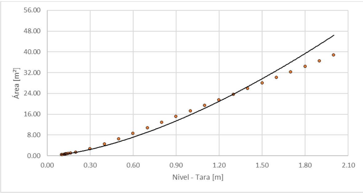
Figura 57. nivel vs área, Quebrada La Francia - Los Puentes
