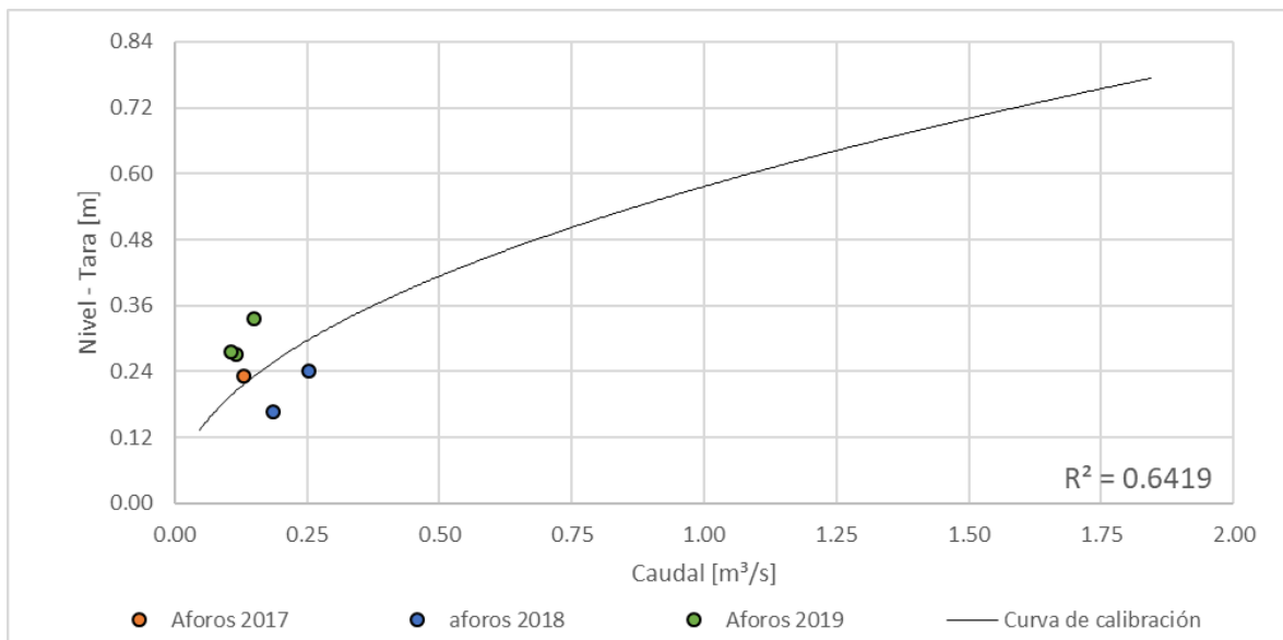
Figura 115. Curva nivel vs caudal, Quebrada Tesorito – Vía al Magdalena
