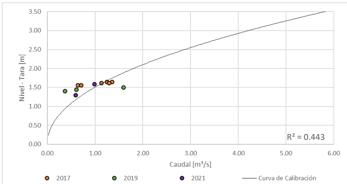
Figura 90. Curva nivel vs caudal, Quebrada Olivares - Bomberos voluntarios
