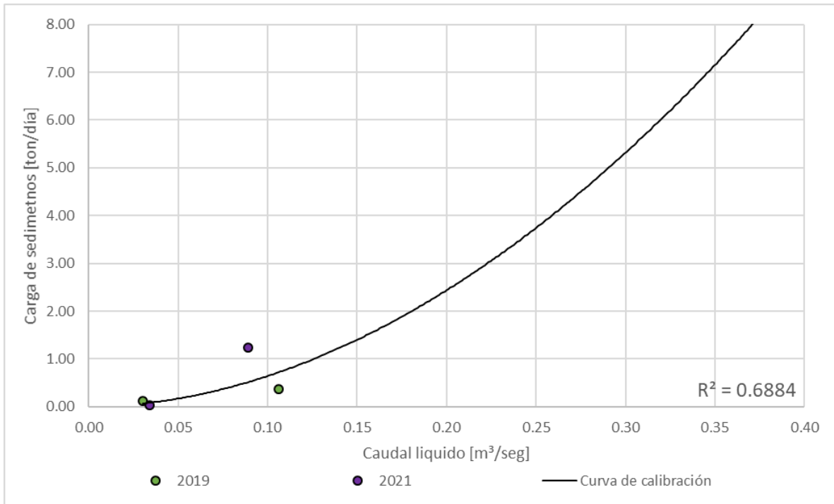
Figura 201. Relación caudal líquido - caudal sólido, Quebrada Olivares - Bocatoma
