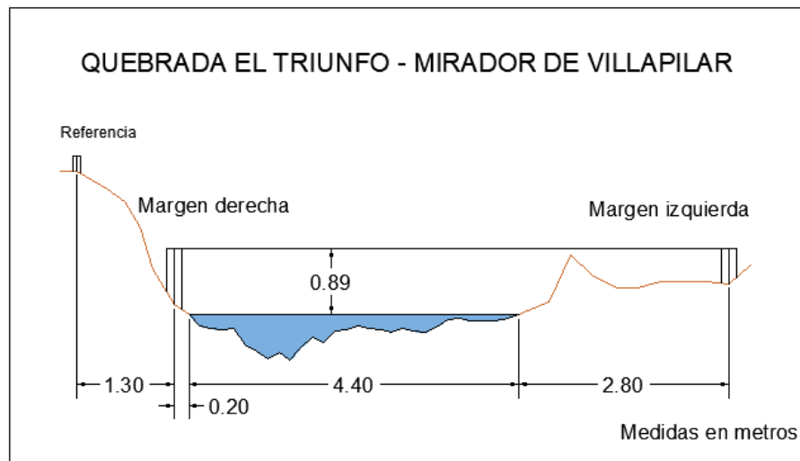
Figura 44. Sección transversal, Quebrada El Triunfo - Mirador de Villapilar, con medidas hechas en un cierto momento
