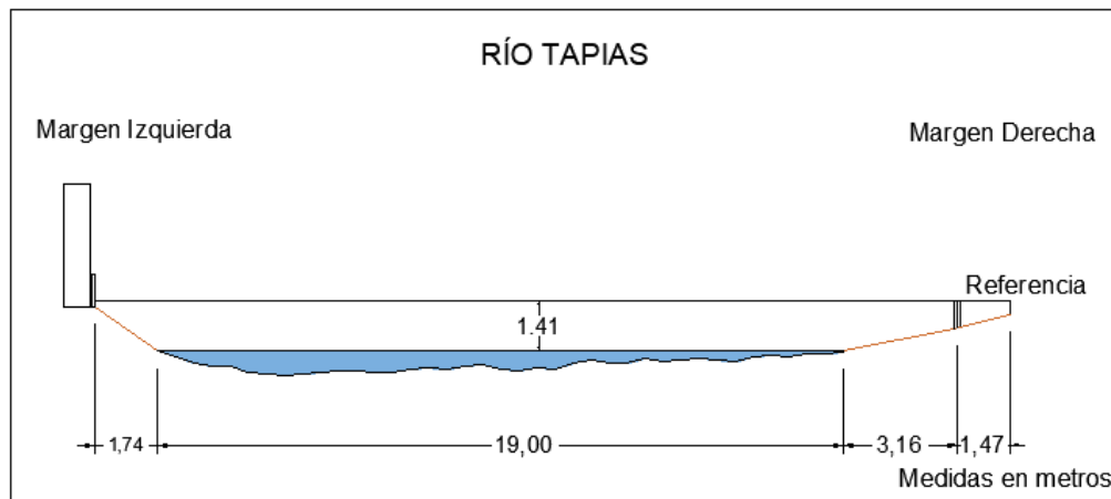
Figura 194. Sección transversal, Río Tapias, con medidas hechas en un cierto momento
