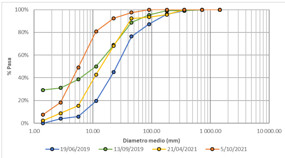
Figura 203. Granulometría material del lecho (conteo de Wolman), Quebrada Olivares – Bocatoma
