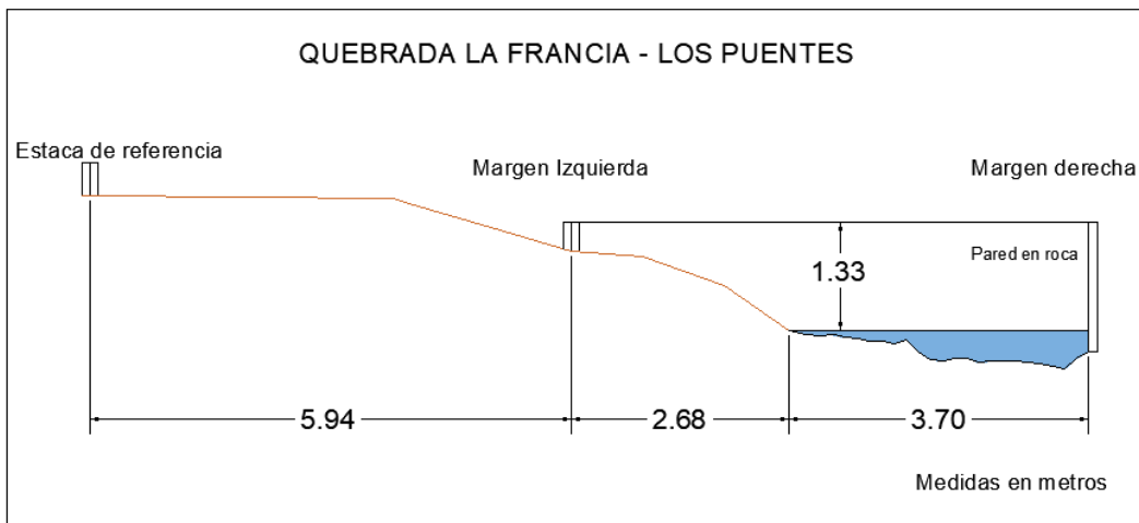
Figura 54. Sección transversal, Quebrada La Francia - Los Puentes, con medidas hechas en un cierto momento
