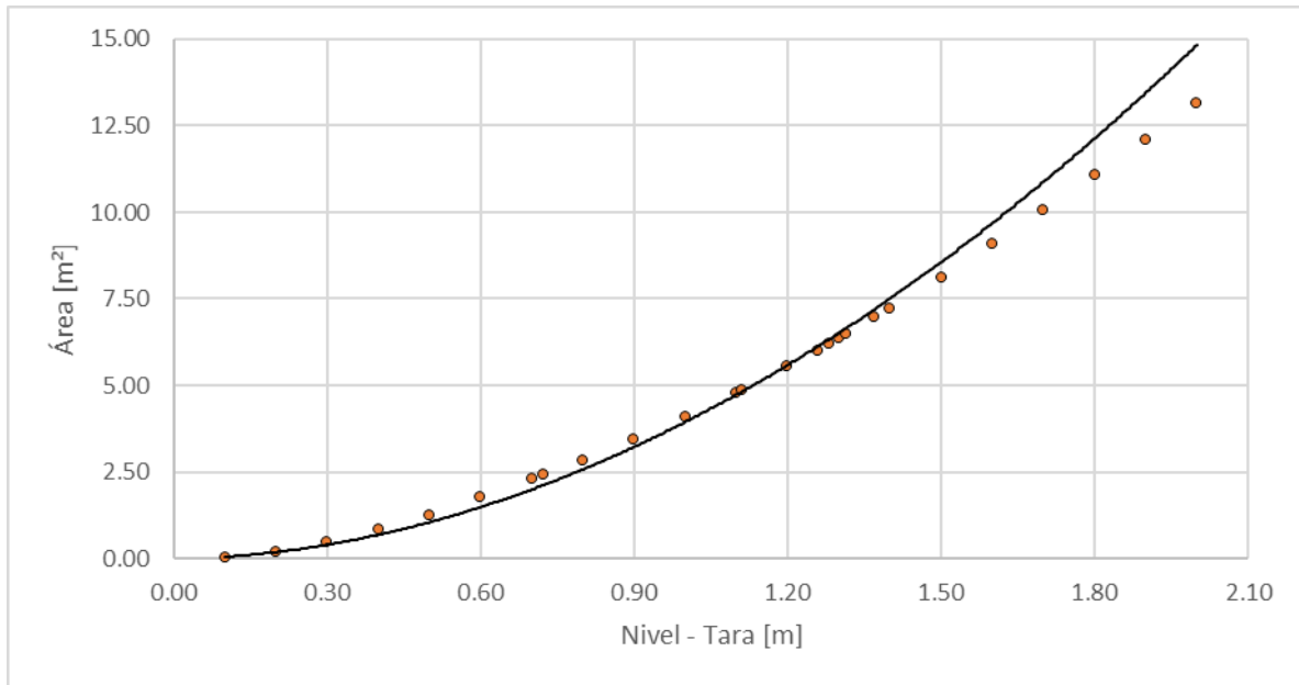
Figura 157. Nivel vs área, Río Pensilvania – Microcentral
