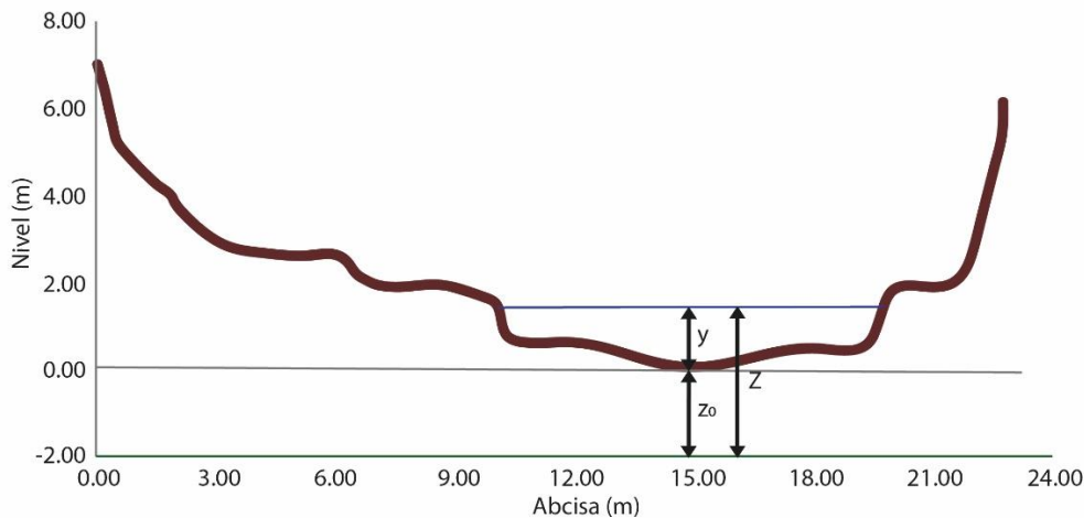
Figura 7. Sección transversal en función de la profundidad ( y ) y el nivel medido por el sensor ( Z )
