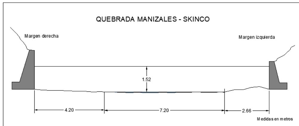
Figura 64. Sección transversal, Quebrada Manizales – Skinco, con medidas hechas en un cierto momento
