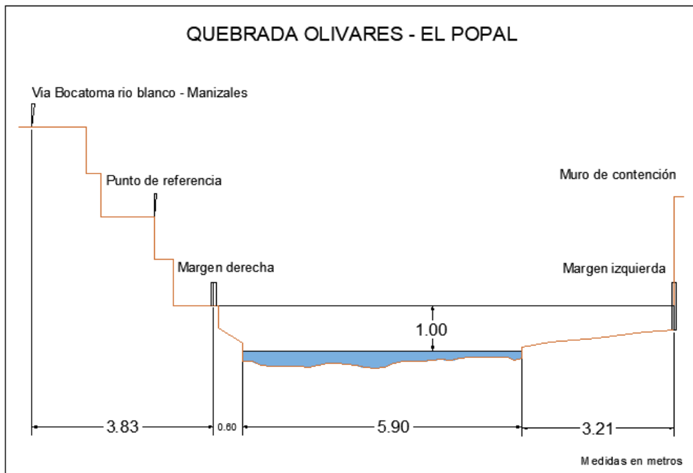
Figura 94. Sección transversal, Quebrada Olivares - El Popal, con medidas hechas en un cierto momento
