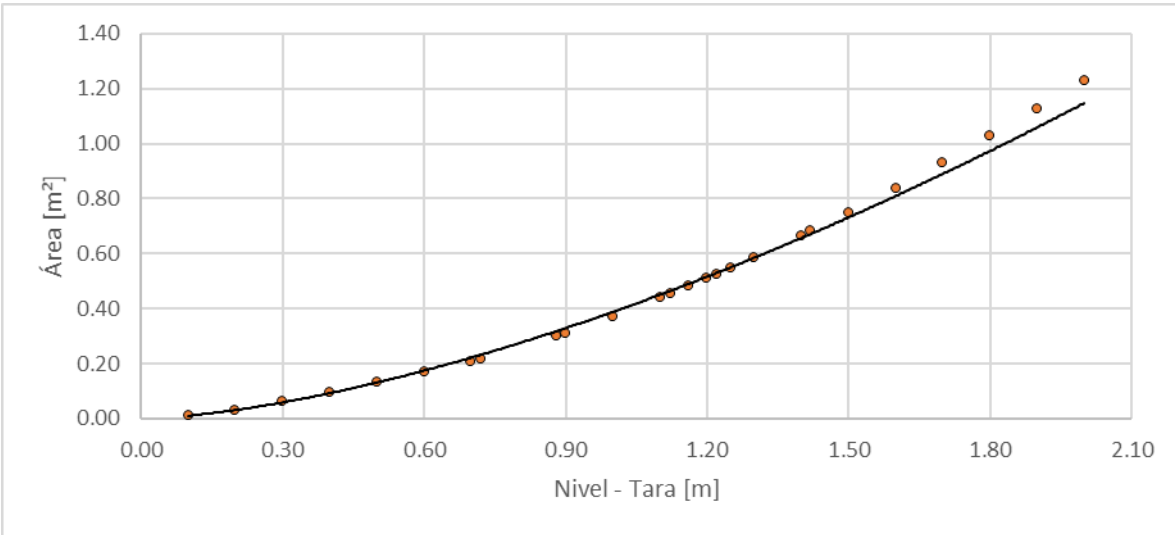
Figura 17. Nivel vs área, Quebrada El Bohío – Vereda El Águila
