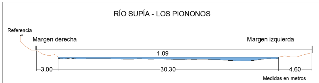
Figura 184. Sección transversal, Río Supía - Los Piononos, con medidas hechas en un cierto momento
