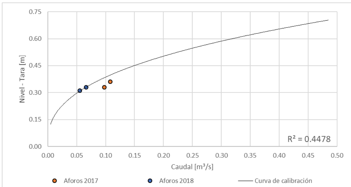
Figura 105. Curva nivel vs caudal, Quebrada Palogrande - Terminal de transportes
