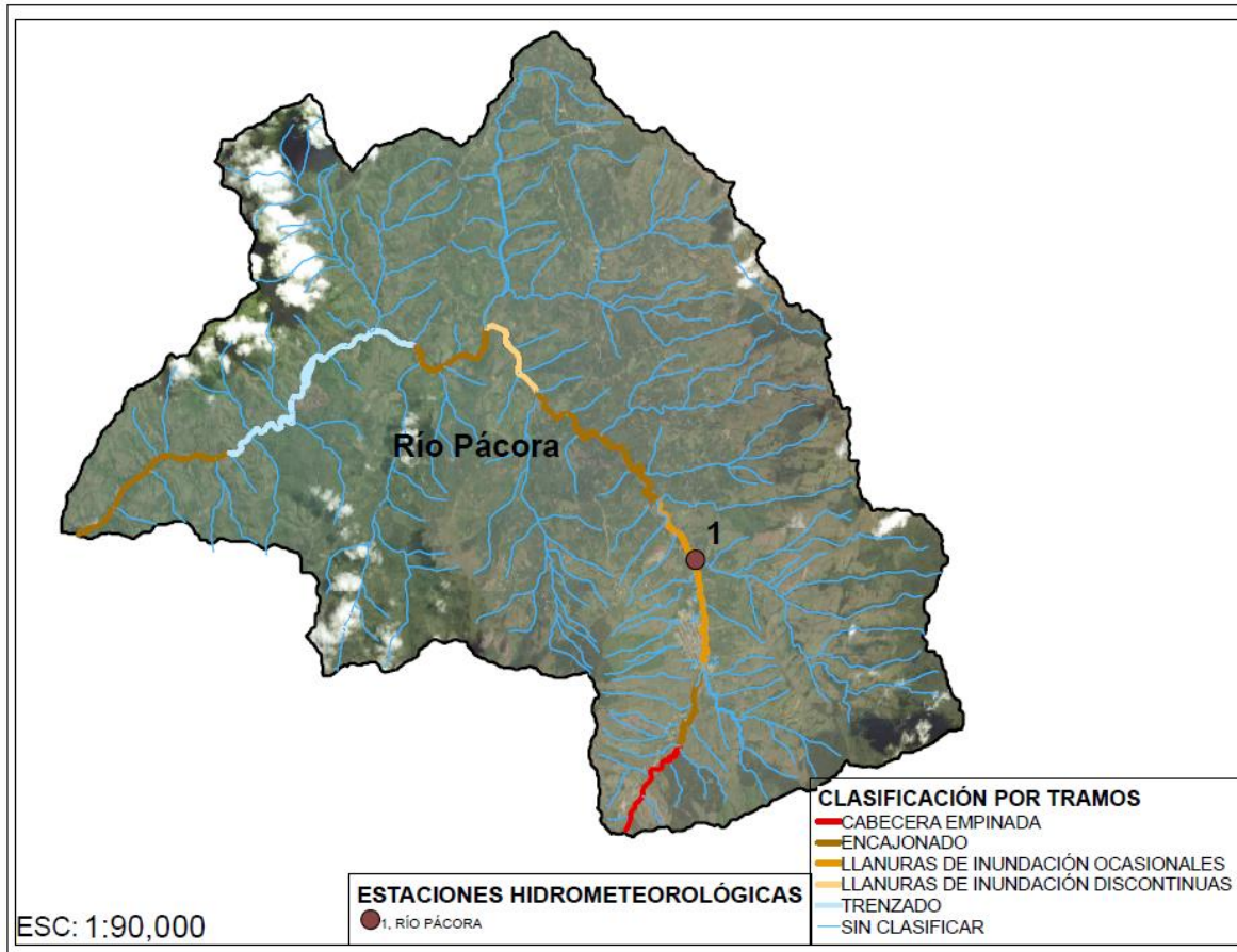
Figura 230. Clasificación cuenca del río Pácora
