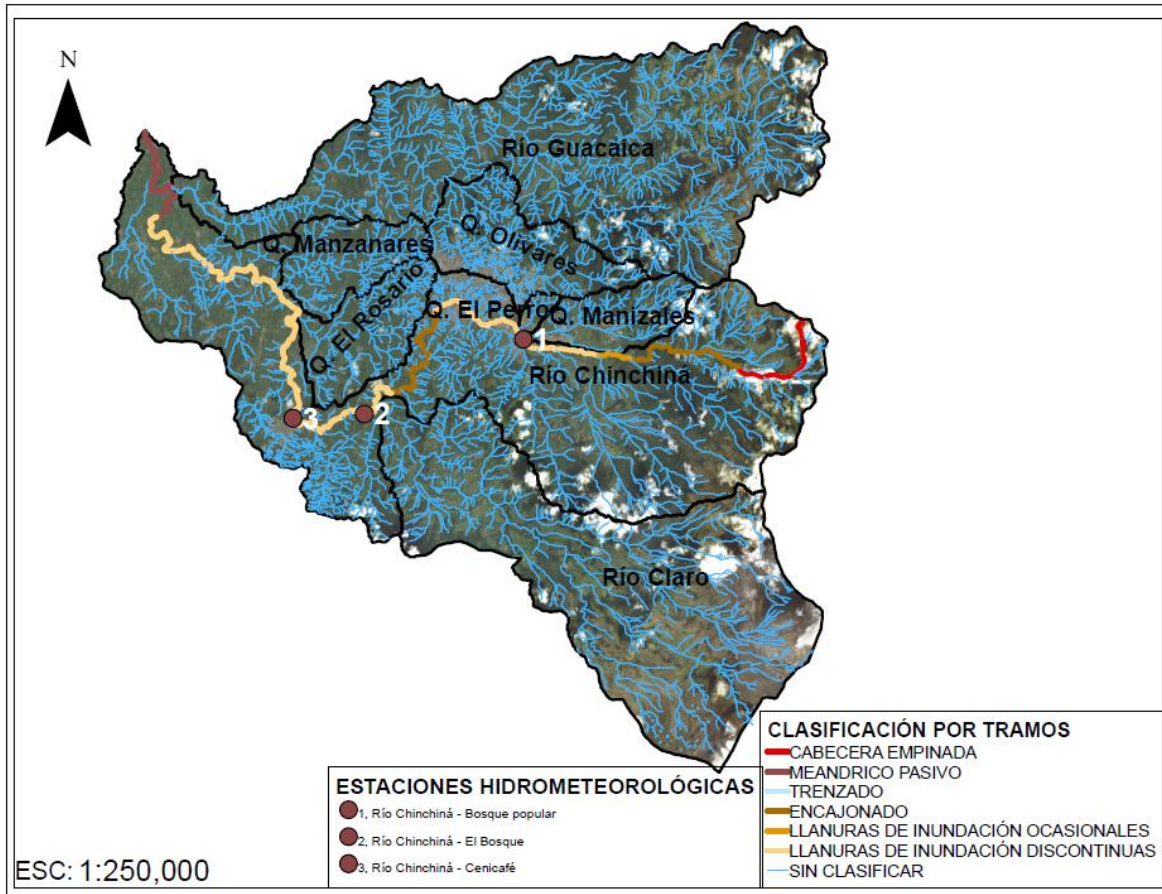
Figura 225. Clasificación cuenca del río Chinchiná
