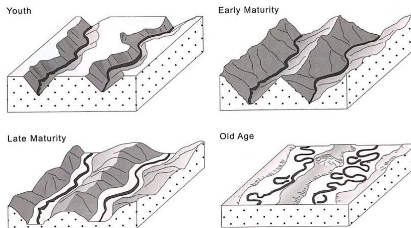
Figura 215. Clasificación de los ríos según su edad. (Fryirs & Brierley, 2013)
