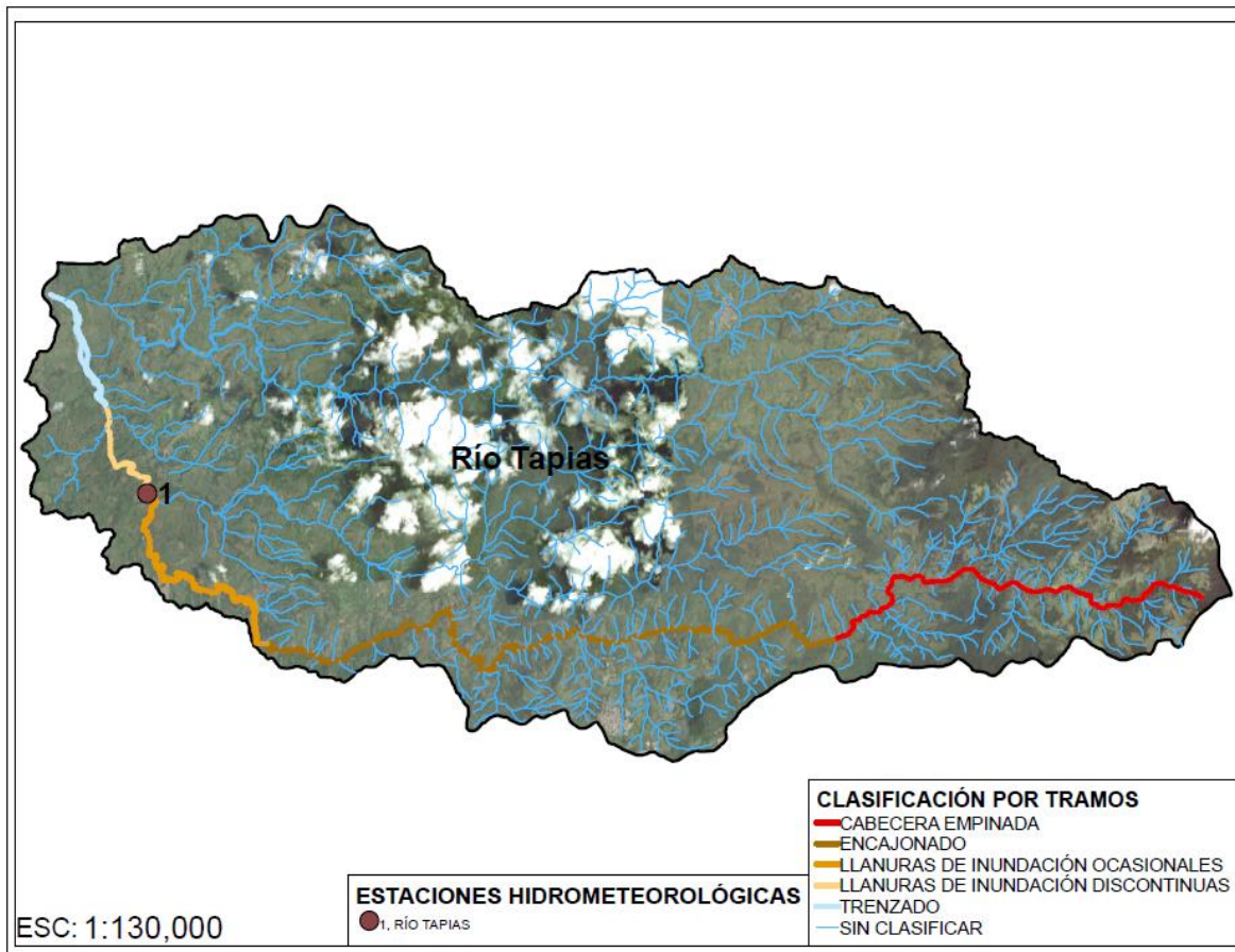
Figura 228. Clasificación cuenca del río Tapias
