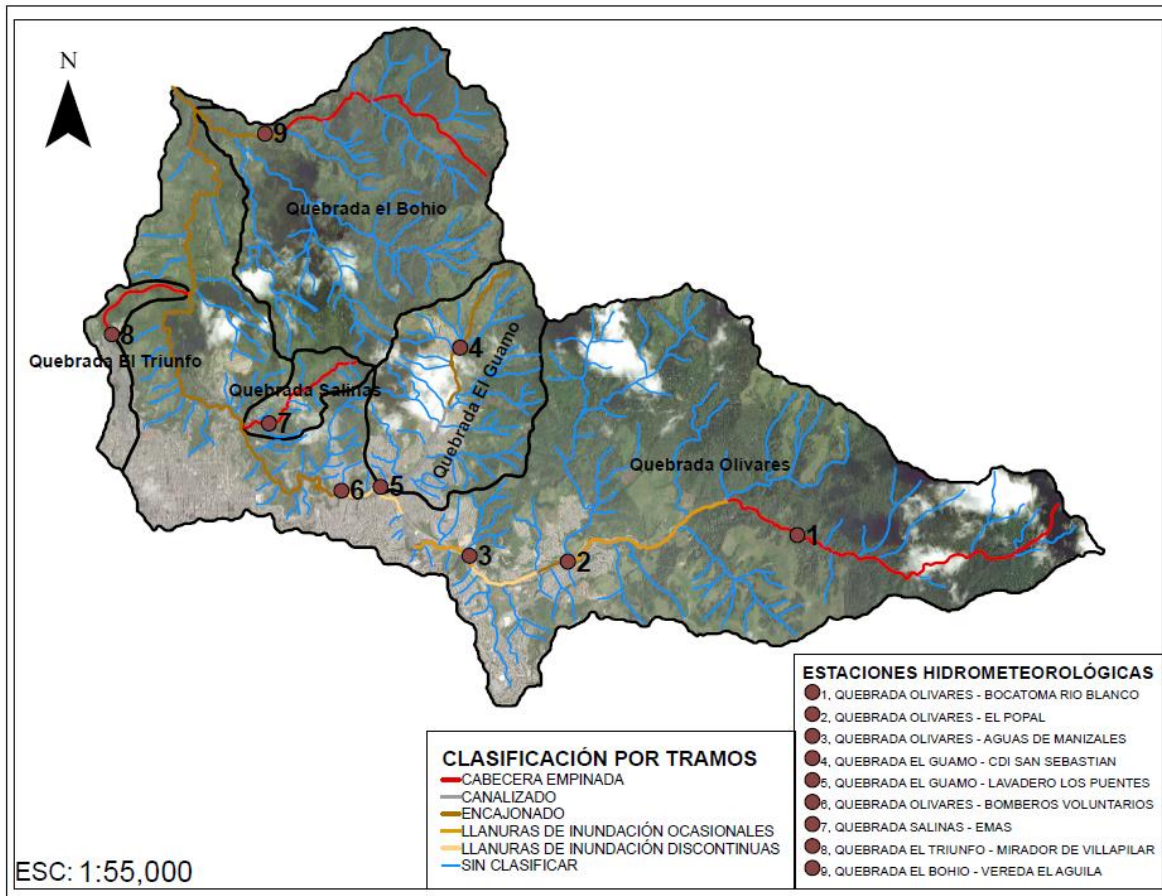
Figura 218. Clasificación cuenca de la quebrada Olivares
