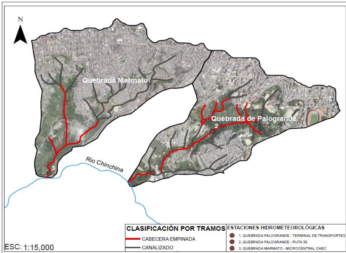
Figura 221. Clasificación cuencas de las quebradas Palogrande y Marmato
