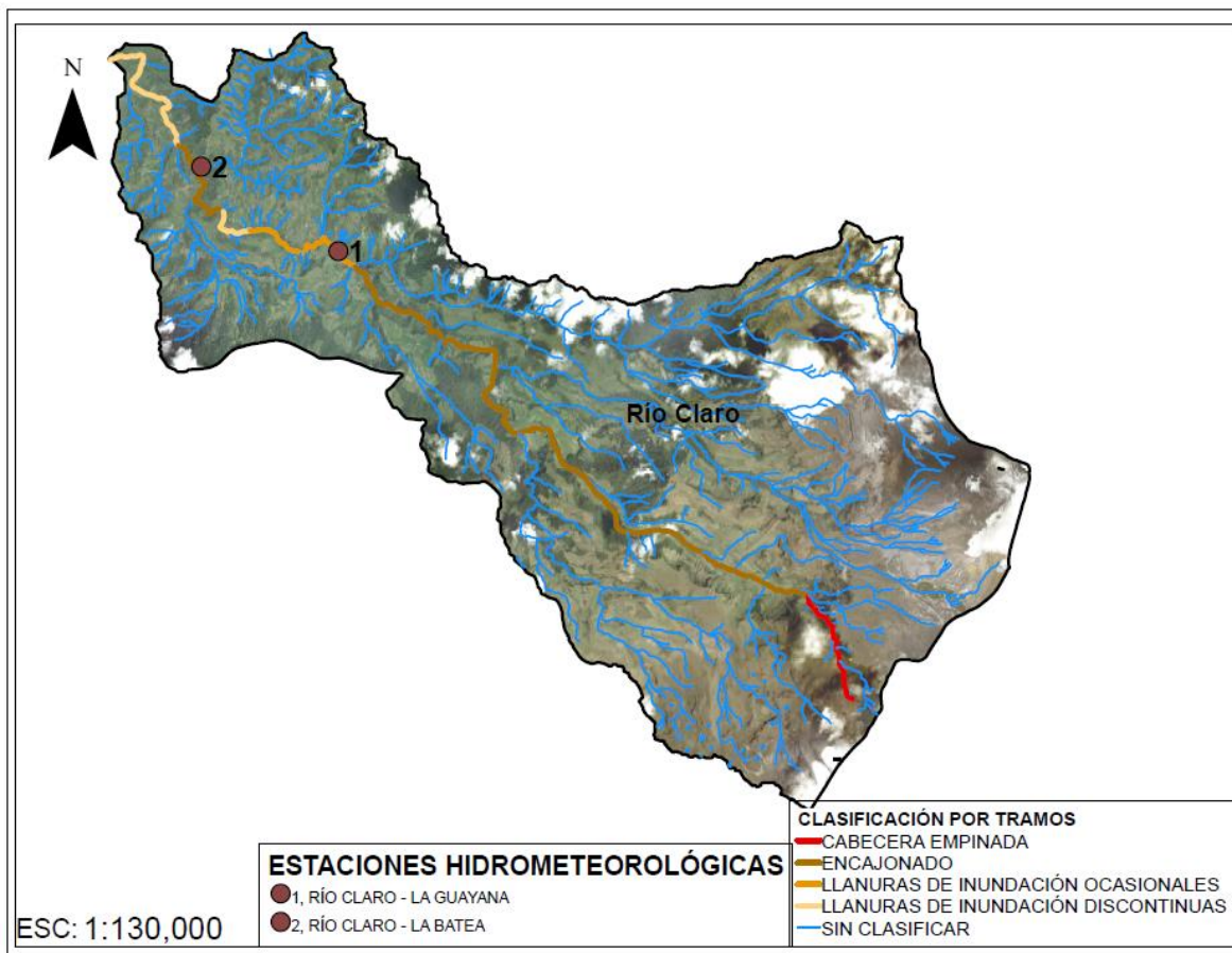
Figura 222. Clasificación cuenca del río Rioclaro
