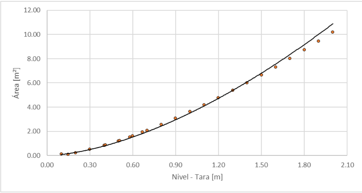
Figura 42. Nivel vs área, Quebrada El Rosario - San Marcos de León
