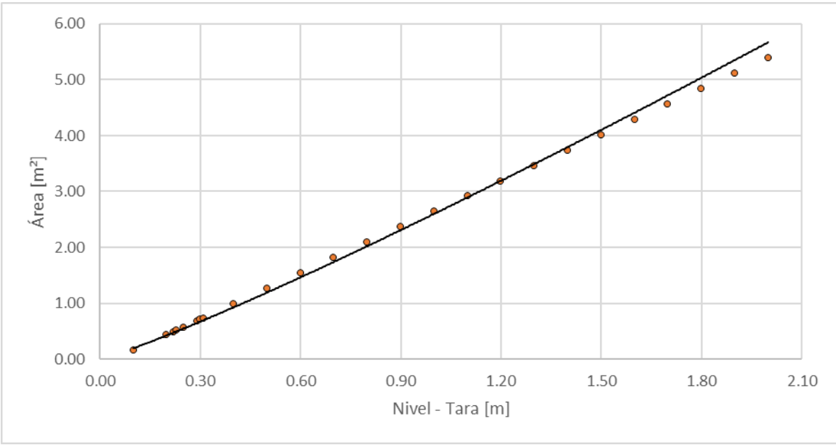
Figura 62. Nivel vs área, Quebrada Las Pavas - Autopistas del Café
