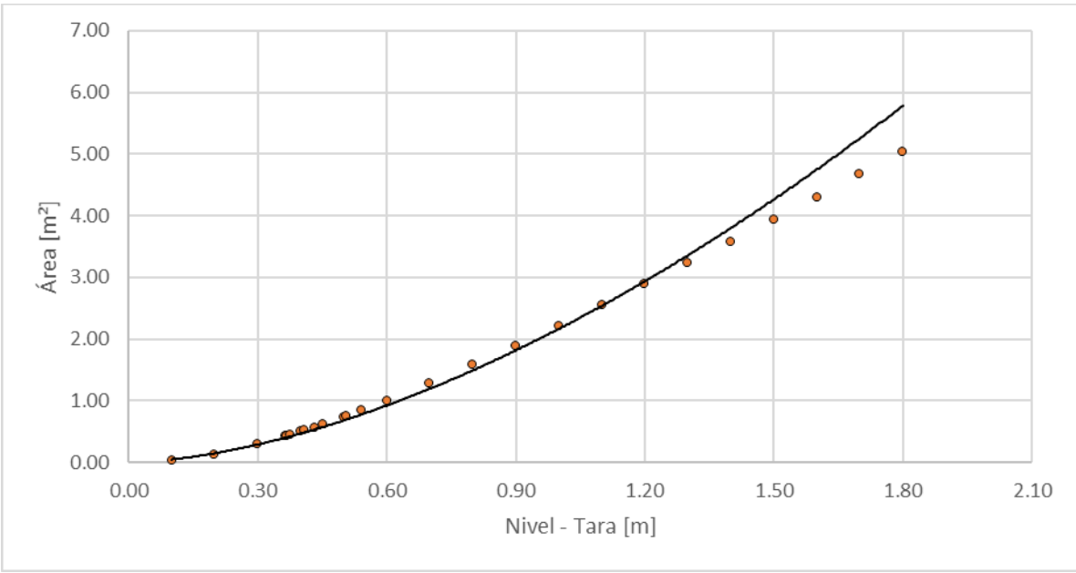
Figura 52. Nivel vs área, Quebrada Guayabal - Recinto del pensamiento
