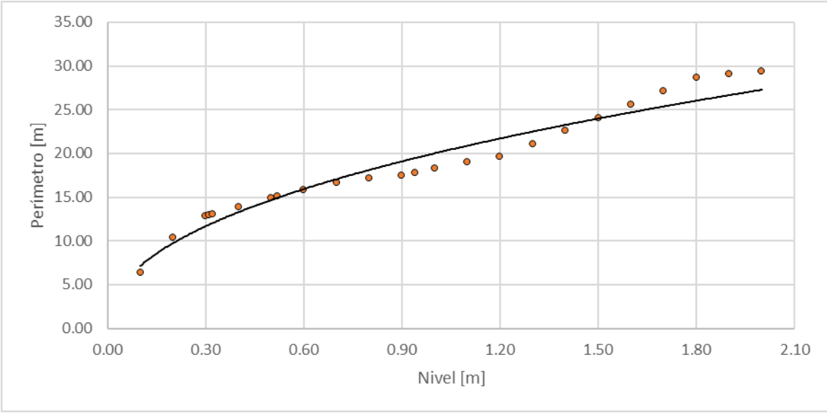
Figura 151. Nivel vs perímetro, Río Pácora
