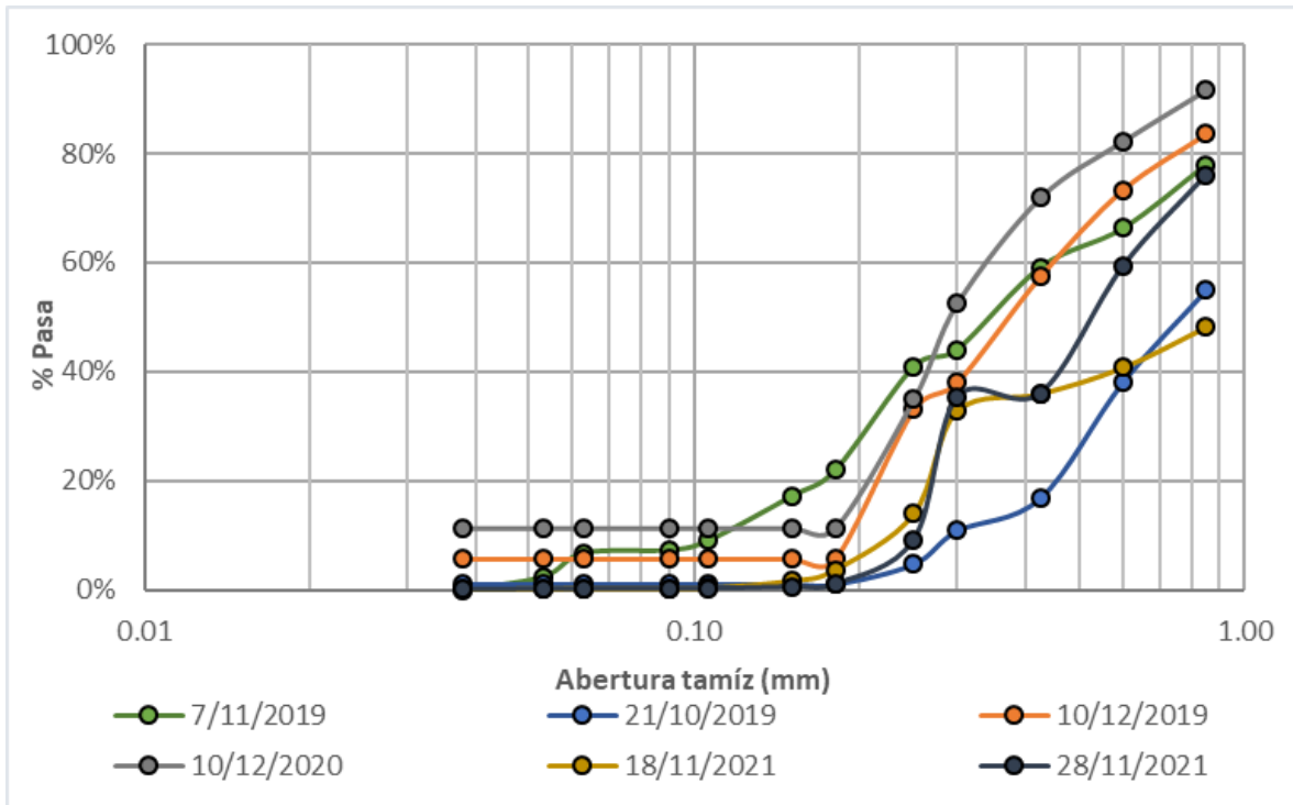
Figura 210. Granulometría sedimentos de fondo, Río Chinchiná - Cenicafé
