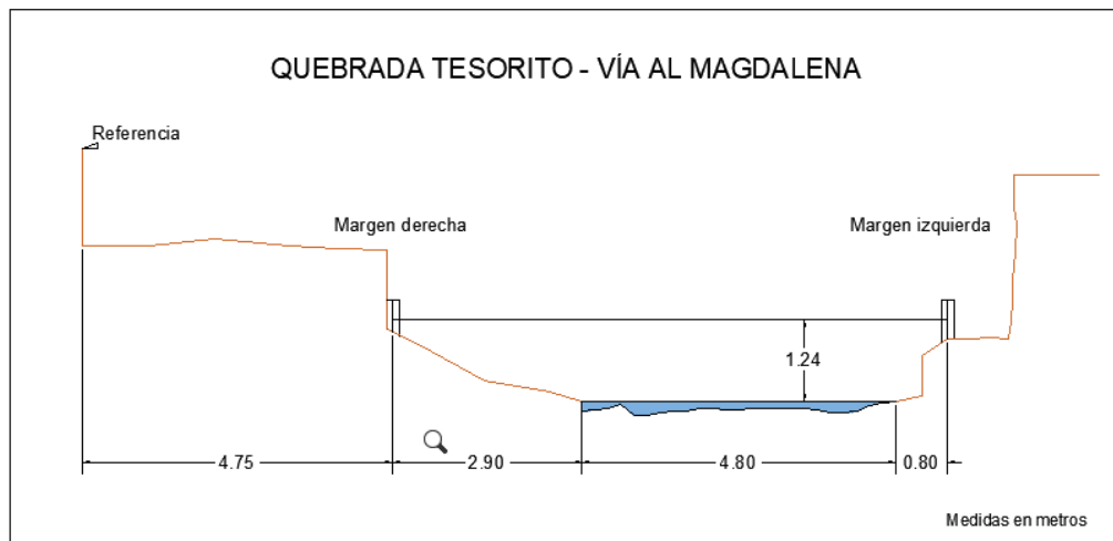
Figura 114. Sección transversal, Quebrada Tesorito – Vía al Magdalena, con medidas hechas en un cierto momento
