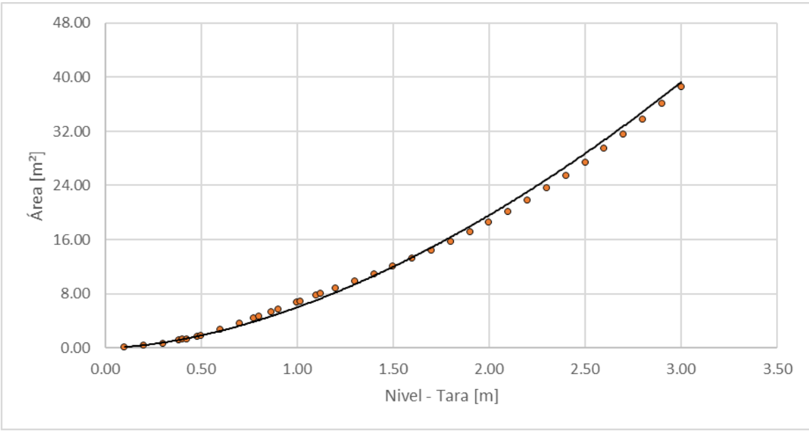
Figura 122. Nivel vs área, Río Chinchiná - Bosque Popular
