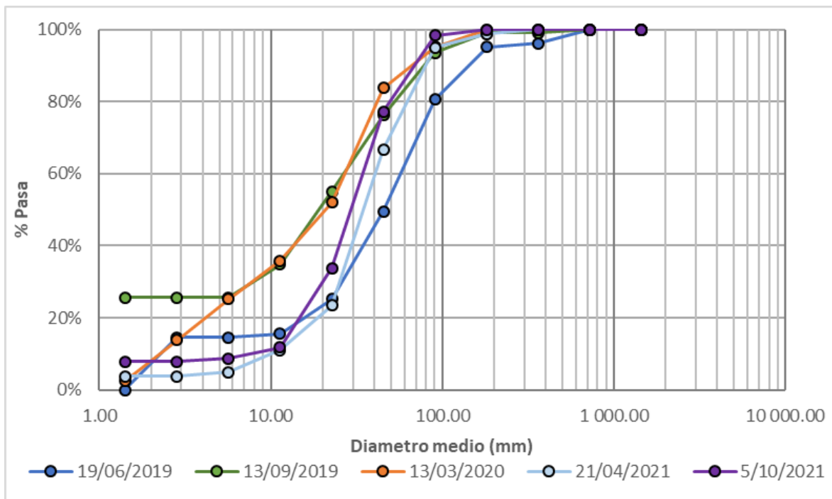
Figura 206. Granulometría material del lecho (conteo de Wolman), Quebrada Olivares – El Popal
