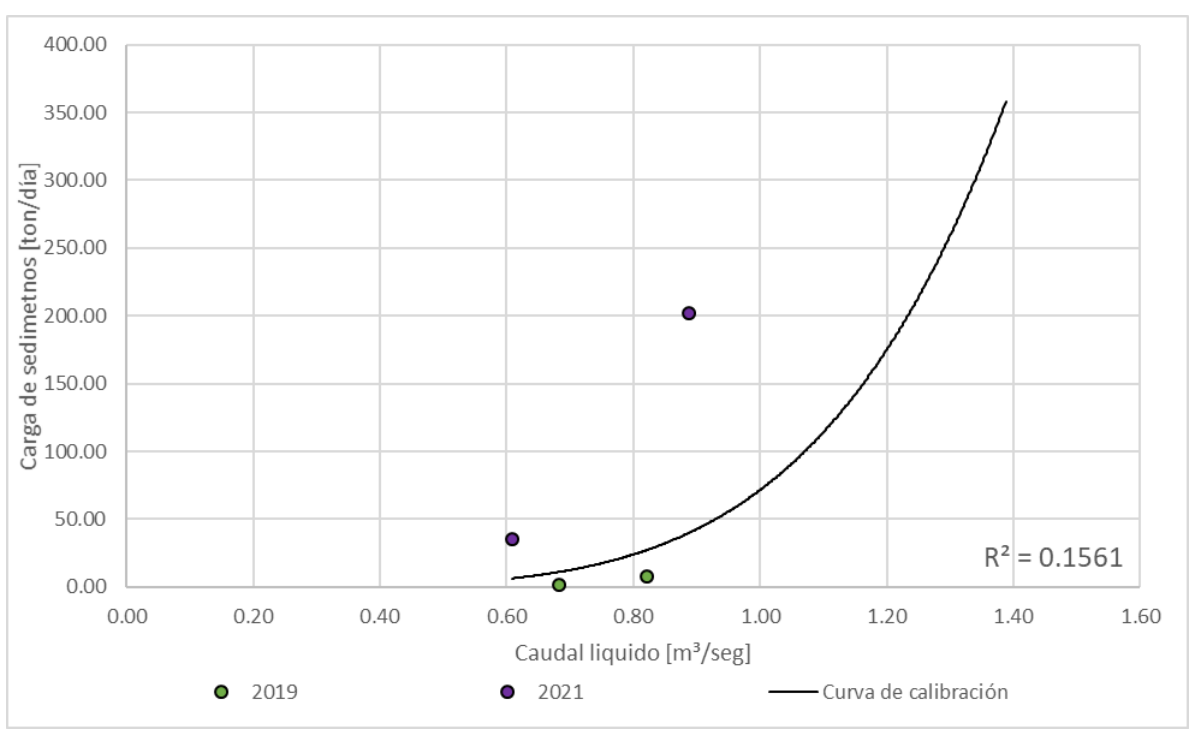
Figura 198. Relación caudal líquido – caudal sólido, Quebrada El Rosario - Autopistas
