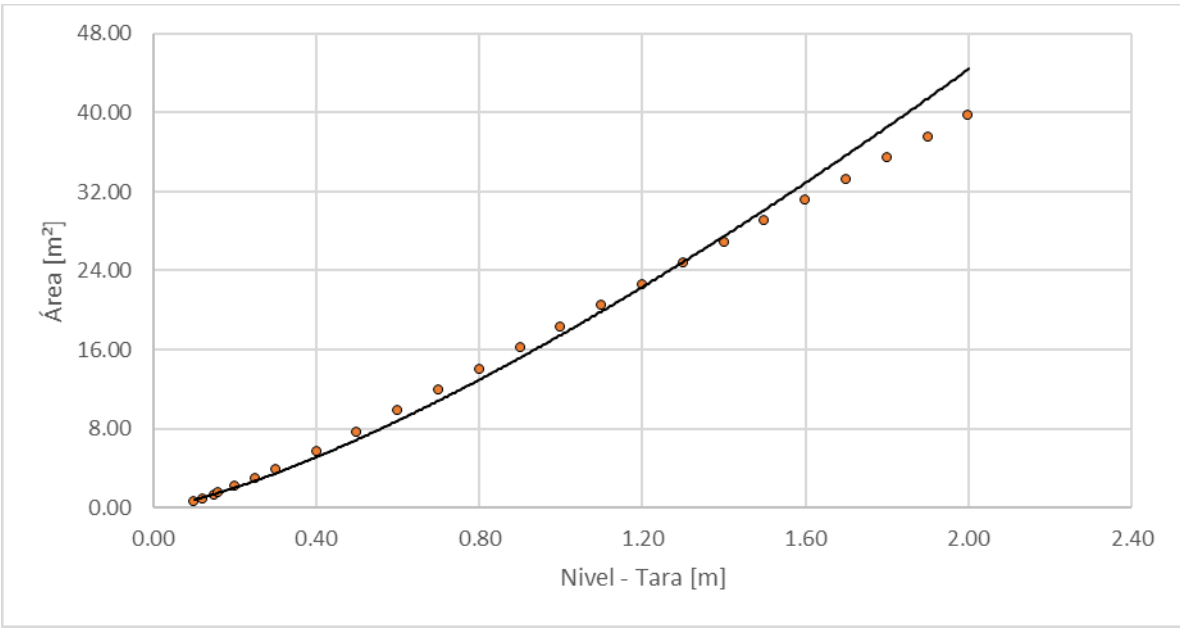
Figura 82. Nivel vs área, Quebrada Olivares - Aguas de Manizales
