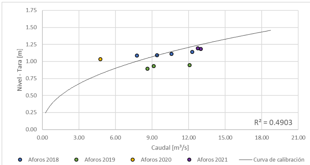
Figura 130. Curva nivel vs caudal, Río Chinchiná - El Bosque
