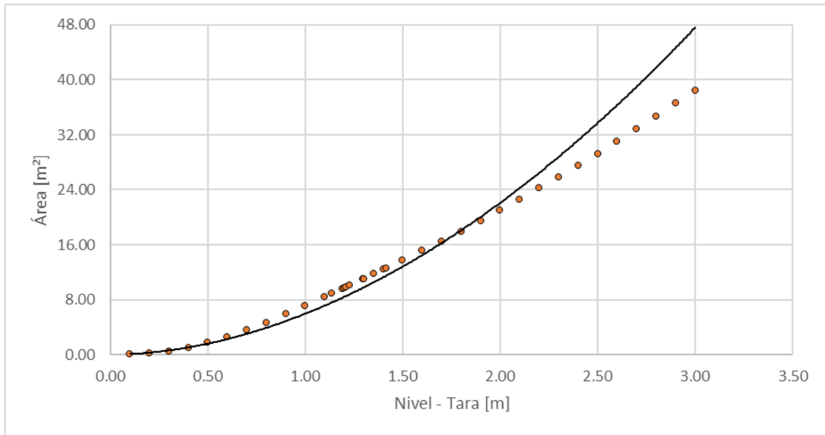
Figura 147. Nivel vs área, río Guacaica - El Jordán
