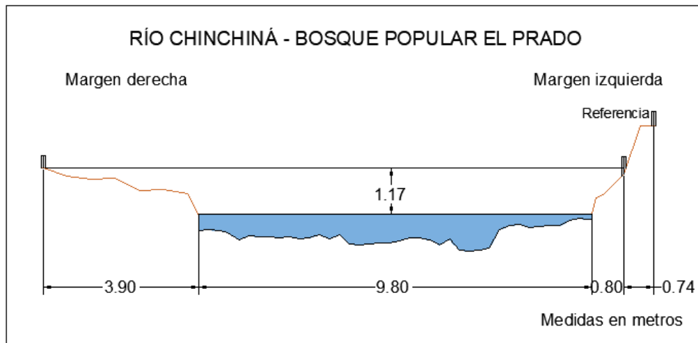
Figura 119. Sección transversal, Río Chinchiná - Bosque Popular, con medidas hechas en un cierto momento
