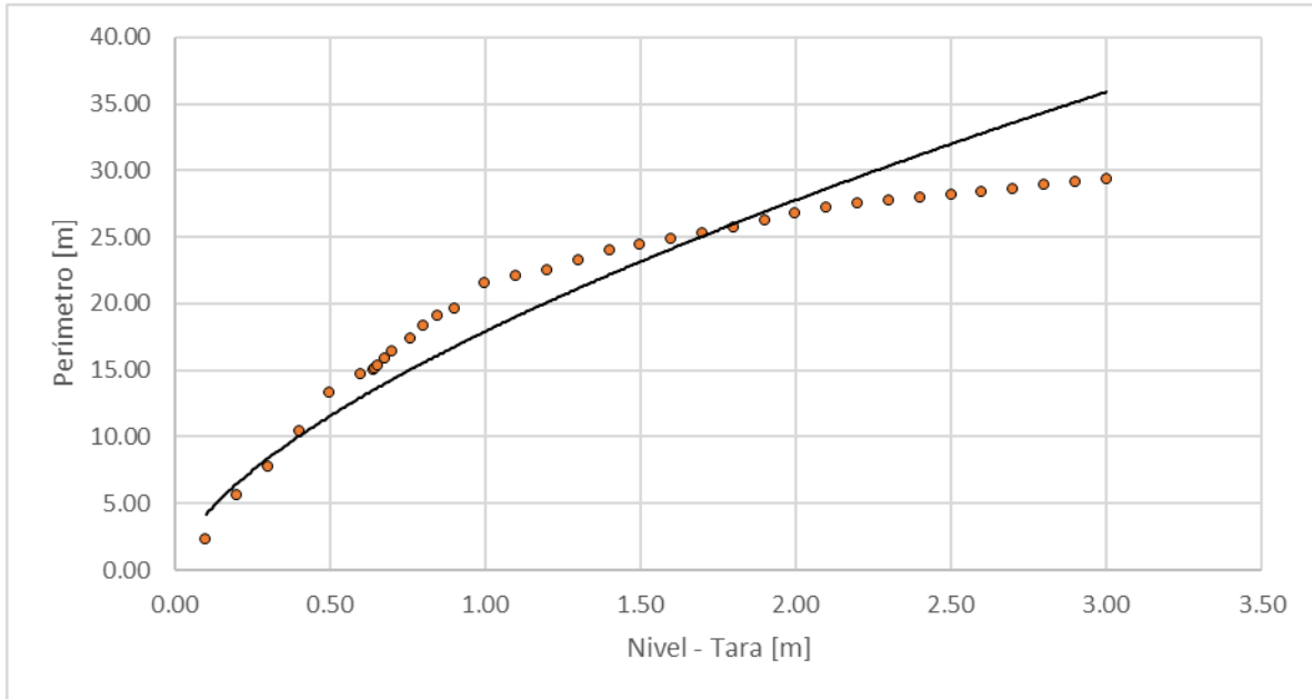
Figura 161. Nivel vs perímetro, Río Pozo – Vía La Merced Pácora
