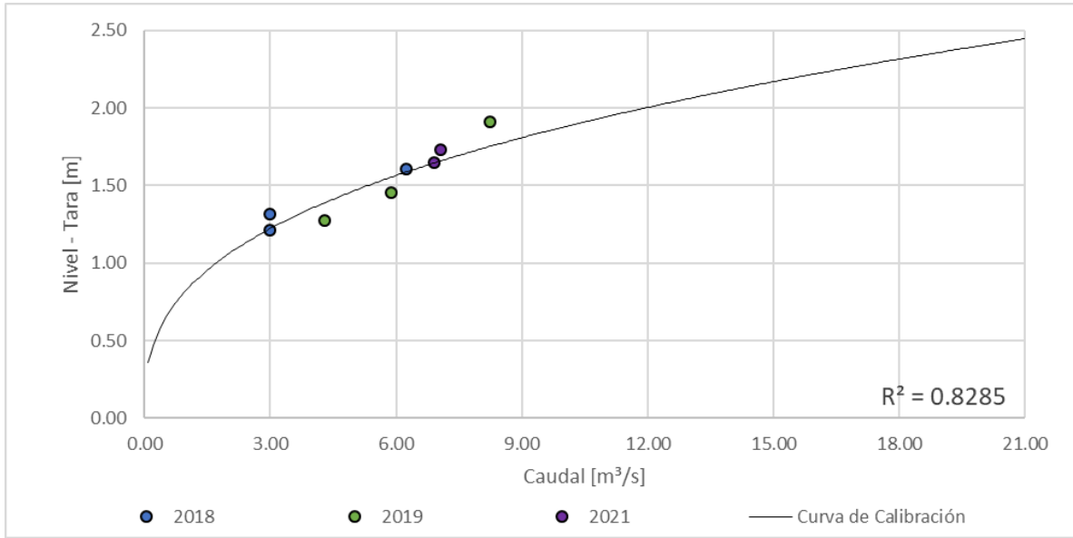
Figura 185. Curva nivel vs caudal, Río Supía - Los Piononos
