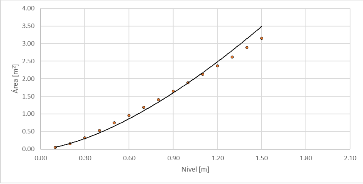
Figura 37. Nivel vs área, Quebrada el Rosario - Autopistas
