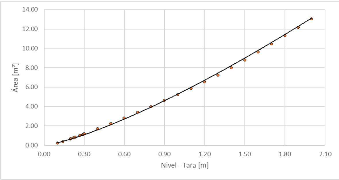
Figura 117. Nivel vs área, Quebrada Tesorito – Vía al Magdalena
