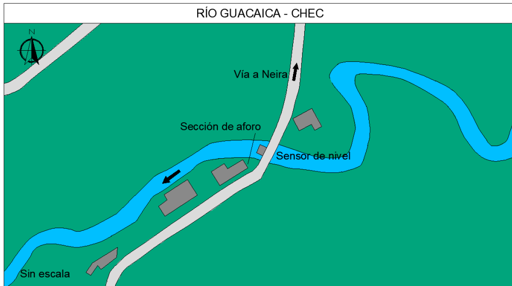
Figura 138. Vista en planta, Río Guacaica - CHEC
