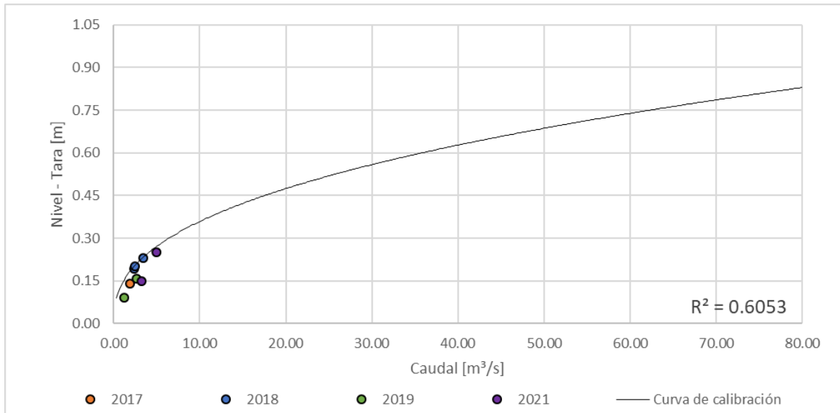
Figura 180. Curva nivel vs caudal, Río Santo Domingo - Manzanares
