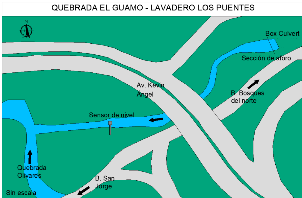
Figura 23. Vista en planta, Quebrada el Guamo - Lavadero Los Puentes
