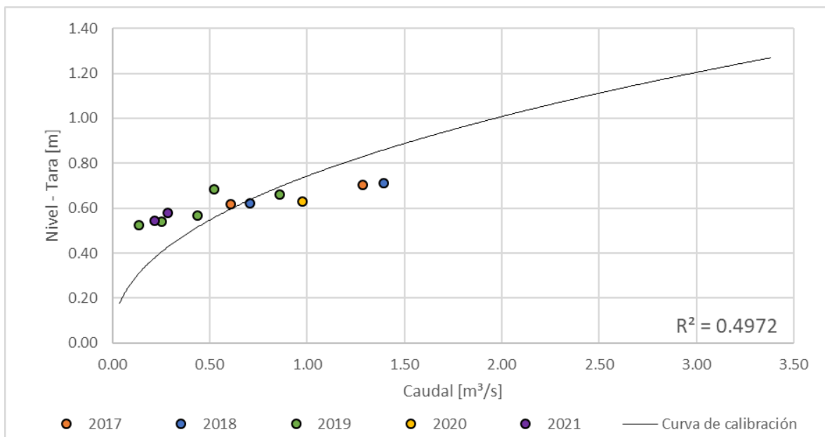
Figura 95. Curva nivel vs caudal, Quebrada Olivares - El Popal
