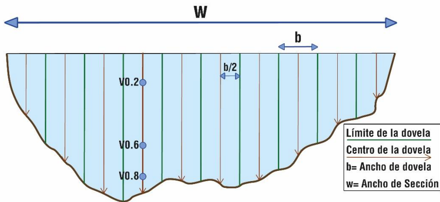
Figura 6. Sección típica de aforo, profundidades medidas desde la superficie
