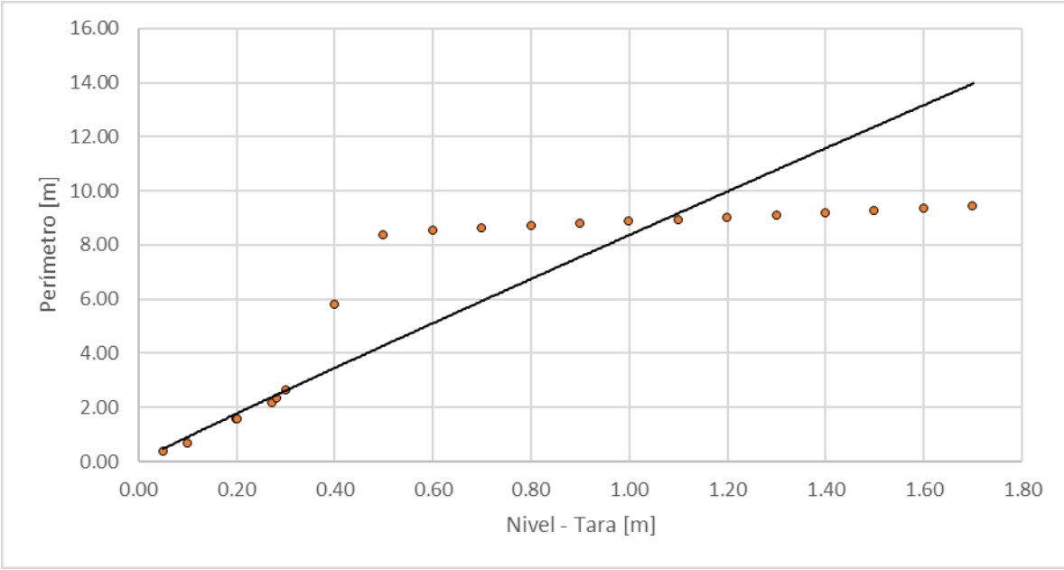
Figura 31. Nivel vs perímetro, Quebrada El Perro – Expoferias
