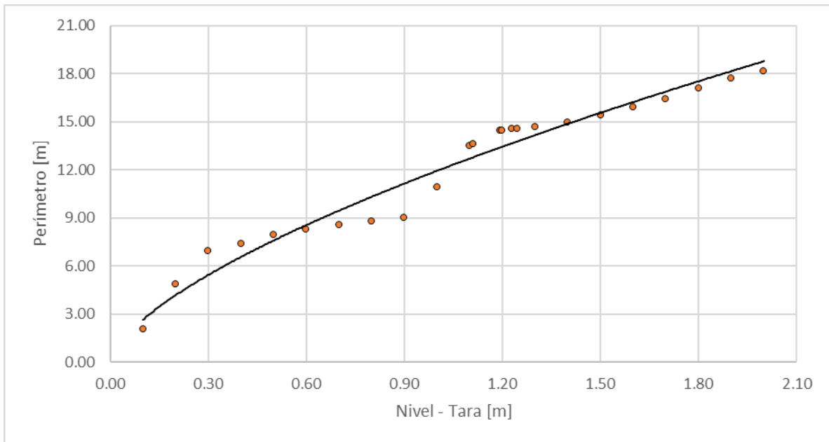
Figura 171. Nivel vs perímetro, Río Rioclaro - La Guayana
