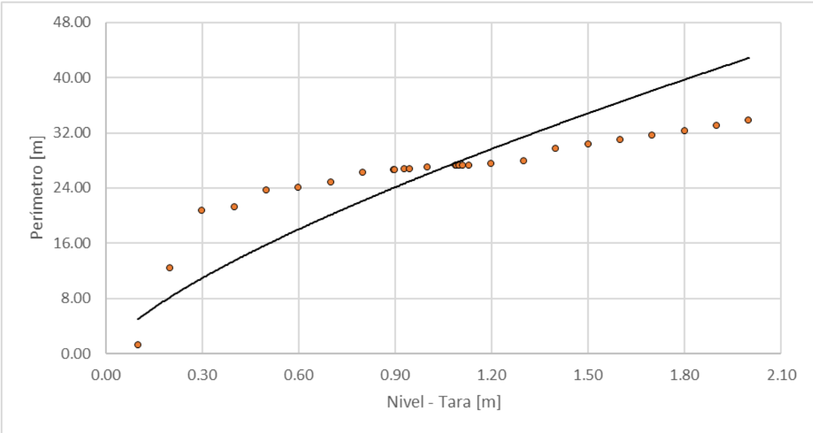
Figura 131. Nivel vs Perímetro, Río Chinchiná - El Bosque
