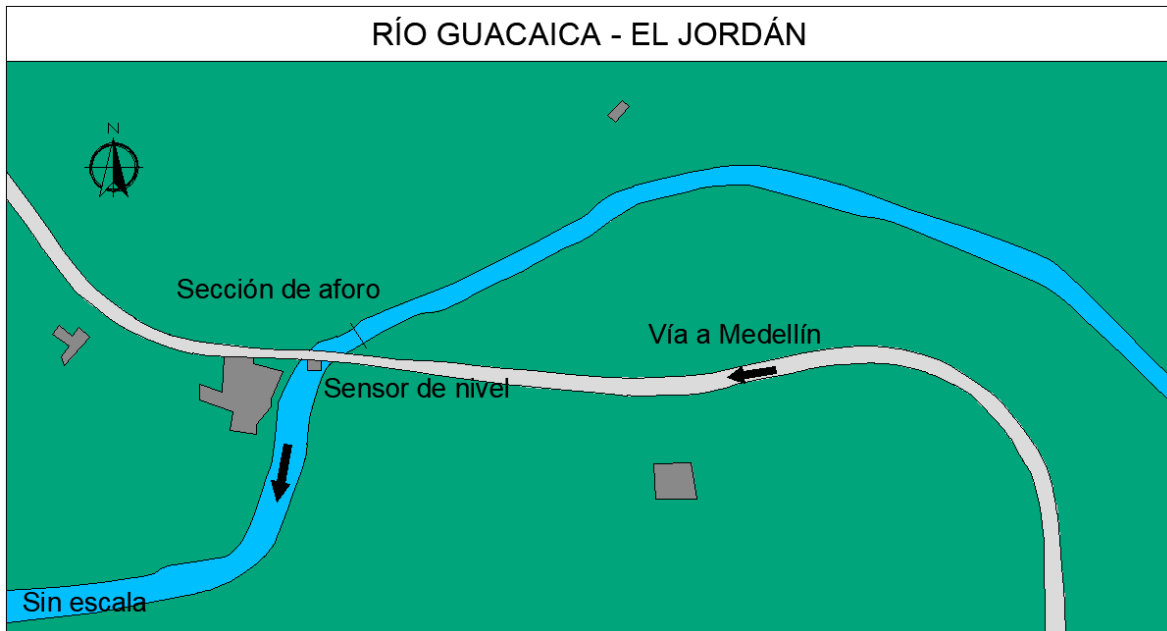
Figura 143. Vista en planta, Río Guacaica - El Jordán
