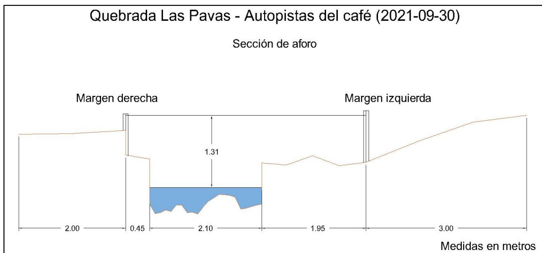
Figura 59. Sección transversal, Quebrada Las Pavas - Autopistas del Café, con medidas hechas en un cierto momento
