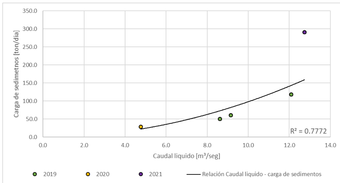
Figura 212. Relación caudal líquido - caudal sólido, Río Chinchiná - El Bosque
