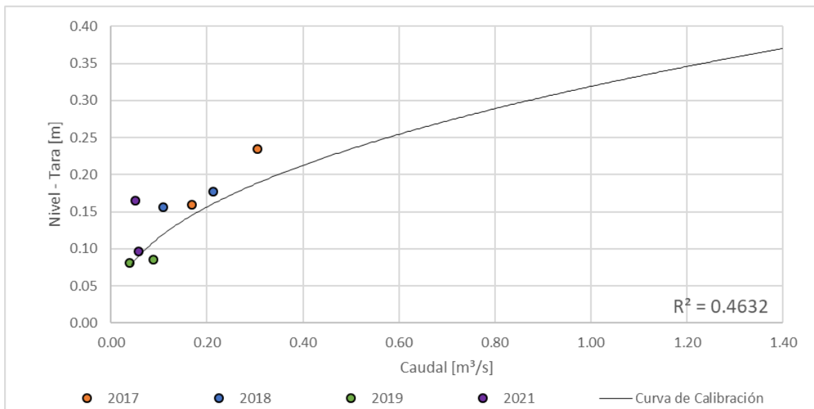
Figura 55. Curva nivel vs caudal, Quebrada La Francia - Los Puentes
