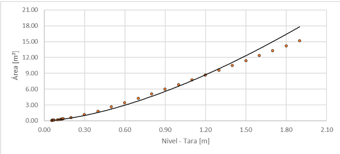
Figura 22. Nivel vs área, Quebrada el Guamo - CDI San Sebastián
