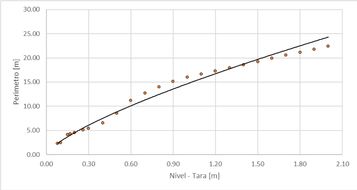
Figura 56. Nivel vs perímetro, Quebrada La Francia - Los Puentes
