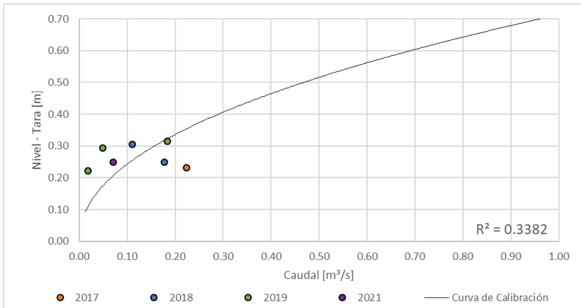
Figura 60. Curva nivel vs caudal, Quebrada Las Pavas - Autopistas del Café
