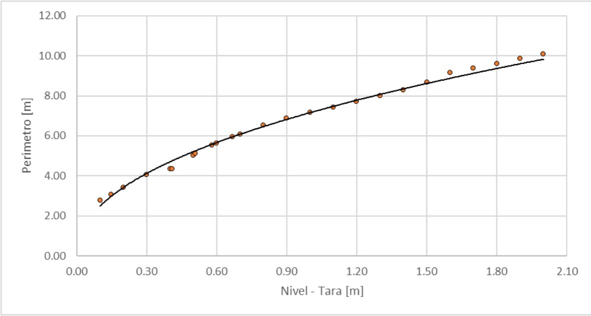
Figura 41. Nivel vs perímetro, Quebrada El Rosario - San Marcos de León
