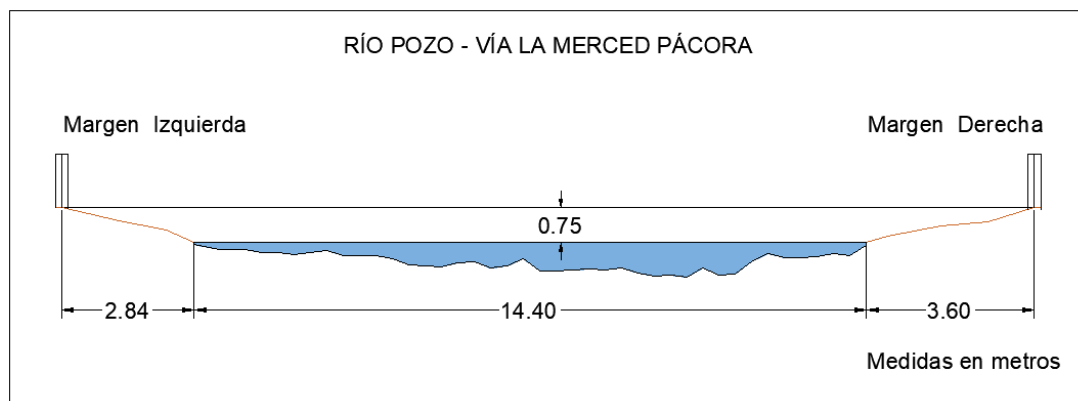
Figura 159. Sección transversal, Río Pozo – Vía La Merced Pácora, con medidas hechas en un cierto momento
