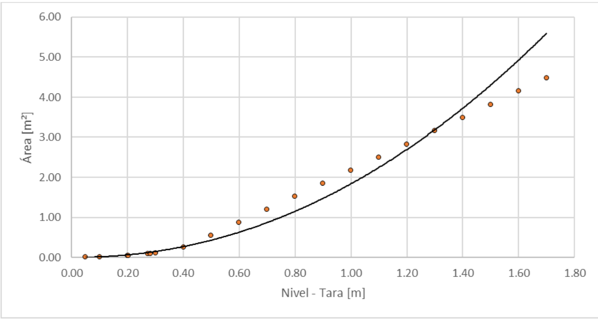
Figura 32. Nivel vs área, Quebrada El Perro – Expoferias
