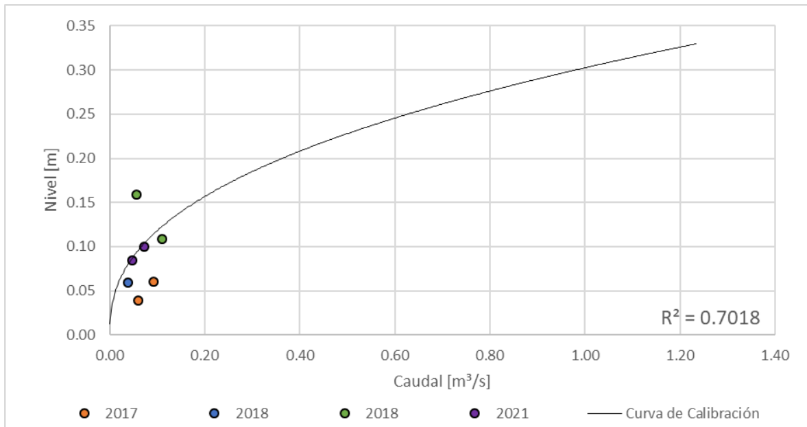
Figura 45. Curva nivel vs caudal, Quebrada el Triunfo - Mirador de Villapilar
