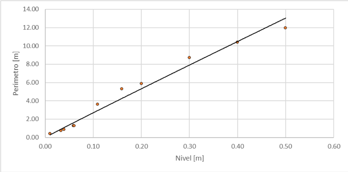
Figura 46. Nivel vs perímetro, Quebrada El Triunfo - Mirador de Villapilar
