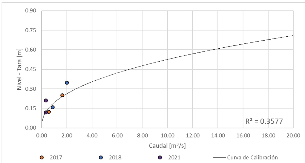
Figura 80. Curva nivel vs caudal, Quebrada Olivares - Aguas de Manizales
