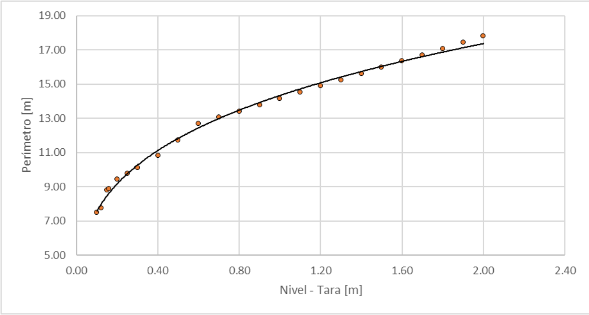
Figura 81. Nivel vs perímetro, Quebrada Olivares - Aguas de Manizales
