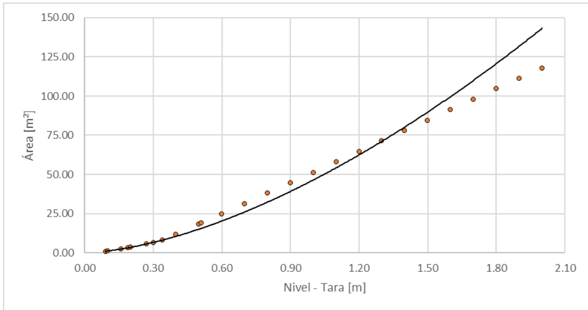
Figura 182. Nivel vs área, Río Santo Domingo - Manzanares
