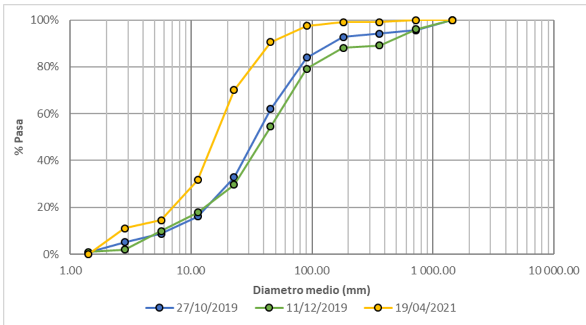
Figura 200. Granulometría material del lecho (conteo de Wolman), Quebrada El Rosario - Autopistas
