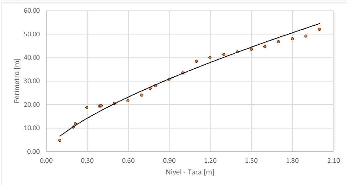
Figura 191. Nivel vs perímetro, Río Supía – Supía
