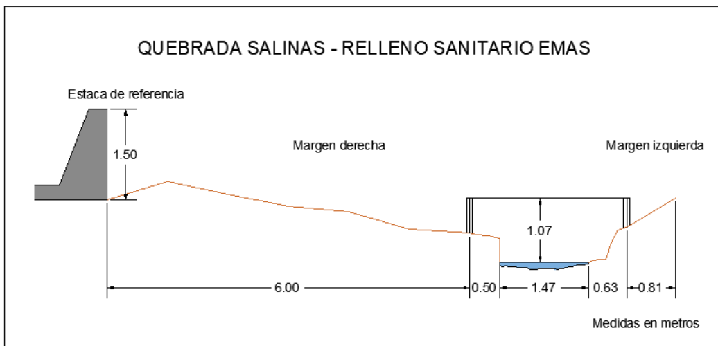
Figura 109. Sección transversal, Quebrada Salinas - Relleno sanitario EMAS, con medidas hechas en un cierto momento
