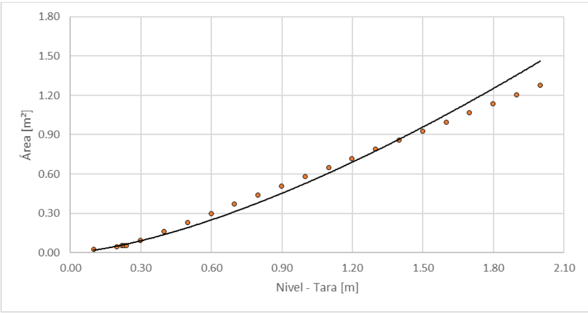
Figura 107. Nivel vs área, Quebrada Palogrande - Terminal de transportes
