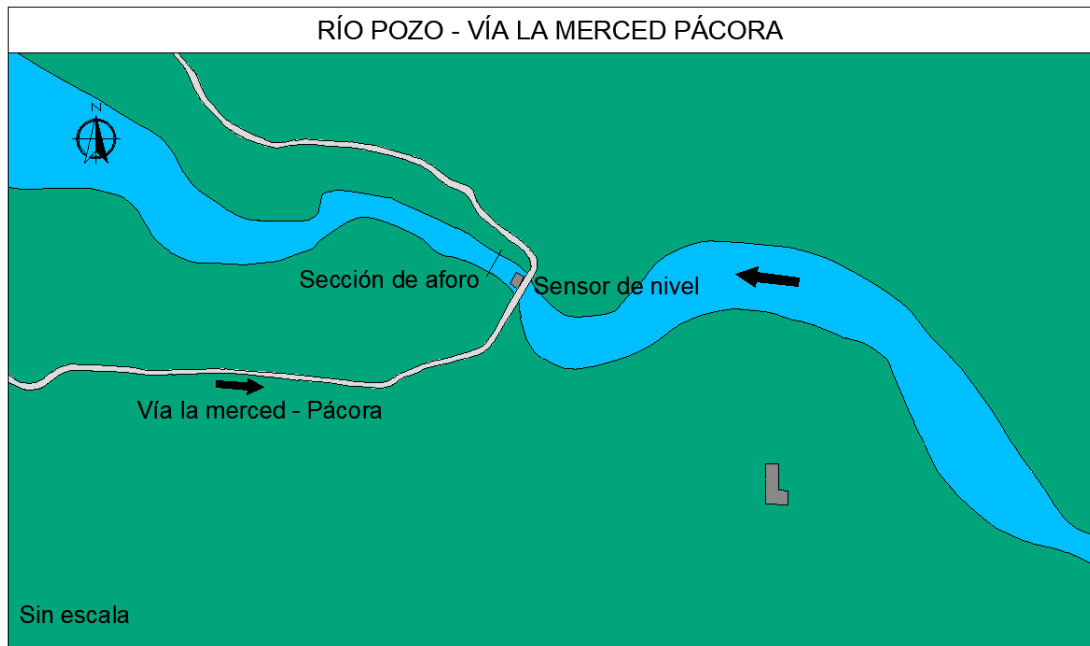
Figura 158. Vista en planta, Río Pozo - Vía La Merced Pácora
