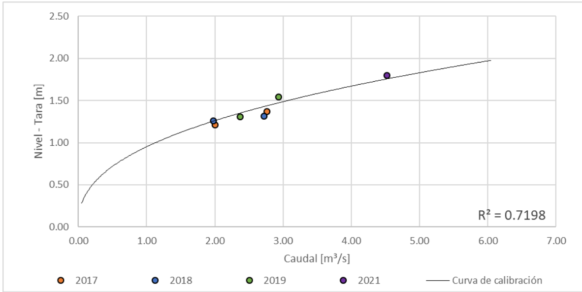
Figura 155. Curva nivel vs caudal, Río Pensilvania – Microcentral
