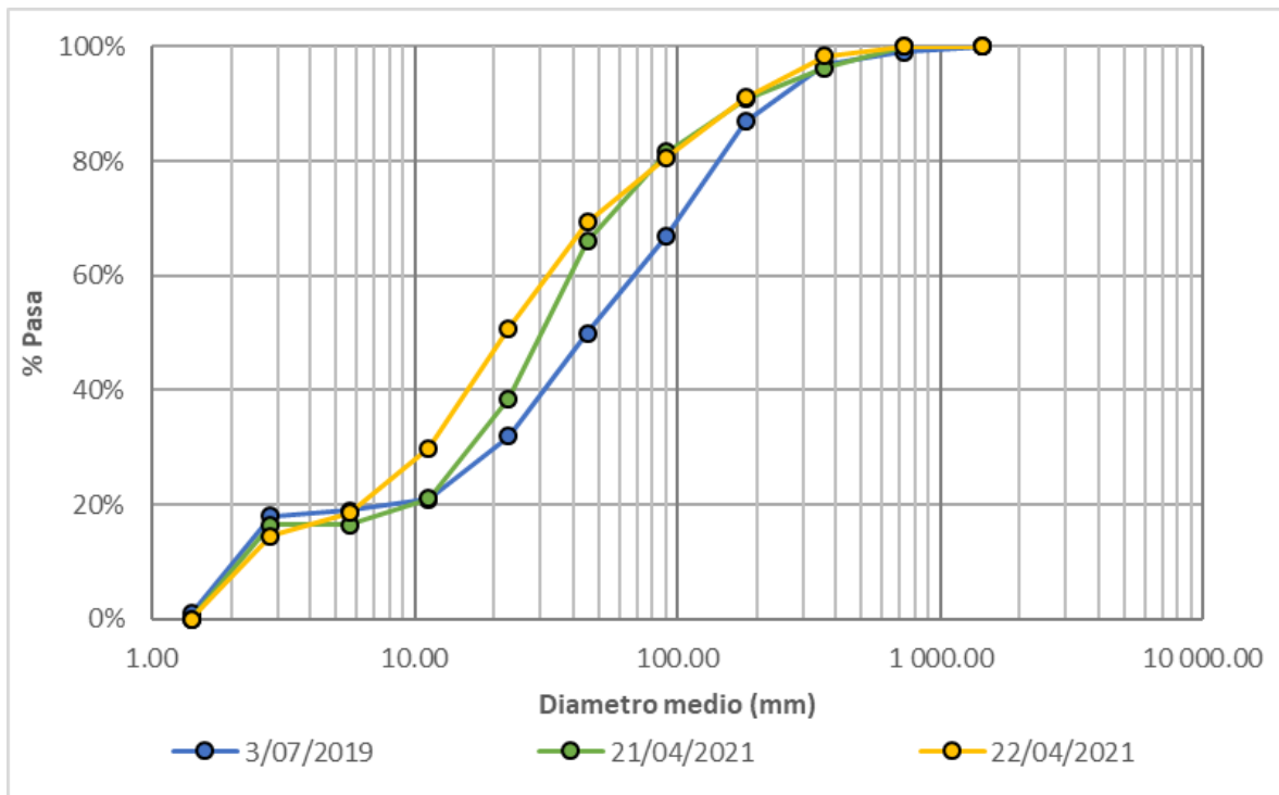
Figura 208. Granulometría material del lecho (conteo de Wolman), Quebrada Salinas – Relleno sanitario EMAS
