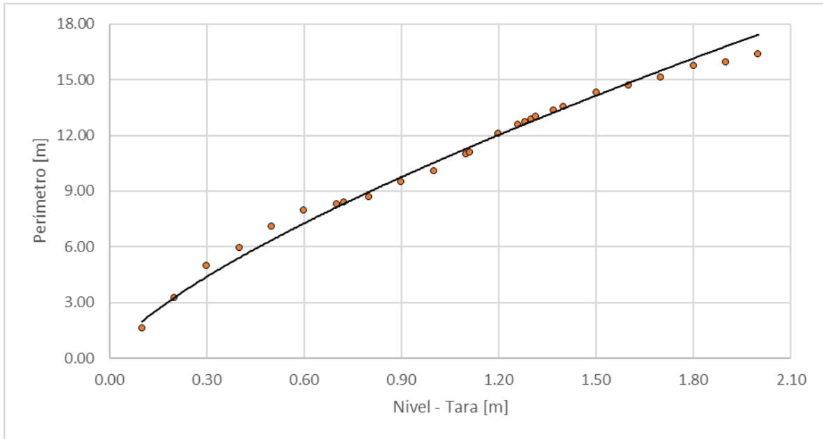
Figura 156. Nivel vs Perímetro, Río Pensilvania - Microcentral
