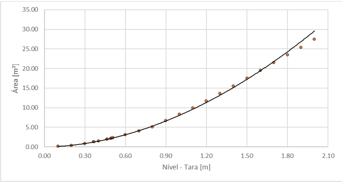
Figura 77. Nivel vs área, Quebrada Marmato - Planta Intermedia CHEC
