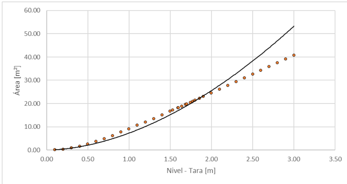
Figura 177. Nivel vs área, Río Risaralda - Camping La Palmera
