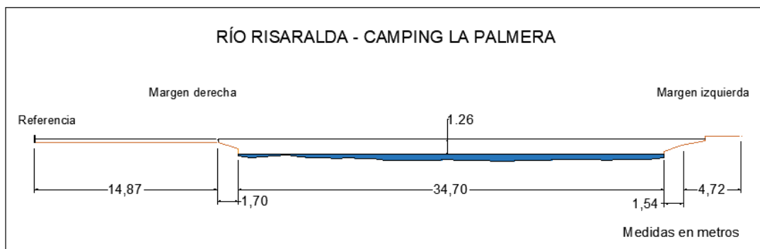
Figura 174. Sección transversal, Río Risaralda - Camping La Palmera, con medidas hechas en un cierto momento
