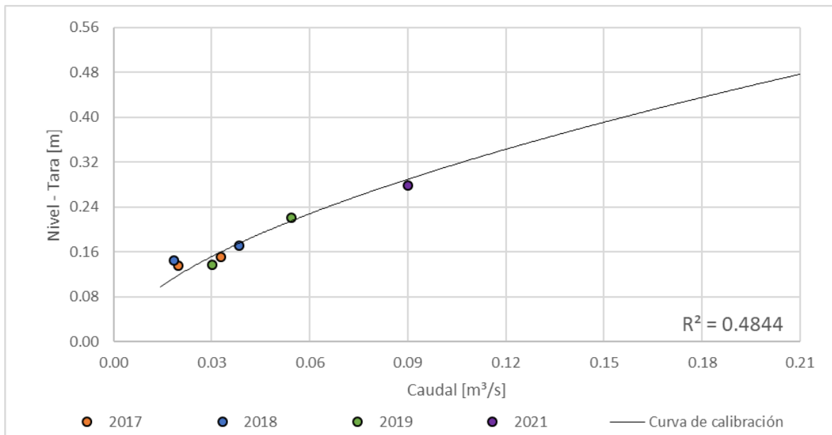
Figura 110. Curva nivel vs caudal, Quebrada Salinas - Relleno sanitario EMAS
