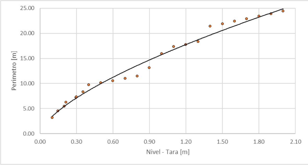
Figura 71. Nivel vs perímetro, Quebrada Manzanares - Industrias Básicas de Caldas
