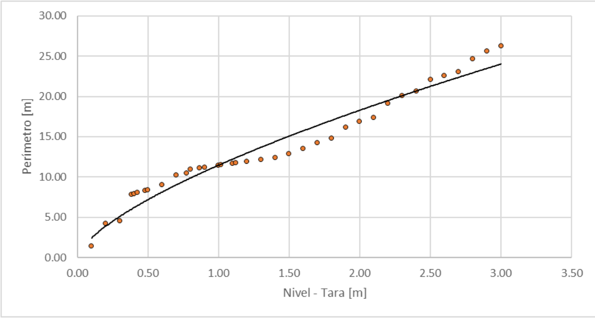
Figura 121. Nivel vs perímetro, Río Chinchiná - Bosque Popular
