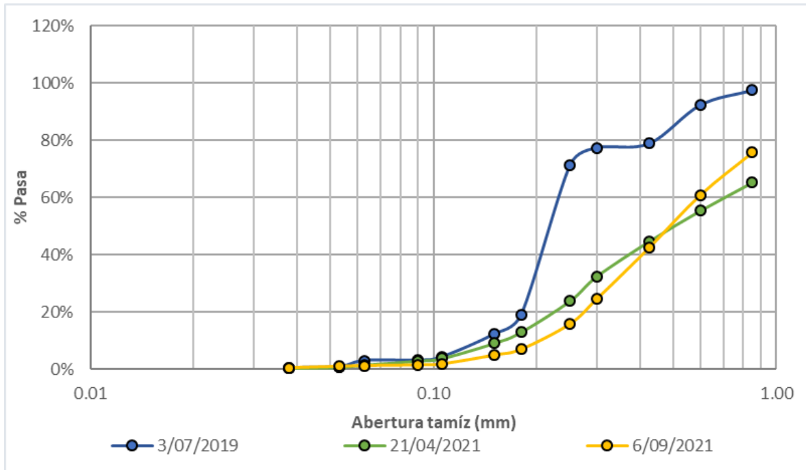
Figura 207. Granulometría sedimentos de fondo, Quebrada Salinas – Relleno sanitario EMAS
