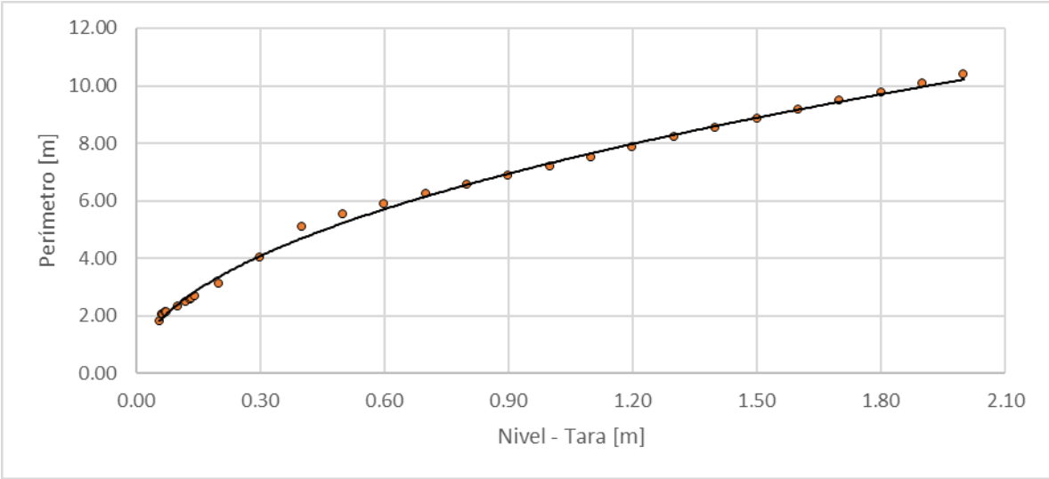
Figura 21. Nivel vs perímetro, Quebrada el Guamo - CDI San Sebastián
