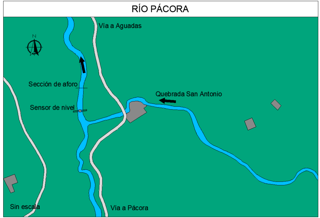
Figura 148. vista en planta, Río Pácora
