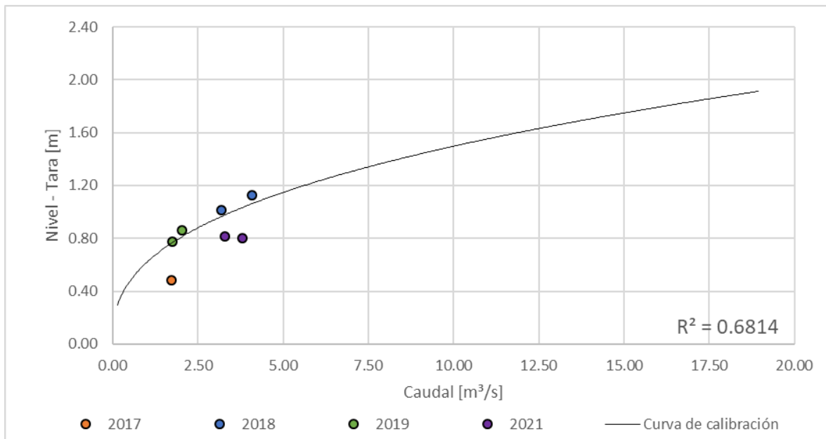
Figura 120. Curva nivel vs caudal, Río Chinchiná - Bosque Popular
