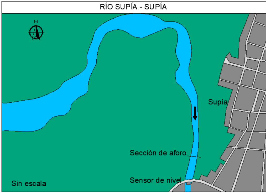
Figura 188. Vista en planta, Río Supía - Supía
