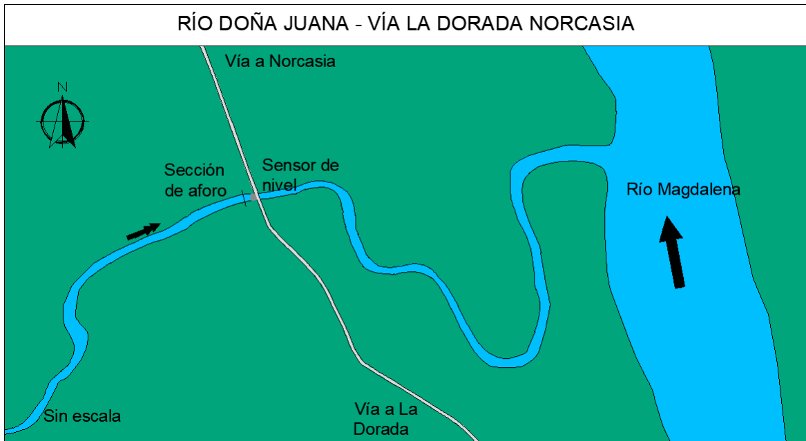
Figura 133. Vista en planta, Río Doña Juana - Vía La Dorada Norcasia
