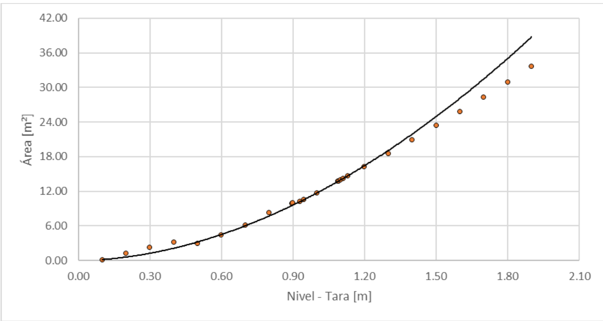
Figura 132. Nivel vs área, Río Chinchiná - El Bosque
