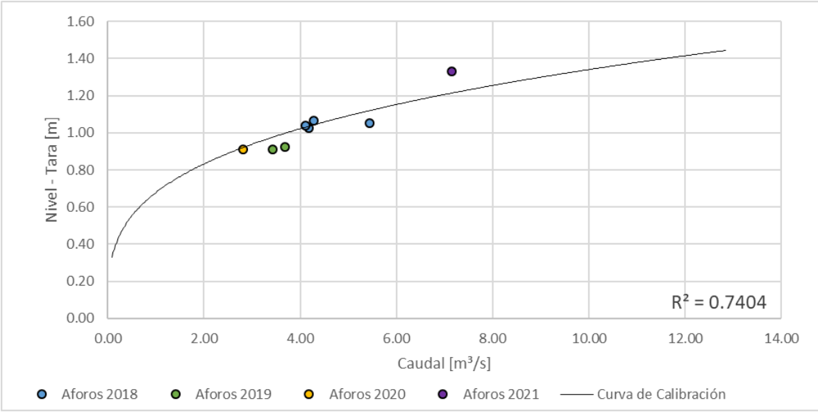
Figura 165. Curva nivel vs caudal, Río Rioclaro - La Batea
