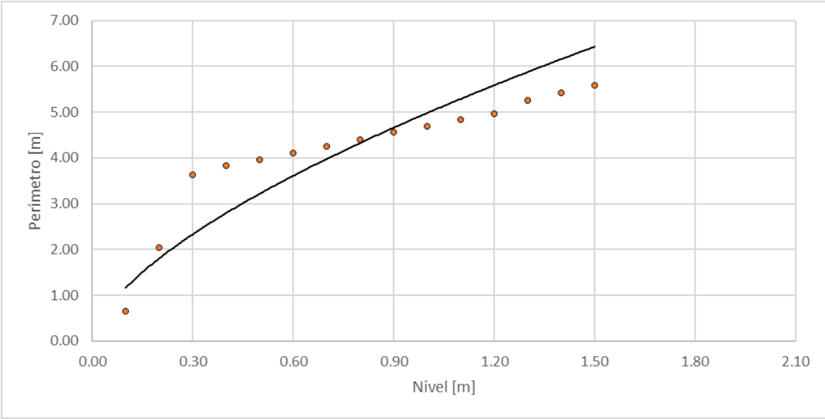
Figura 36. Nivel vs perímetro, Quebrada el Rosario – Autopistas
