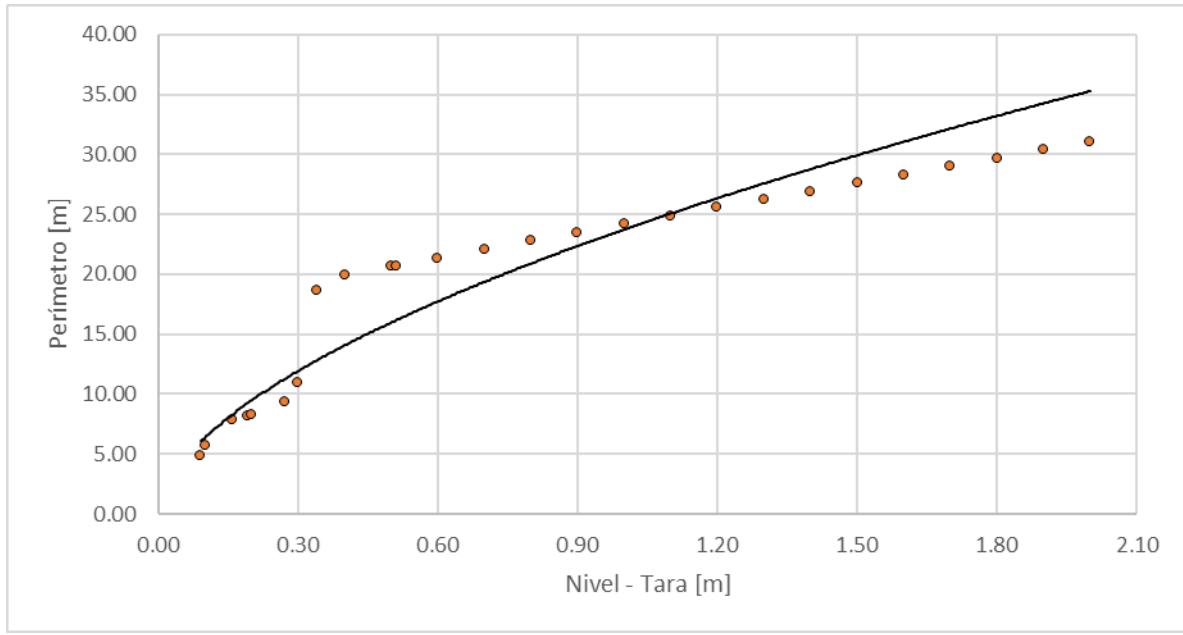
Figura 181. Nivel vs perímetro, Río Santo Domingo - Manzanares
