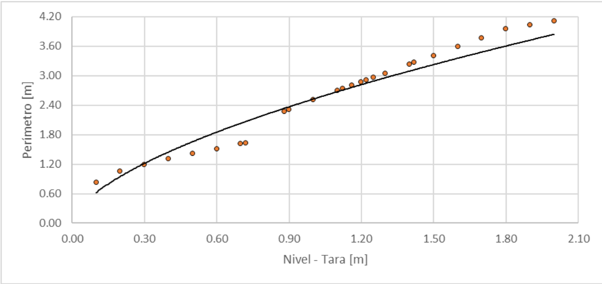
Figura 16. Nivel vs perímetro, Quebrada El Bohío – Vereda El Águila
