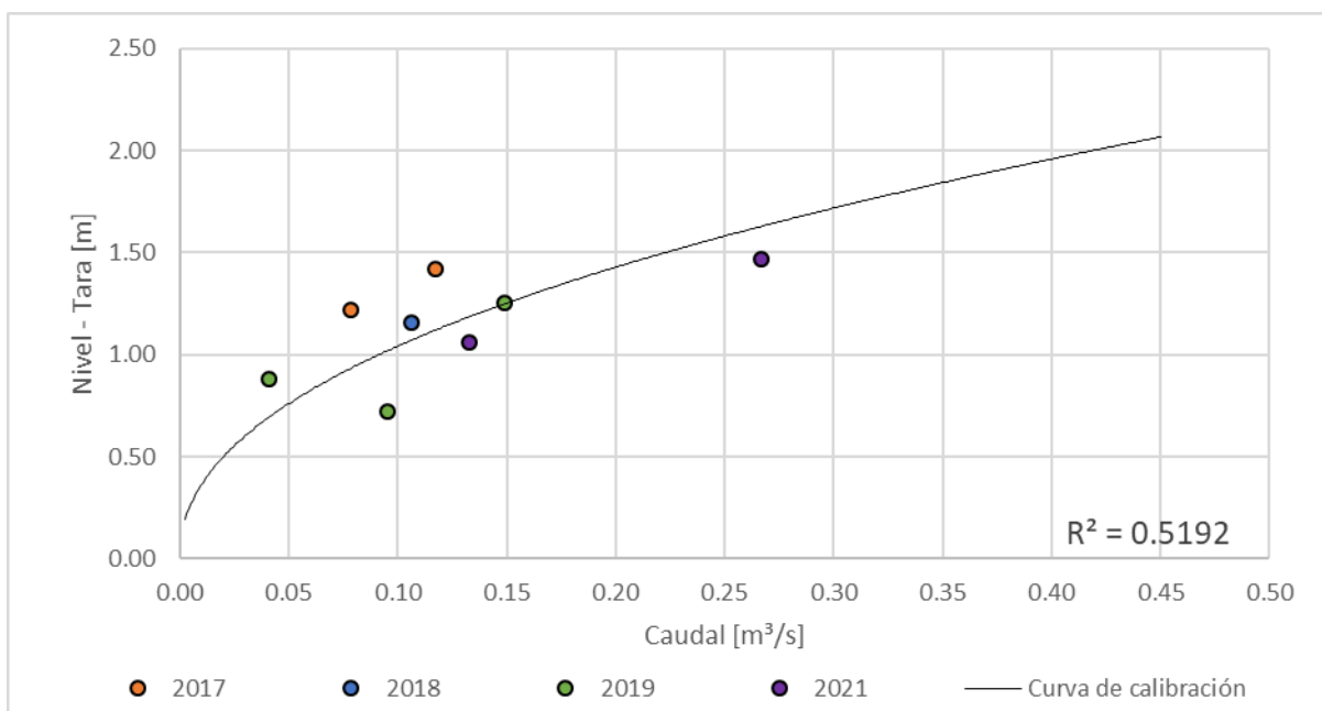
Figura 15. Curva nivel vs caudal, Quebrada El Bohío – Vereda El Águila
