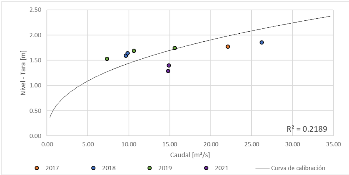
Figura 175. Curva nivel vs caudal, Río Risaralda - Camping La Palmera
