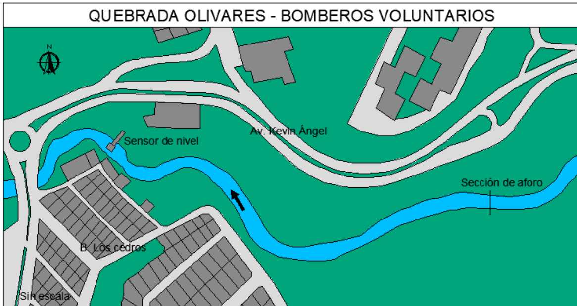
Figura 88. Vista en planta, Quebrada Olivares - Bomberos voluntarios
