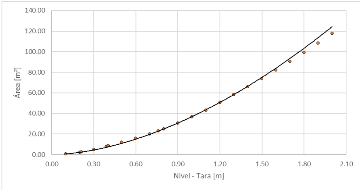
Figura 192. Nivel vs área, Río Supía – Supía
