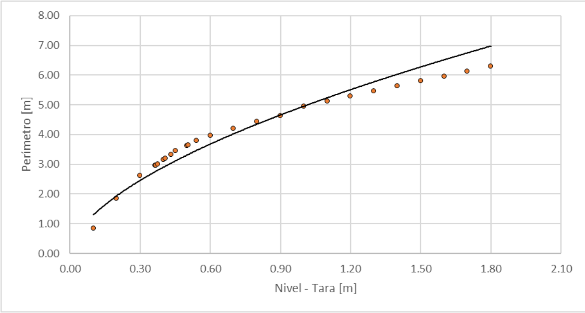
Figura 51. Nivel vs perímetro, Quebrada Guayabal - Recinto del pensamiento
