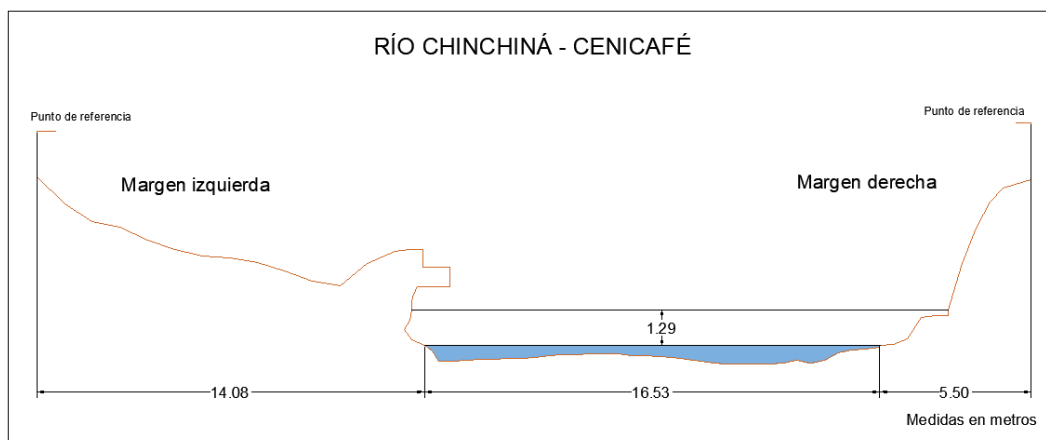
Figura 124. Sección transversal, Río Chinchiná - Cenicafé, con medidas tomadas en un cierto momento
