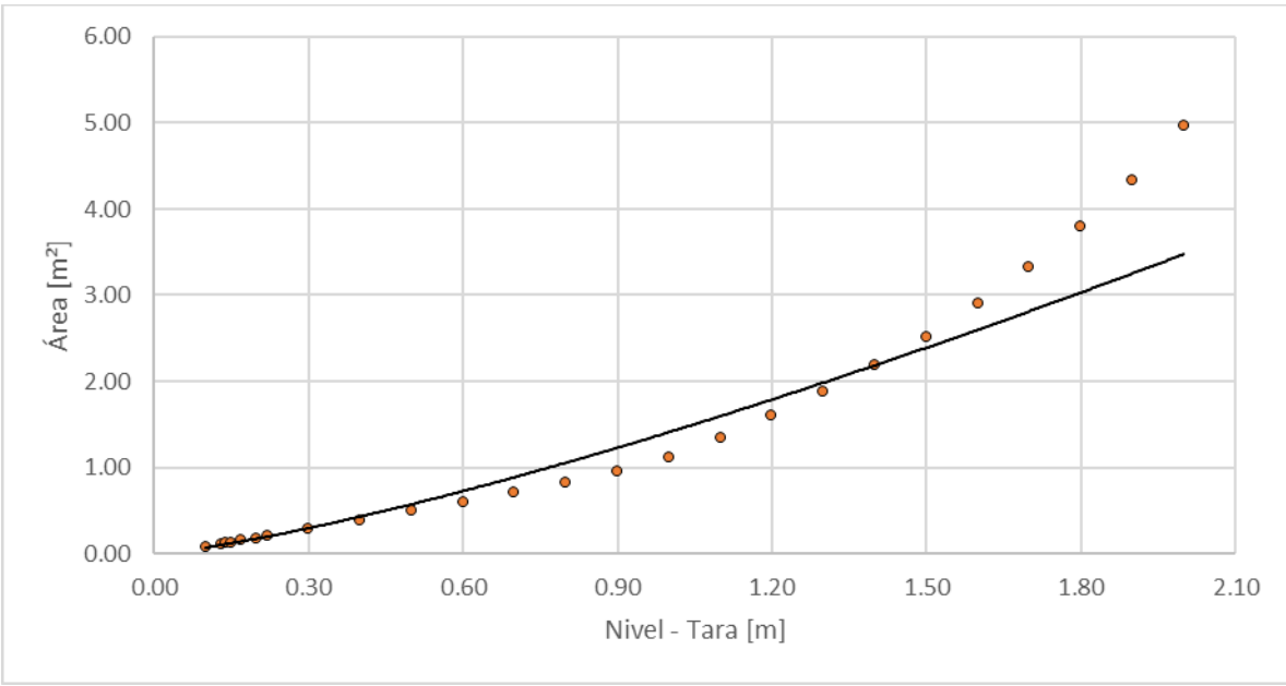
Figura 112. Nivel vs área, Quebrada Salinas - Relleno sanitario EMAS
