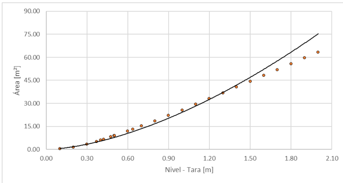
Figura 197. Nivel vs área, Río Tapias
