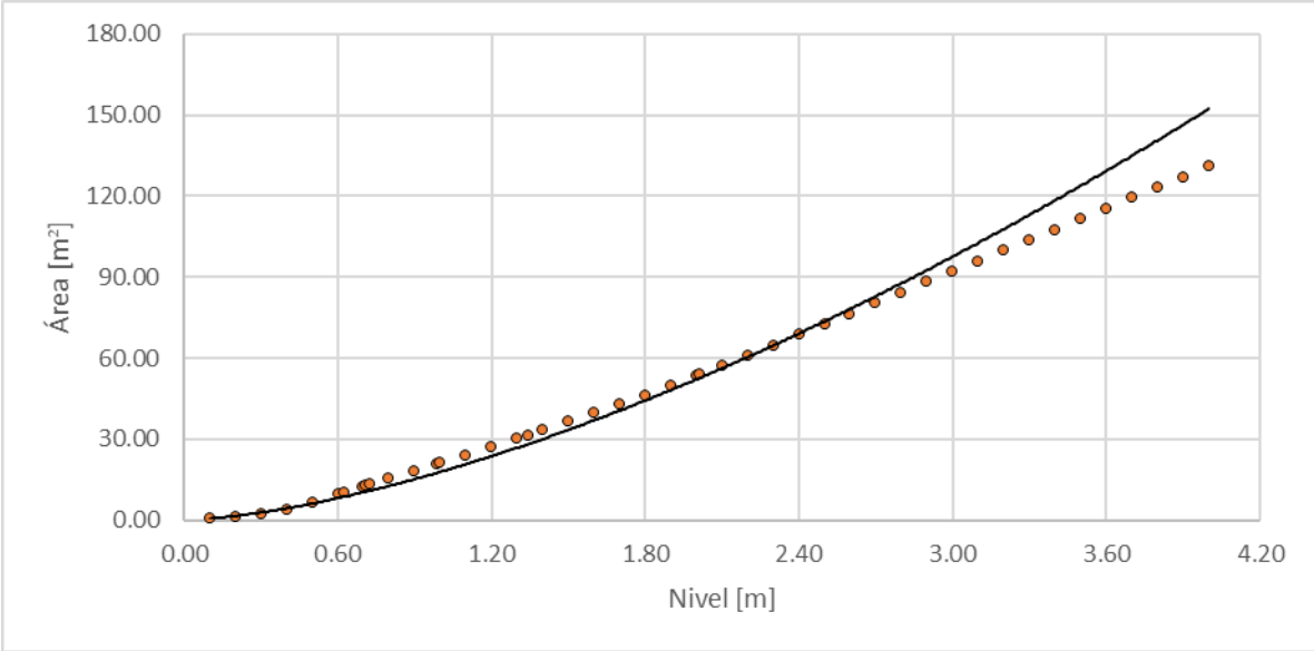
Figura 137. Nivel vs Área, Río Doña Juana - Vía La Dorada Norcasia
