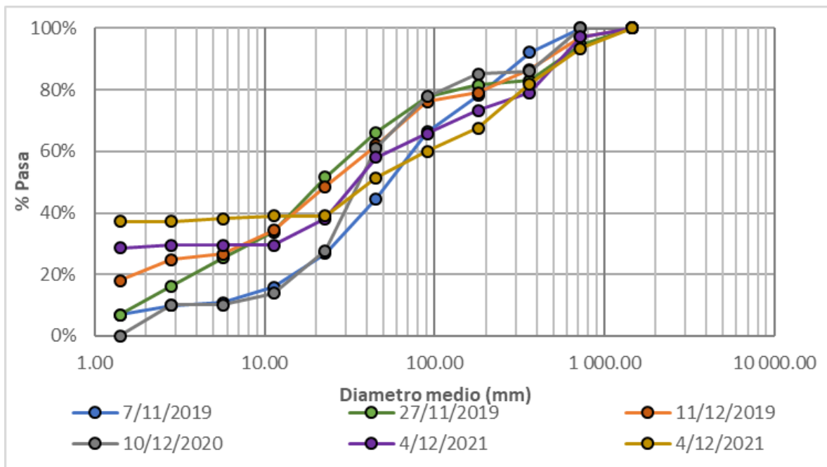
Figura 214. Granulometría material del lecho (conteo de Wolman), Río Chinchiná – El Bosque
