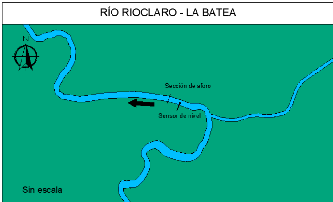
Figura 163. Vista en planta, Río Rioclaro - La Batea
