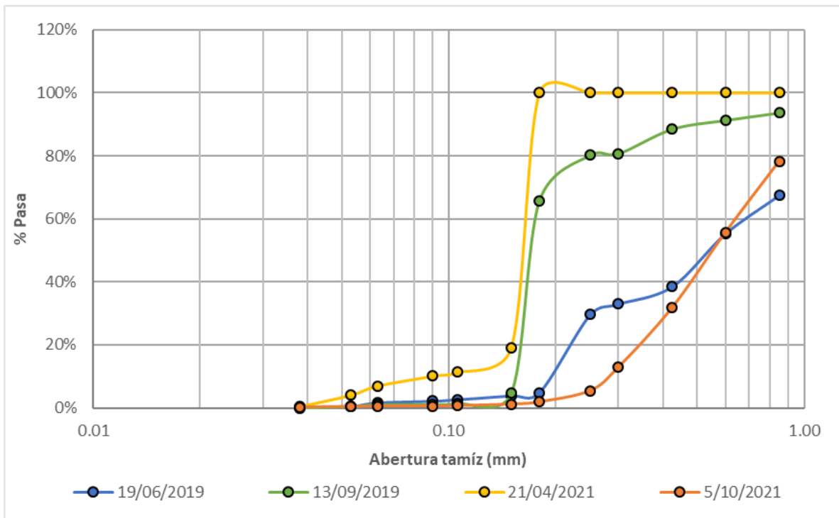
Figura 202. Granulometría sedimentos de fondo, Quebrada Olivares - Bocatoma
