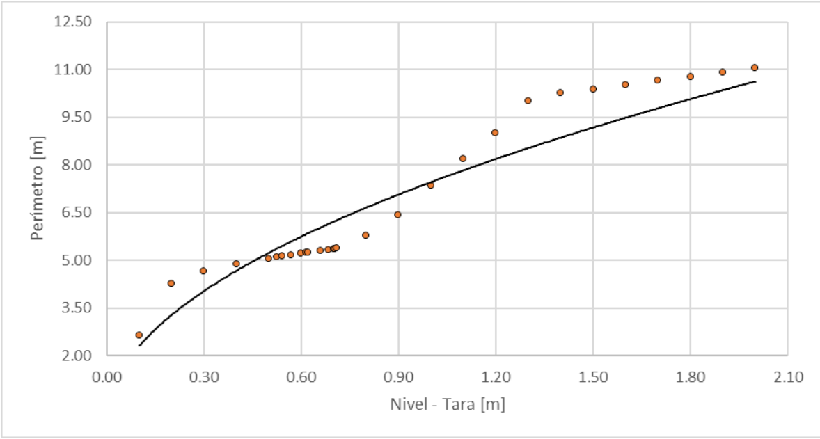
Figura 96. Nivel vs perímetro, Quebrada Olivares - El Popal
