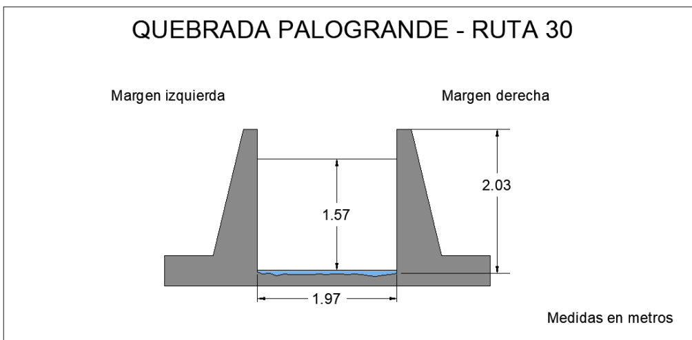
Figura 99. Sección transversal, Quebrada Palogrande – Ruta 30, con medidas hechas en un cierto momento.
