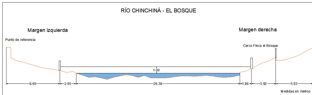
Figura 129. Sección transversal, Río Chinchiná - El Bosque, con medidas hechas en cierto momento
