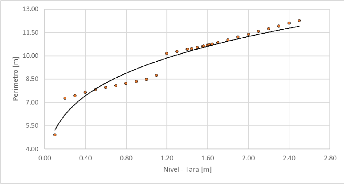
Figura 91. Nivel vs Perímetro, Quebrada Olivares - Bomberos voluntarios
