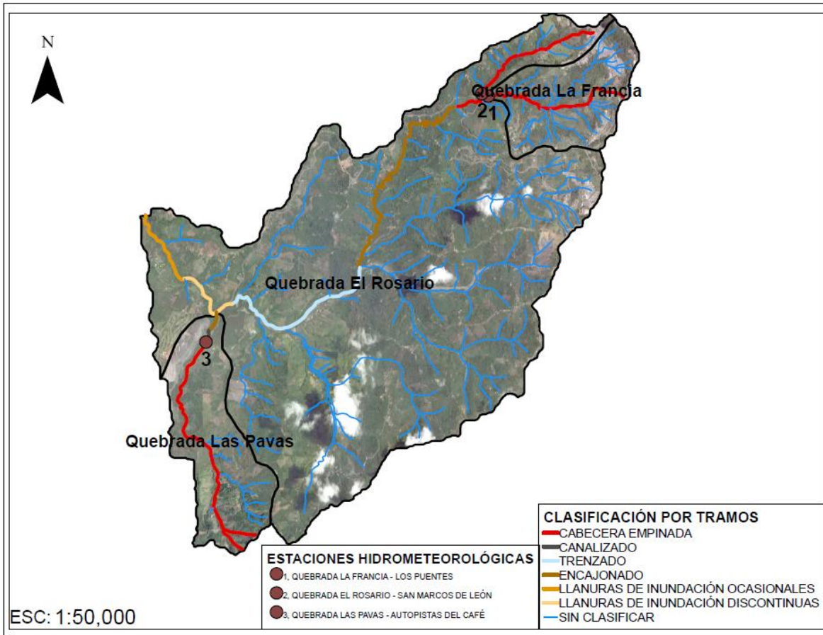
Figura 223. Clasificación cuenca de la quebrada El Rosario
