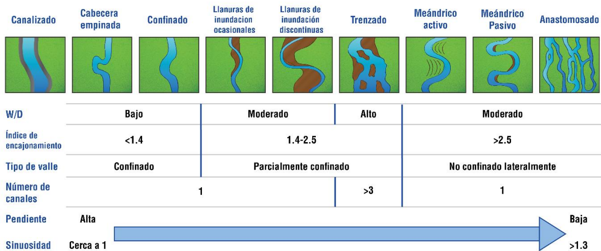
Figura 217. Clasificación de los ríos (Fryirs & Brierley, 2013), Fuente: Adaptada de Fryirs & Brierley, 2013
