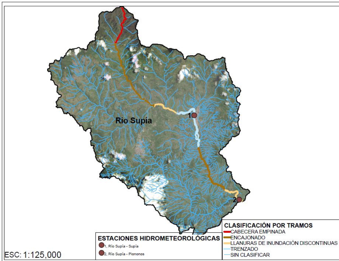
Figura 231. Clasificación cuenca del río Supía.
