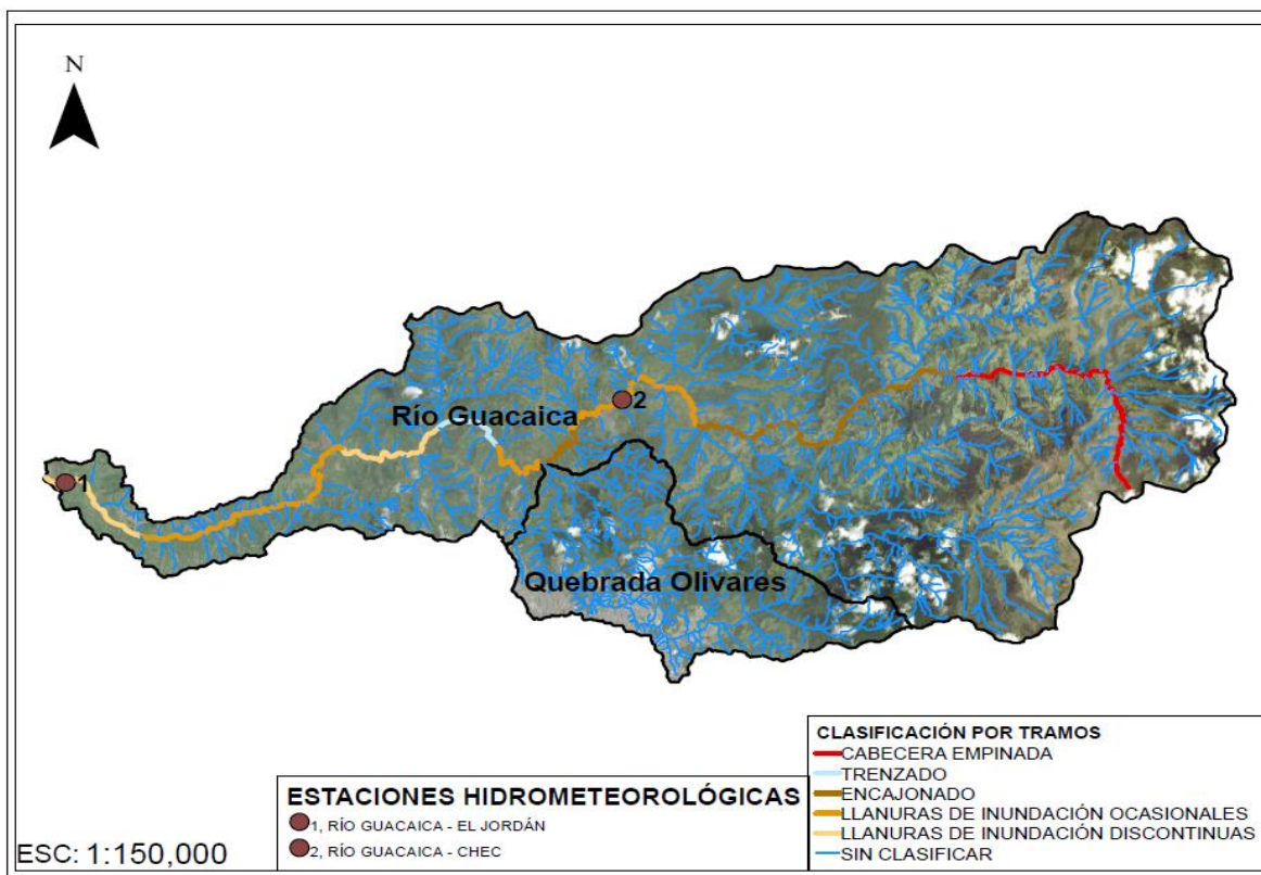
Figura 219. Clasificación cuenca del río Guacaica.
