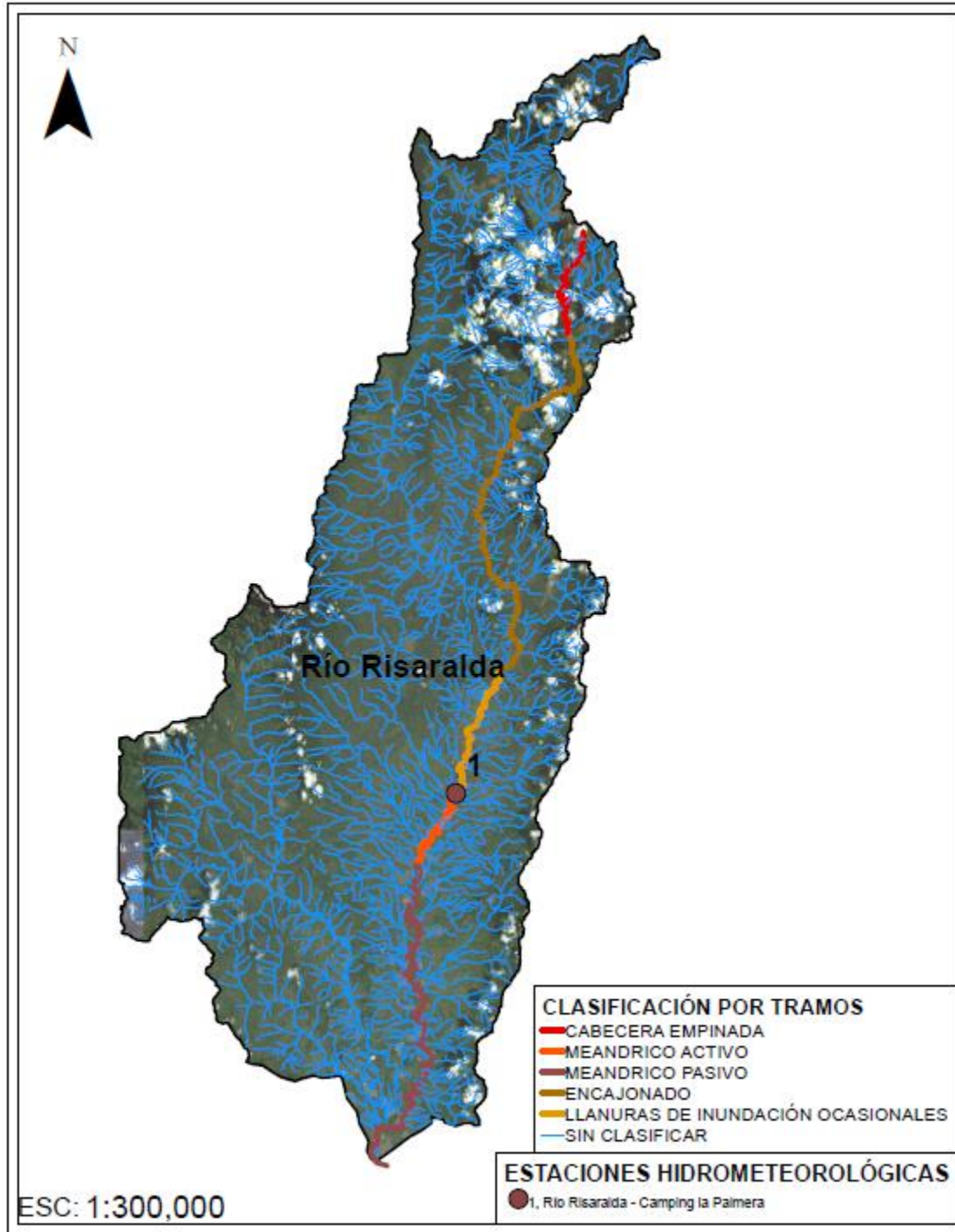
Figura 226. Clasificación cuenca del río Risaralda
