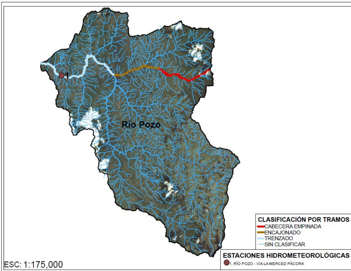
Figura 229. Clasificación cuenca del río Pozo
