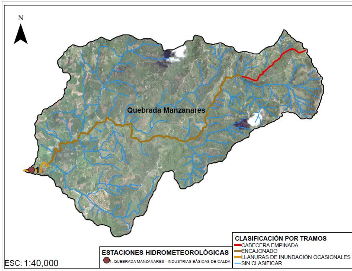
Figura 224. Clasificación cuenca de la quebrada Manzanares
