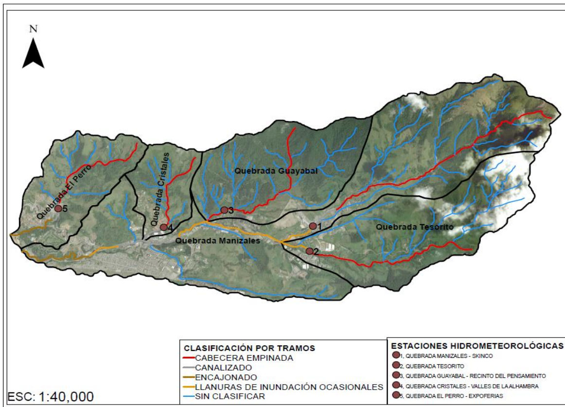
Figura 220. Clasificación cuencas de las quebradas Manizales y El Perro
