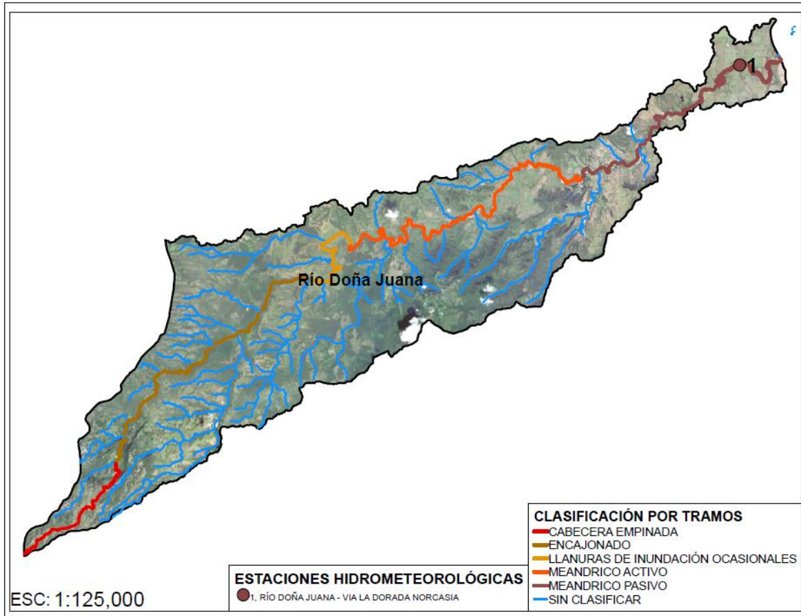
Figura 227. Clasificación cuenca del río Doña Juana
