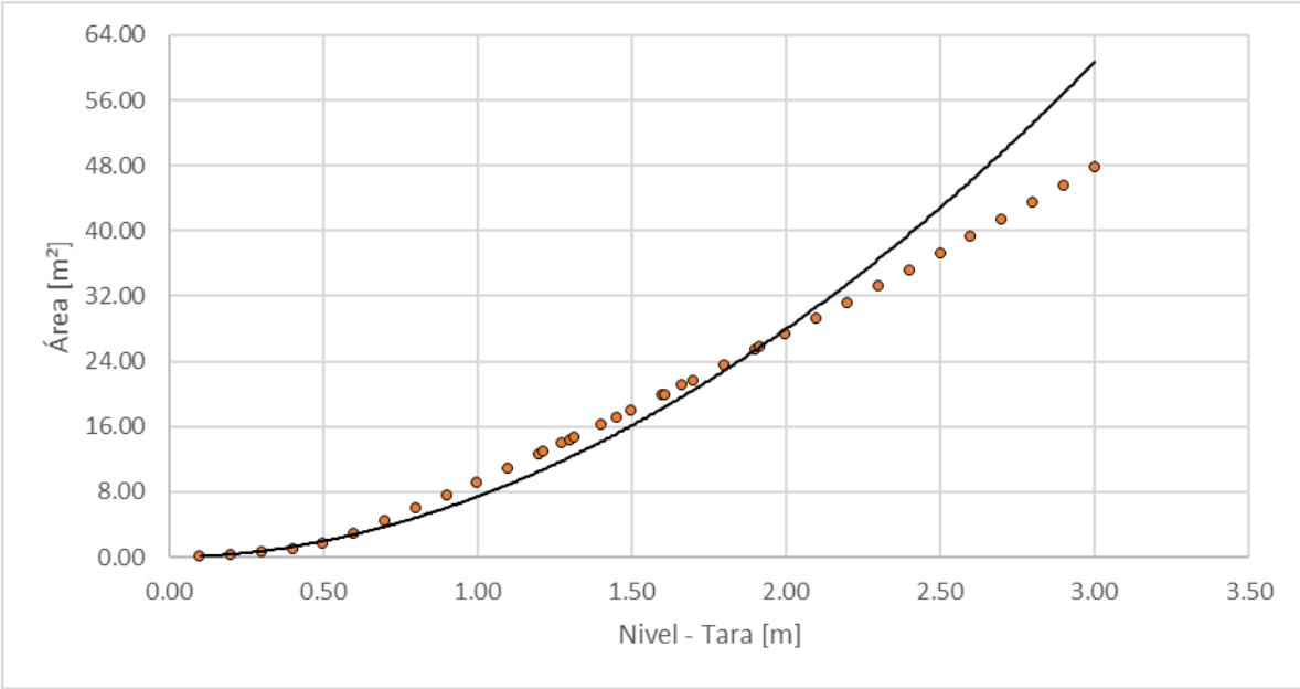
Figura 187. Nivel vs área, Río Supía - Los Piononos
