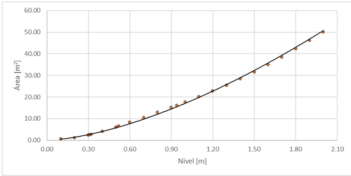
Figura 152. Nivel vs área, Río Pácora
