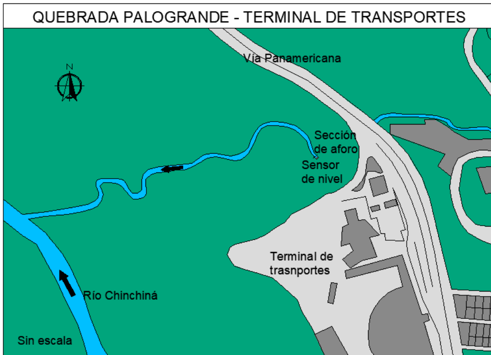
Figura 103. Vista en planta, Quebrada Palogrande - Terminal de transportes
