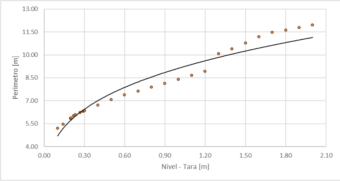
Figura 116. Nivel vs perímetro, Quebrada Tesorito – Vía al Magdalena
