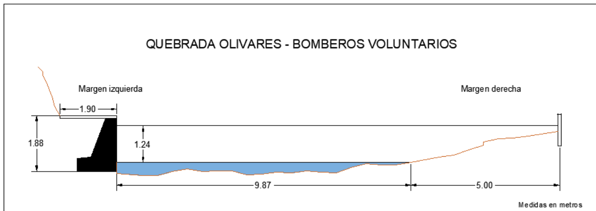
Figura 89. Sección transversal, Quebrada Olivares - Bomberos voluntarios, con medidas hechas en un cierto momento
