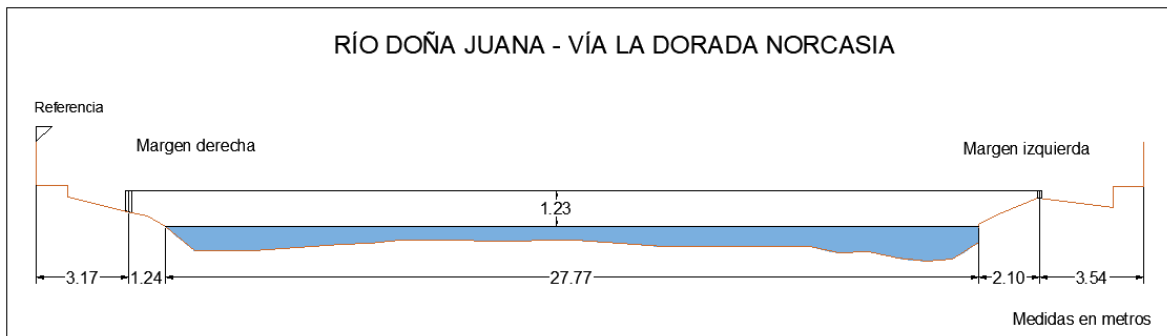
Figura 134. Sección transversal, Río Doña Juana - Vía La Dorada Norcasia, con medidas hechas en un cierto momento
