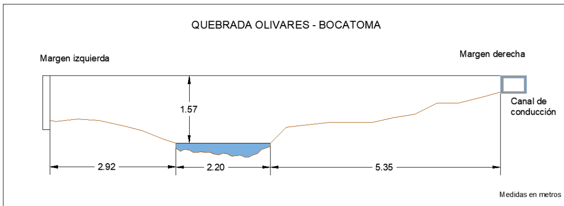
Figura 84. Sección transversal, Quebrada Olivares – Bocatoma, con medidas hechas en un cierto momento
