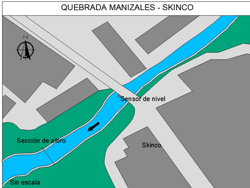
Figura 63. Vista en planta, Quebrada Manizales - Skinco
