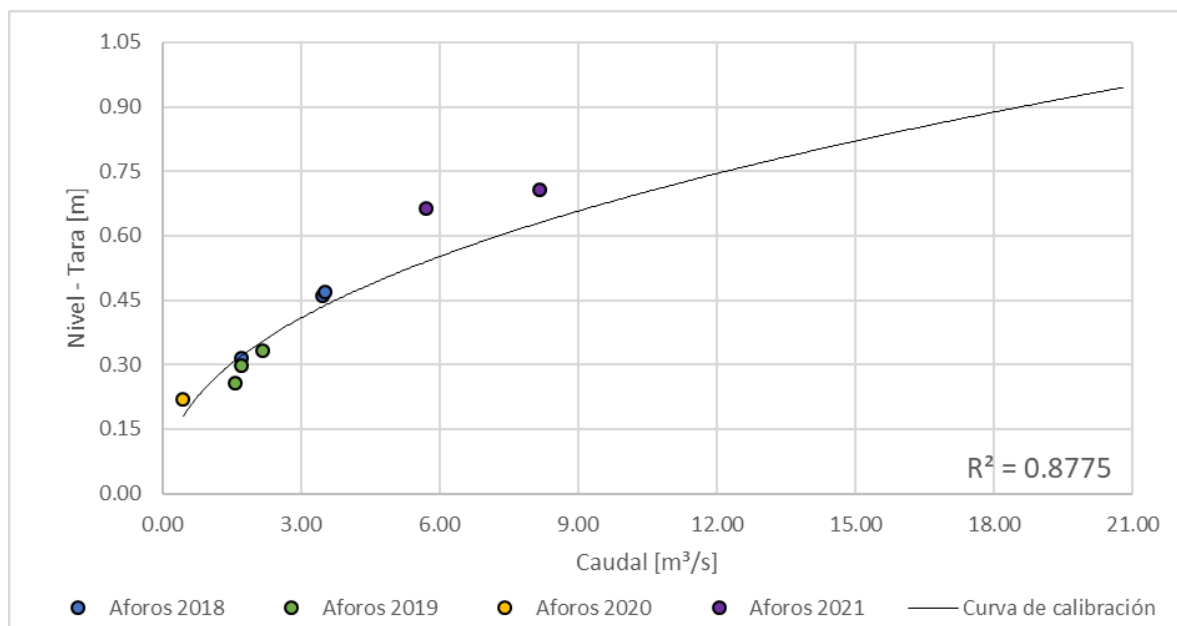
Figura 125. Curva nivel vs caudal, Río Chinchiná – Cenicafé
